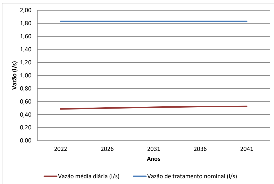
Gráfico 8.7 – Vazão Média Diária (l/s) x Capacidade nominal da ETE (l/s)
