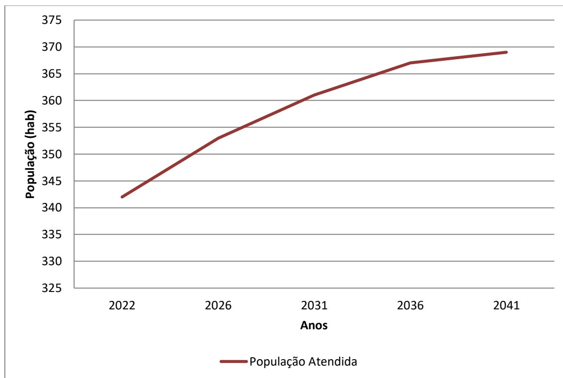
Gráfico 7.3 – População Atendida (hab.) x Anos de Planejamento – Bairro Marilândia
