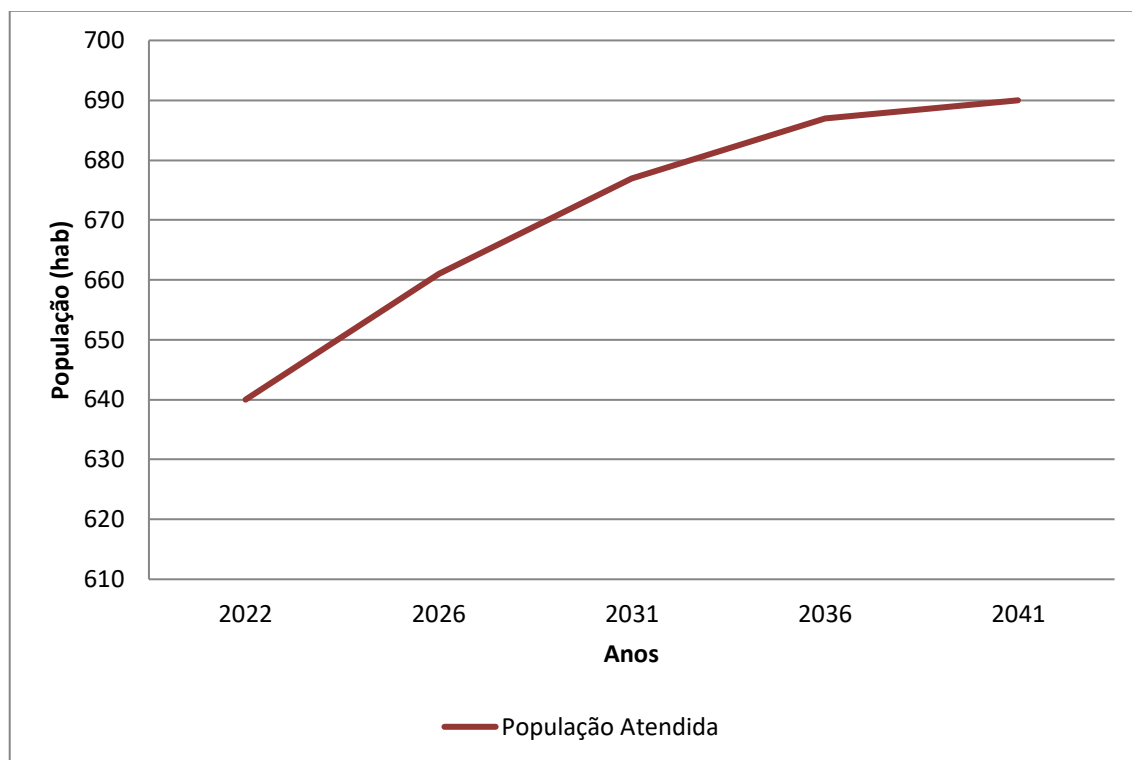
Gráfico 7.4 – População Atendida (hab.) x Anos de Planejamento – Distrito Jacuba
