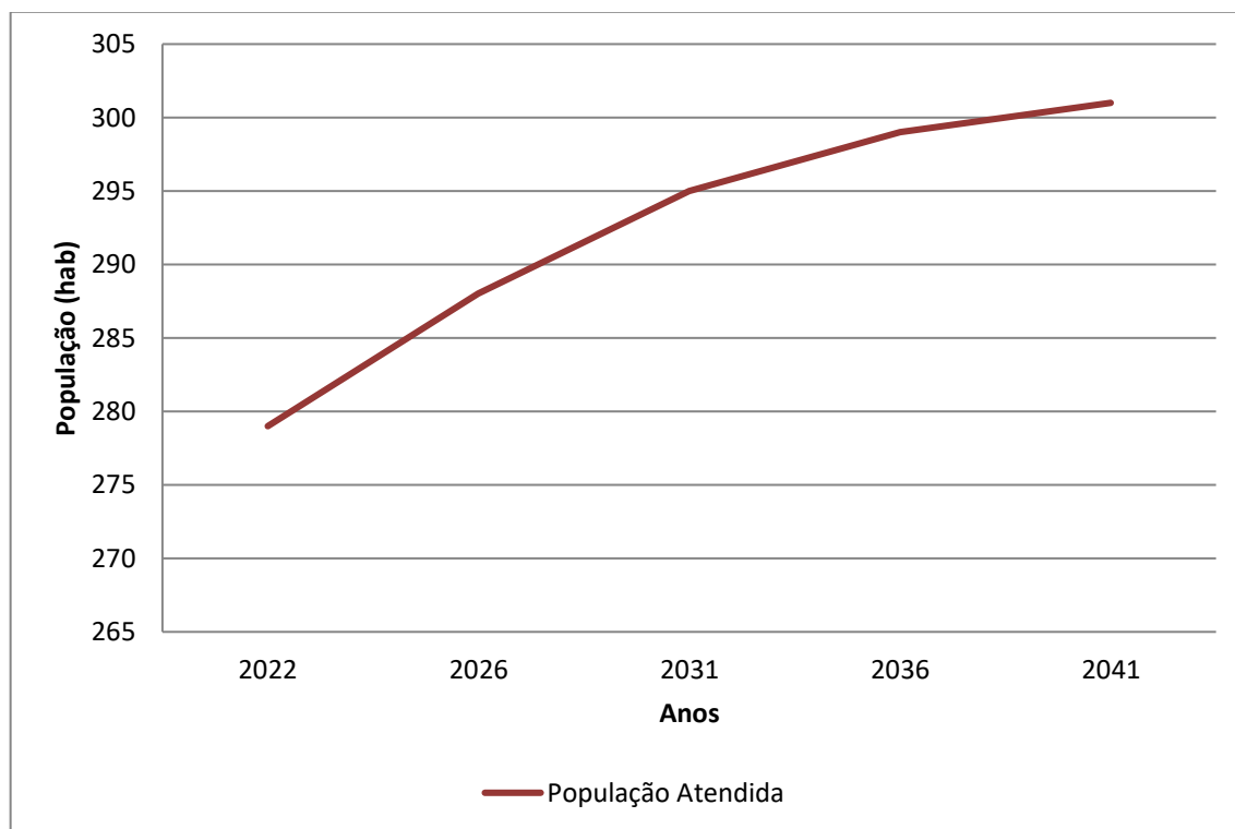
Gráfico 7.5 – População Atendida (hab.) x Anos de Planejamento – Bairro Santa Isabel
