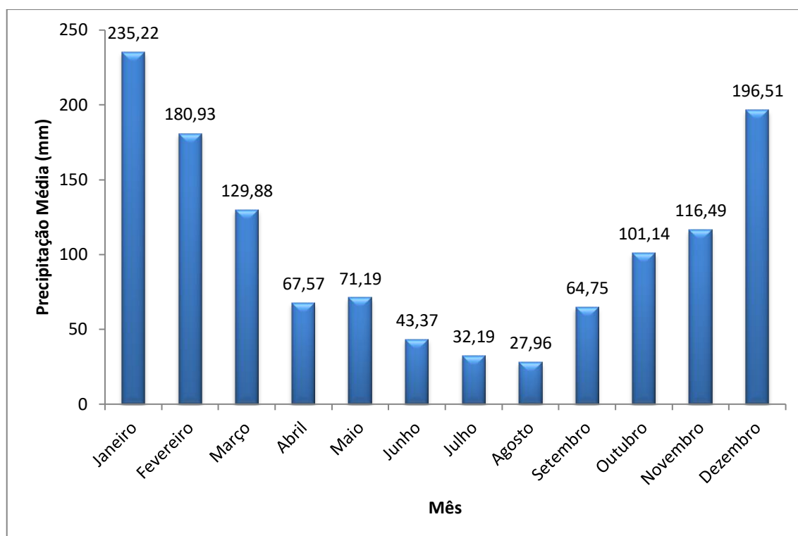
Gráfico 3.1 – Precipitação Média Mensal no Período de 1970 a 2021, Estação D6-087
