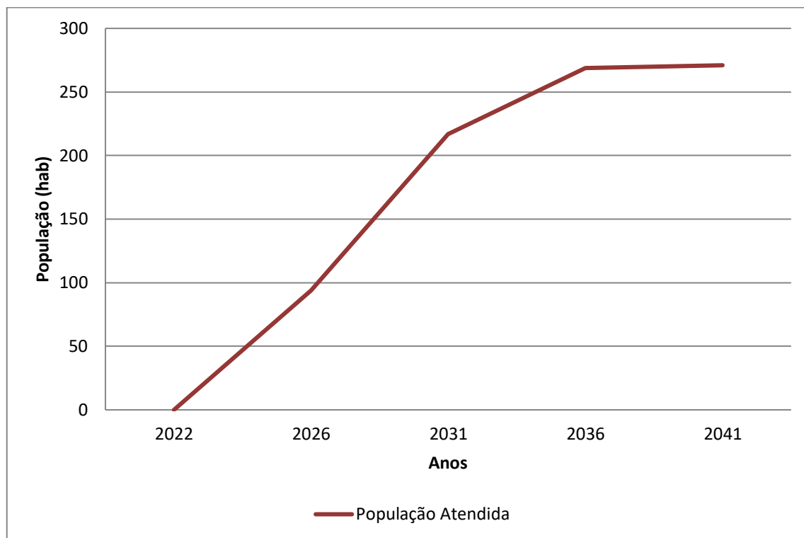
Gráfico 7.9 - População Atendida (hab.) x Anos de Planejamento – Bairro Santa Isabel
