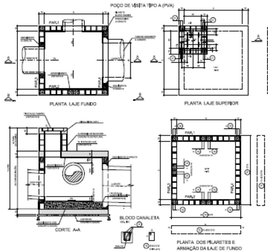
Ilustração 8.3 – Poços de visita.
