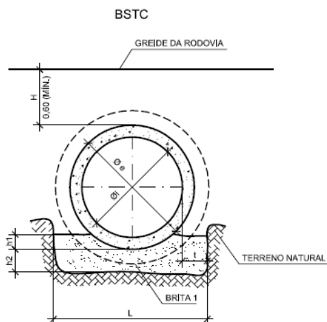
Ilustração 8.4 – Tubos de concreto.
