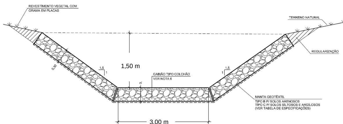
Ilustração 8.8 – Canal em gabião.
