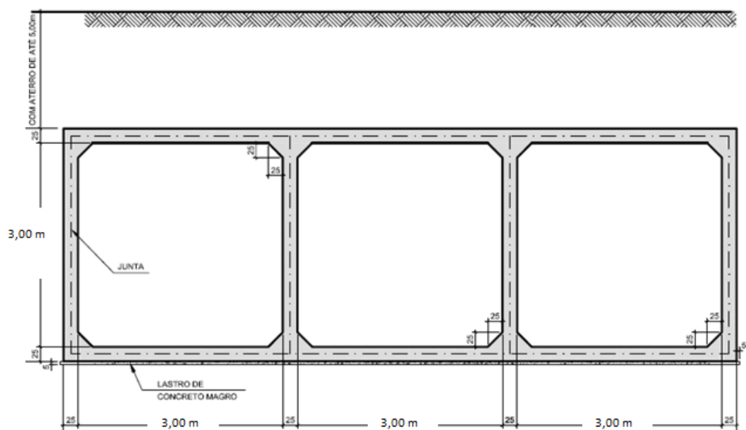
Ilustração 8.10 – BTCC 3,00 m x 3,00 m.
