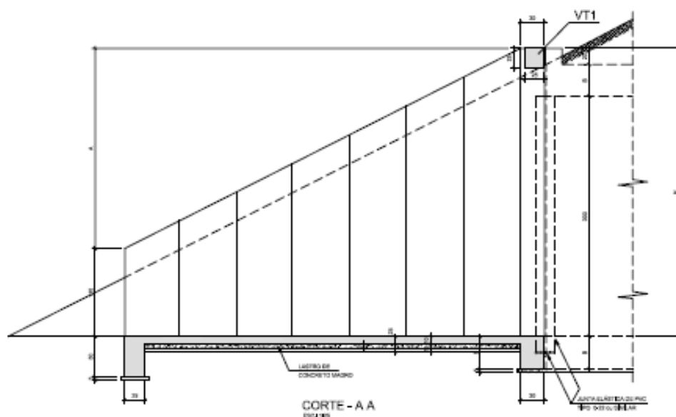
Ilustração 8.11 – Boca de saída de BTCC.
