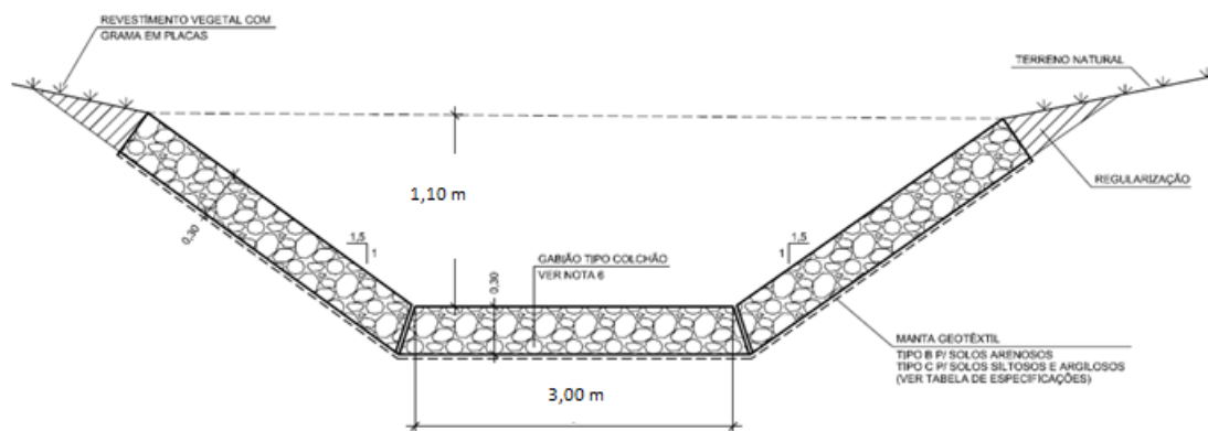
Ilustração 8.15 – Canal em Gabião.
