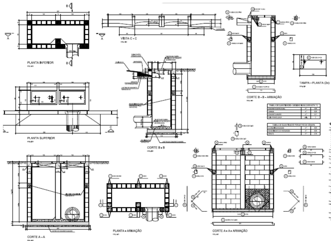
Ilustração 8.2 – Boca de lobo dupla.
