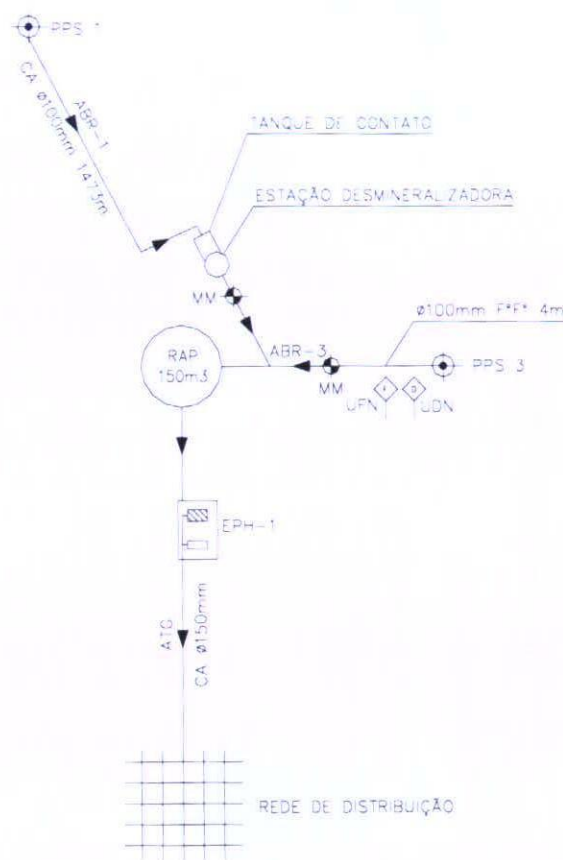
CROQUI GERAL DO SISTEMA DE ABASTECIMENTO DE ÁGUA S/ESCALA
