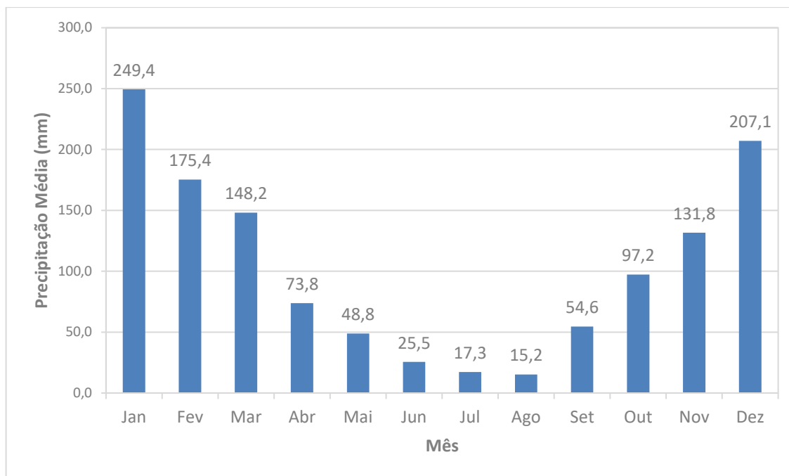
Figura 3.2 - Precipitação Média Mensal no Período de 1959 a 2020, Estação B7-013
