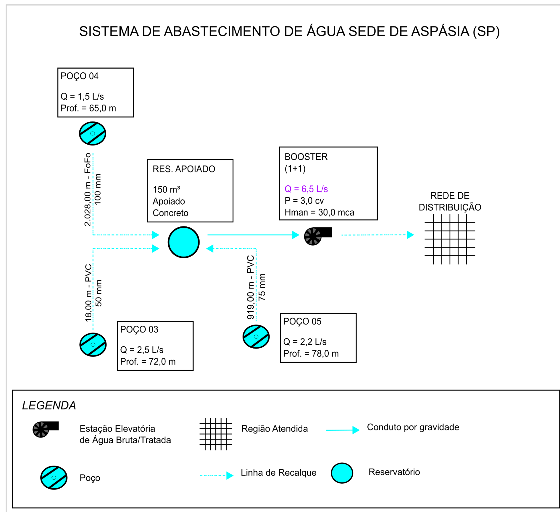
Figura 10.1 – Croqui do sistema de abastecimento de água proposto para Sede
