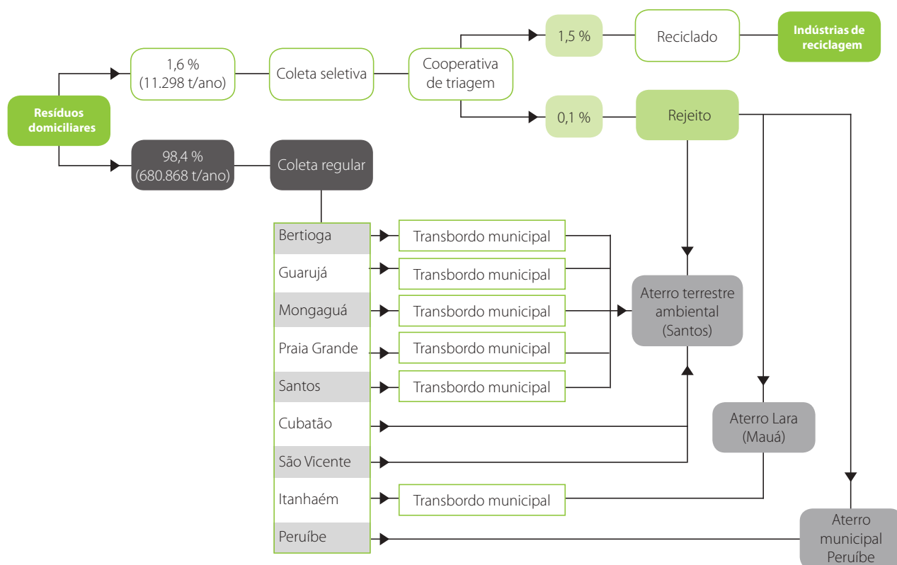
Figura 38 – Rota tecnológica do cenário atual.
