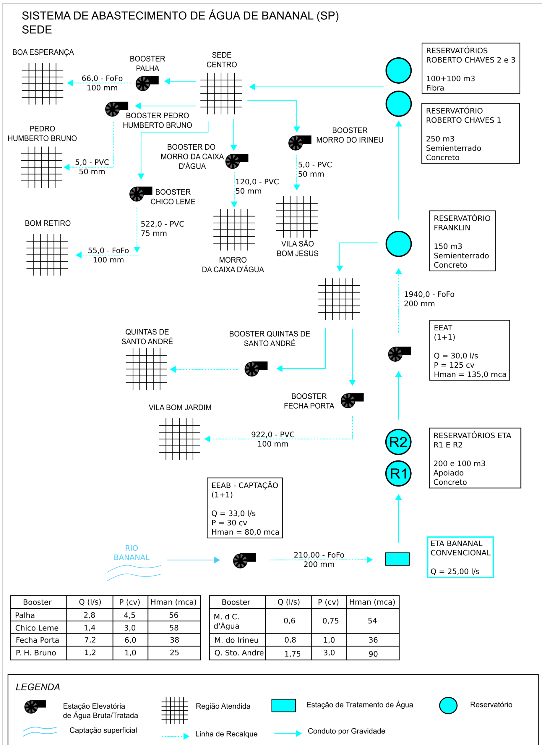
Figura 4.1 – Croqui do Sistema de Abastecimento de Água Sede Fonte: SABESP, 2020.
