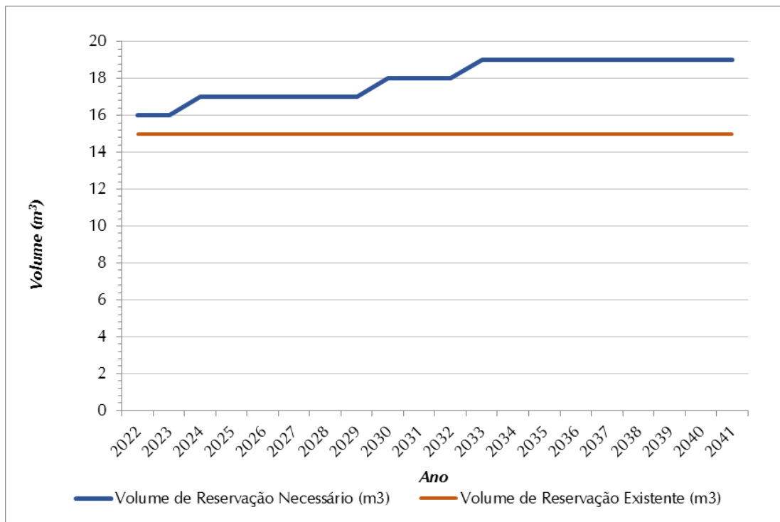
Figura 8.4 - Volume de Reservação Necessário (m³) x Volume de Reservação Atual (m³) SAA Rancho Grande
