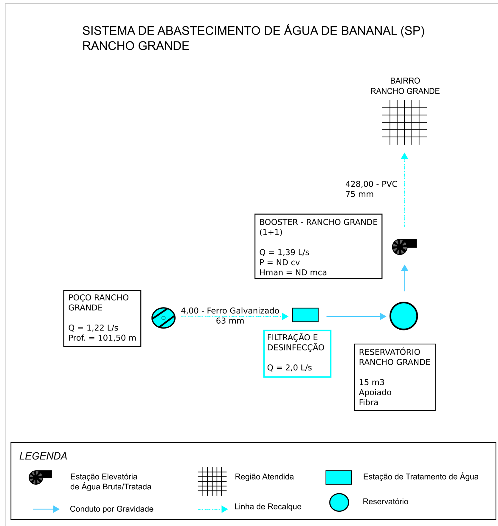
Figura 4.2 – Croqui do Sistema de Abastecimento de Água Rancho Grande
