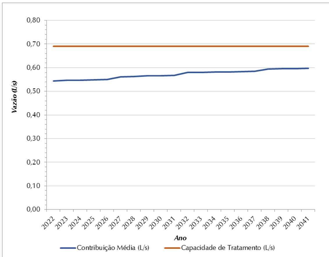
Figura 8.7 – Contribuição Média Total (L/s) x Capacidade de Tratamento de Esgoto (L/s) – SES Rancho Grande
