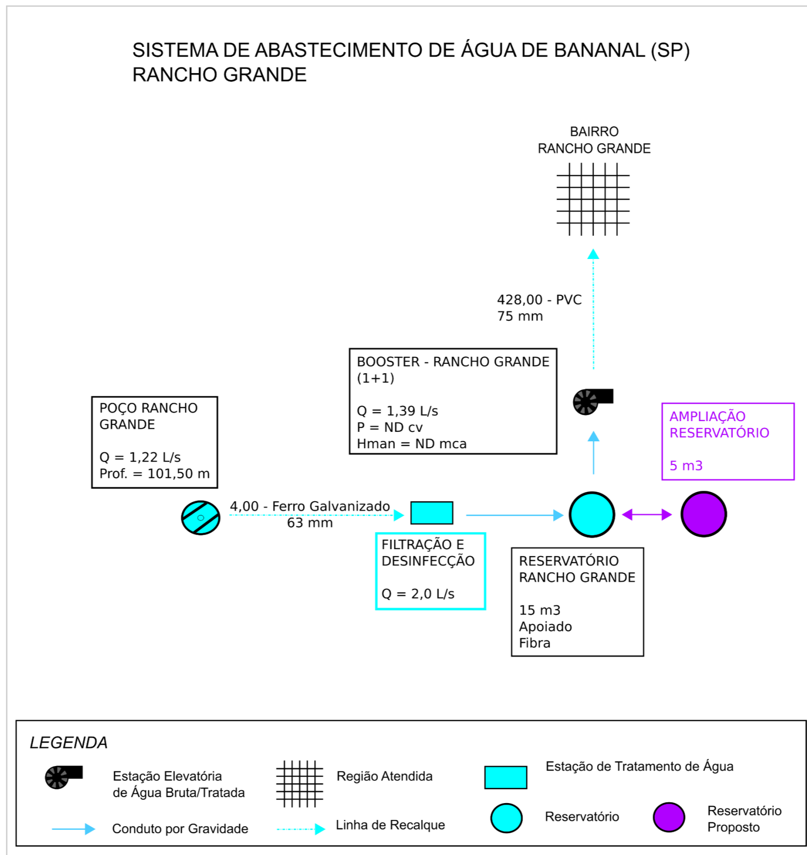
Figura 10.2 – Croqui das intervenções para o sistema de abastecimento de água Rancho Grande
