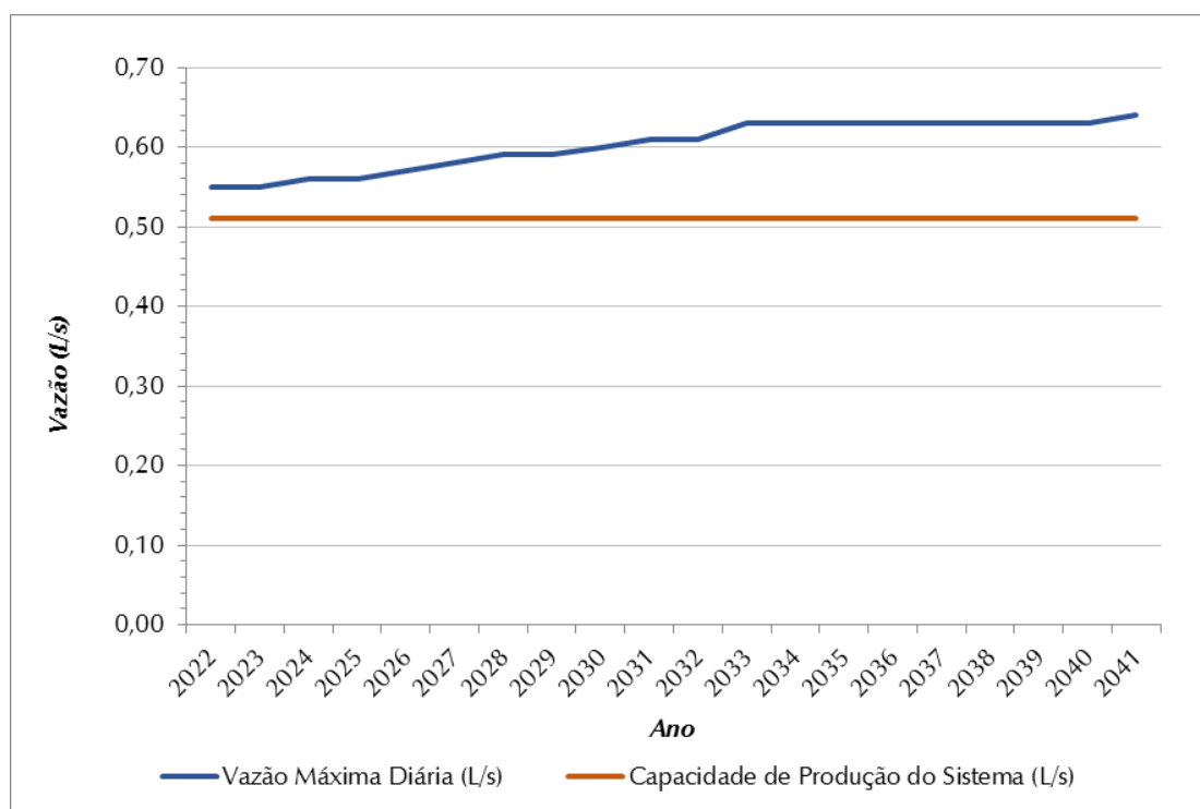
Figura 8.3 – Demandas Máximas Diárias (L/s) X Vazão Captada (L/s) – SAA Rancho Grande
