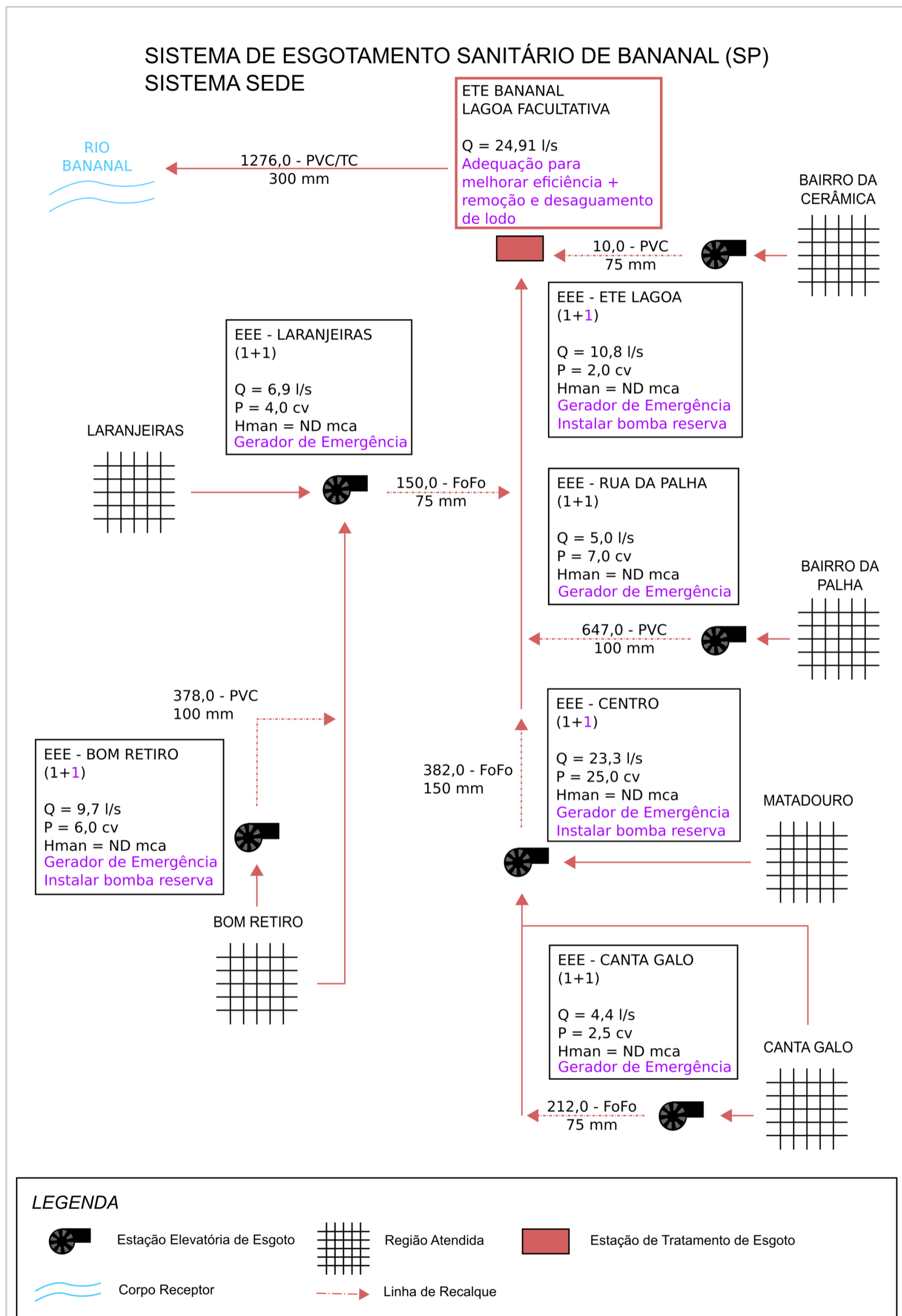
Figura 10.3 – Croqui das intervenções propostas para o sistema de esgotamento sanitário Sede
