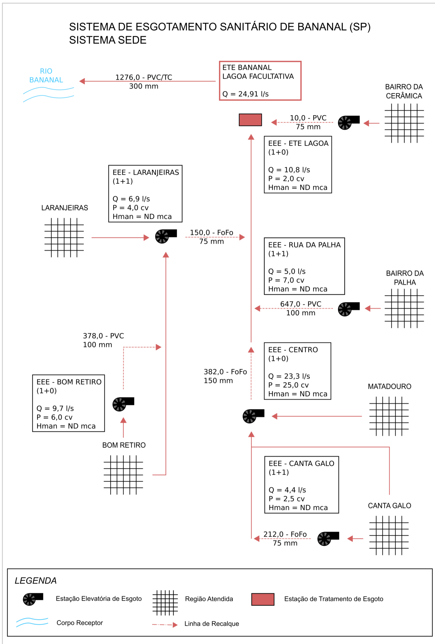
Figura 4.3 – Croqui do Sistema de Esgotamento Sanitário da Sede de Bananal Fonte: SABESP, 2020.
