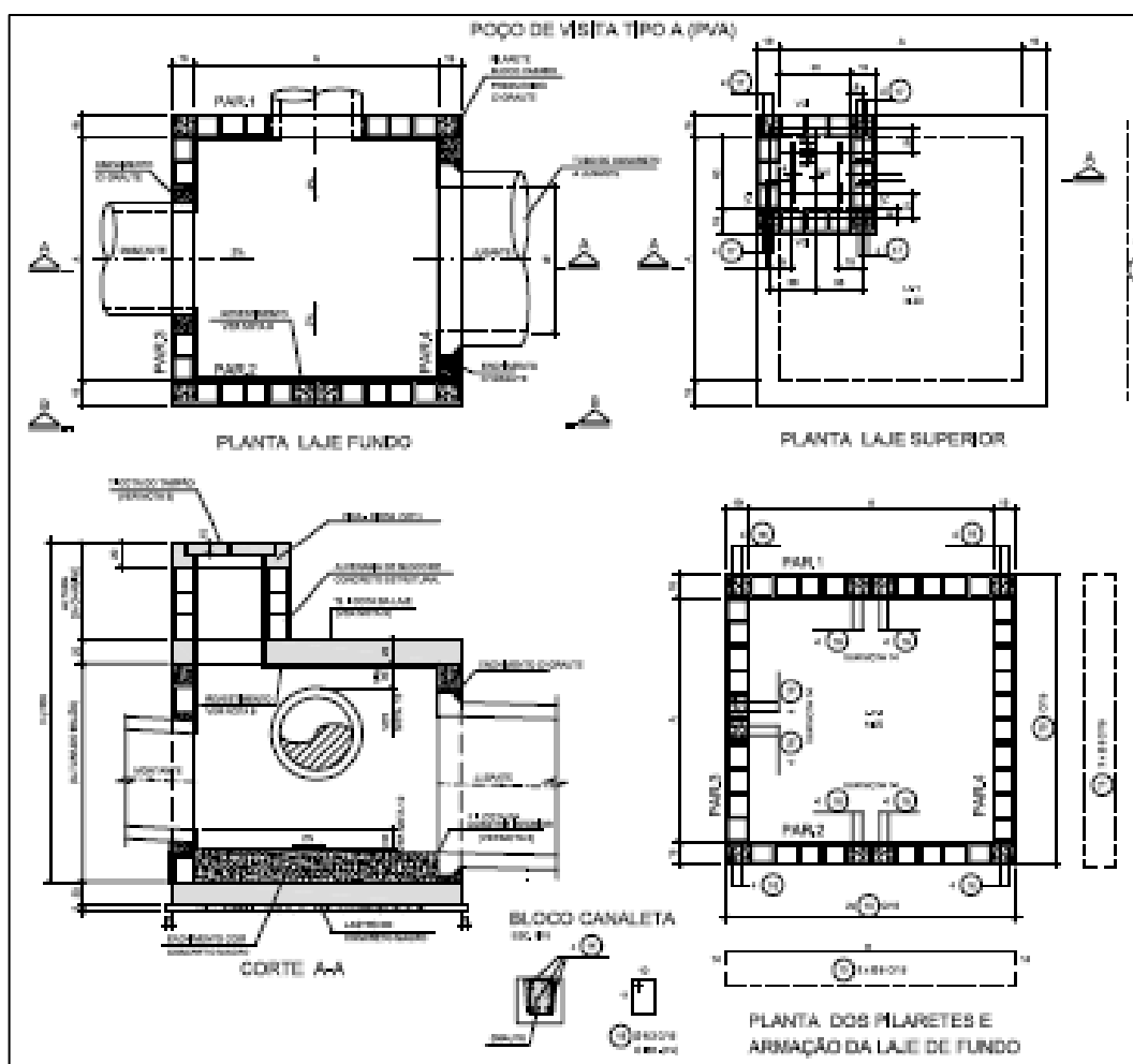
Figura 8.6 – Poço de visita
