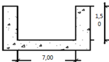
Figura 8.9 – Seção planejada para o canal de concreto
