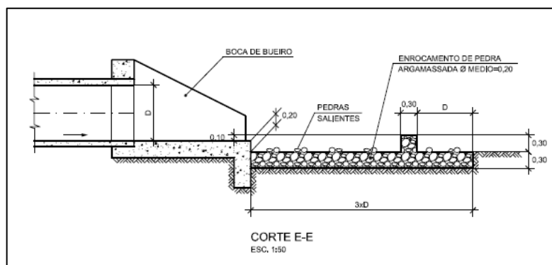
Figura 8.20 – Dissipador de energia
