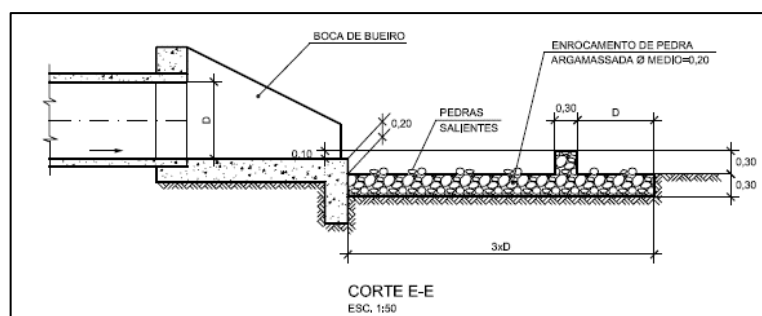
Figura 8.29 – Dissipador de energia
