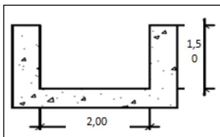
Figura 8.21 – Seção planejada para o canal de concreto
