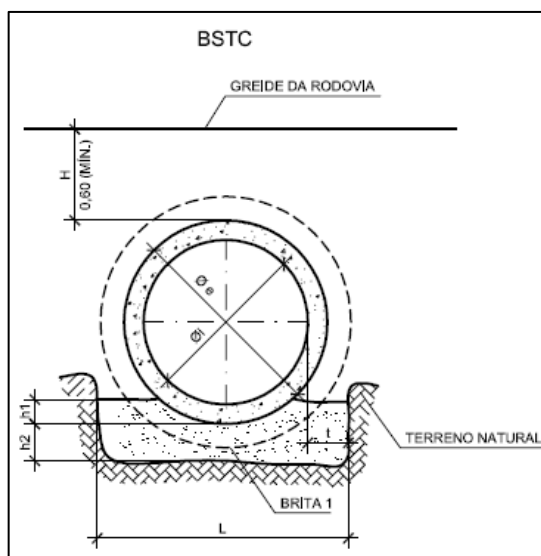
Figura 8.3 – Assentamento de tubos de concreto
