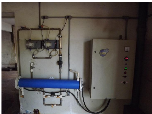
Foto 3.64 – Detalhe do gerador de cloro (hipoclorito de sódio) para desinfecção
