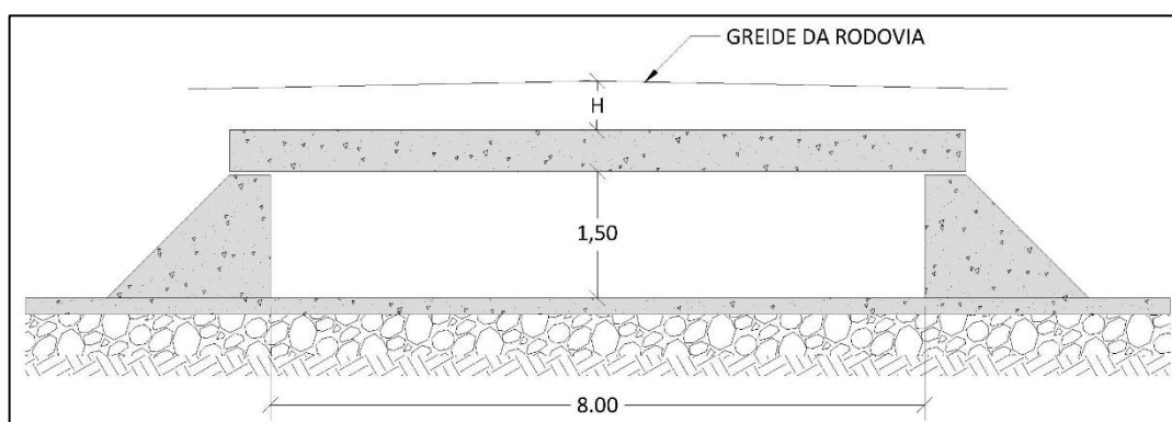
Figura 8.8 – Bueiro de placa
