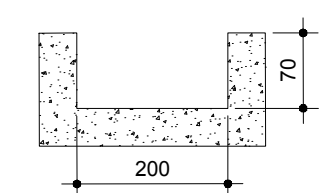
SEÇÃO PLANEJADA PARA O CANAL DE CONCRETO
