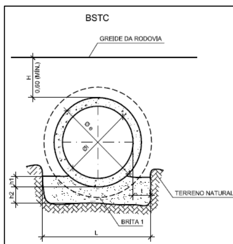
Figura 8.26 – Assentamento de tubos de concreto
