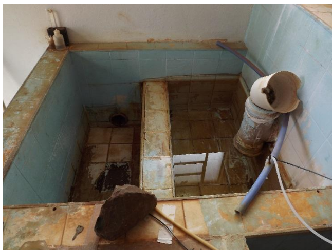
Foto 3.39 – Detalhe de tanque de contato para desinfecção do Poço Ibitu
