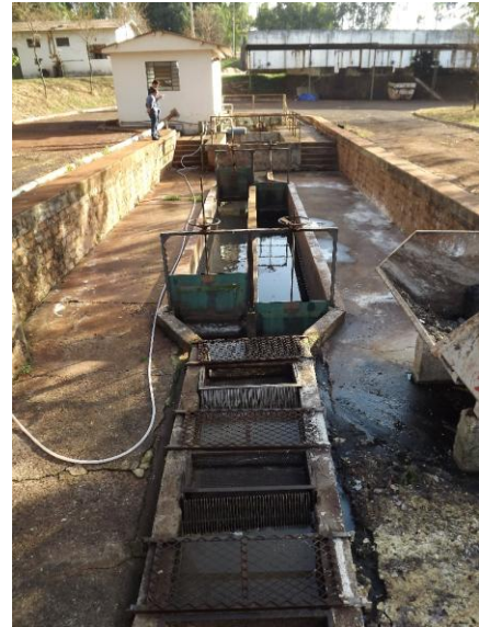
Foto 3.202 – Gradeamento e caixa de areia (ao fundo) – Tratamento Preliminar – ETE IV
