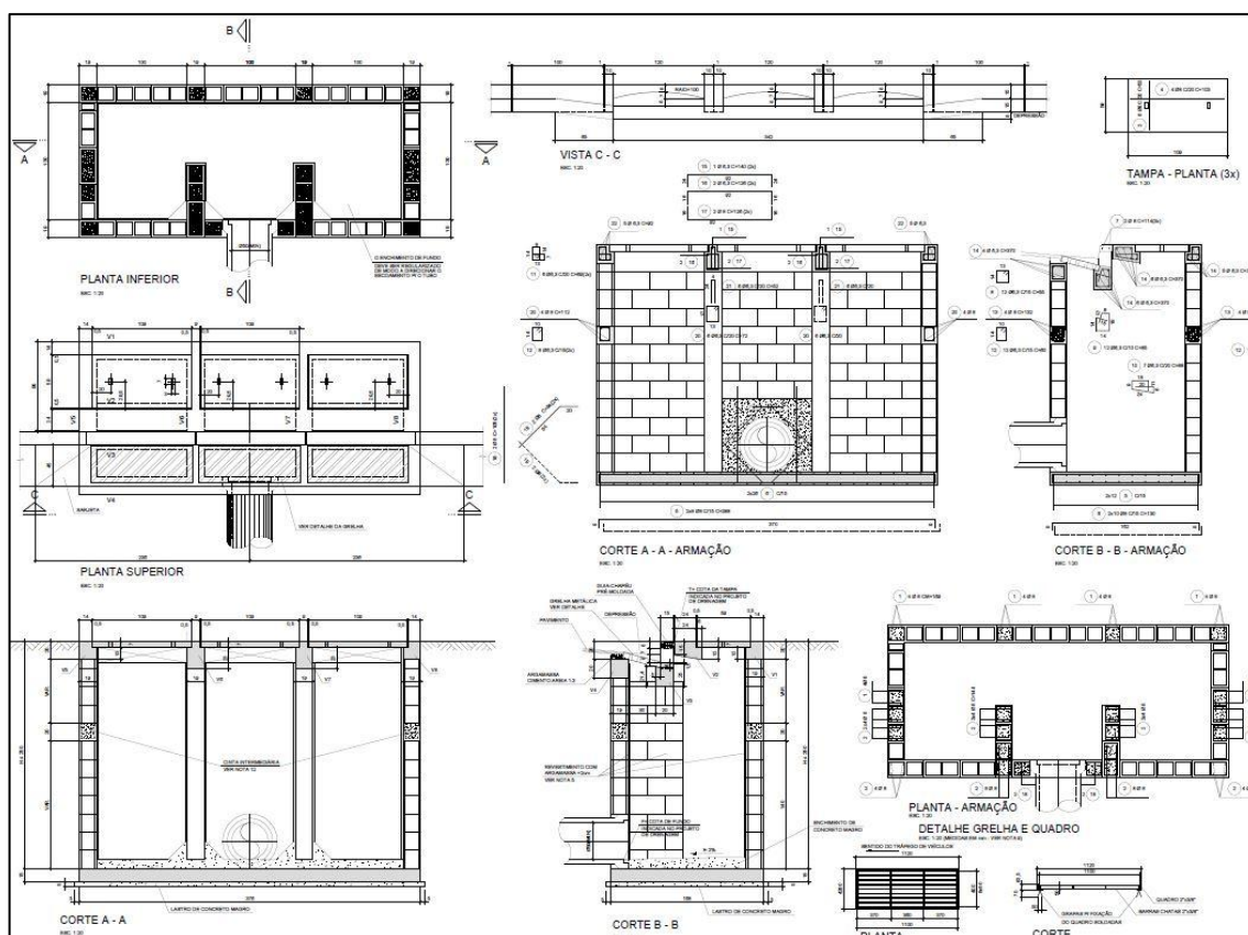
Figura 8.4 – Boca de lobo tripla - BLGT
