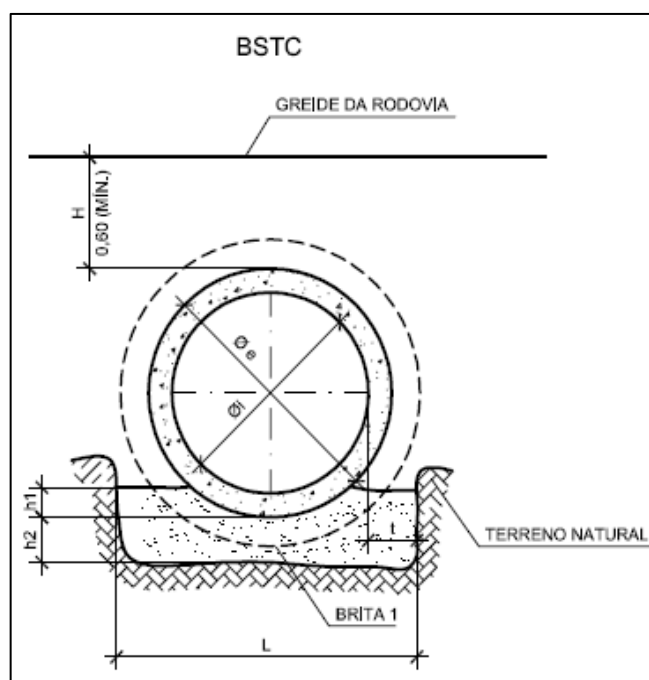
Figura 8.13 – Assentamento de tubos de concreto
