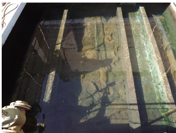
Foto 3.49 – Vista geral de um dos filtros ascendentes da ETA
