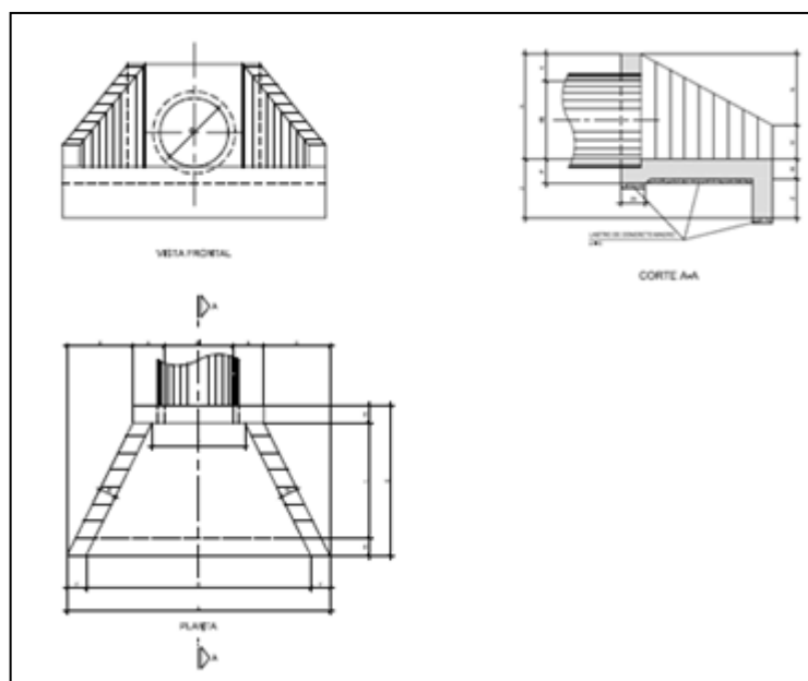
Figura 8.30 – Ala de saída de BSTC
