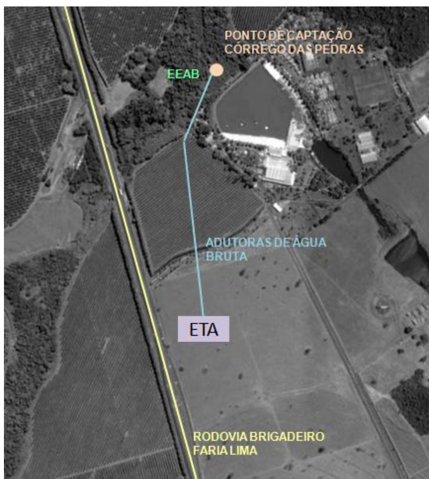
Figura 8.1 – Esquema das possíveis intervenções no sistema de captação superficial do Córrego das Pedras
