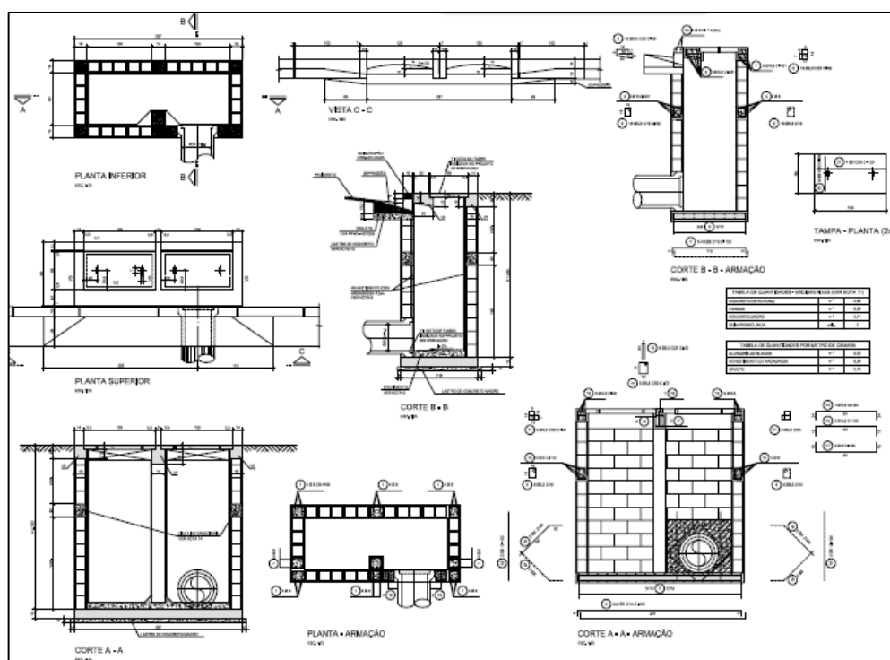
Figura 8.5 – Boco de lobo dupla
