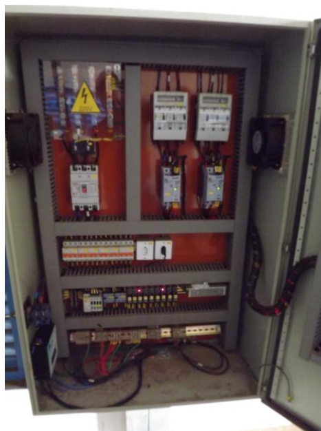
Foto 3.112 – Detalhe de painel elétrico na EEAT Vida Nova
