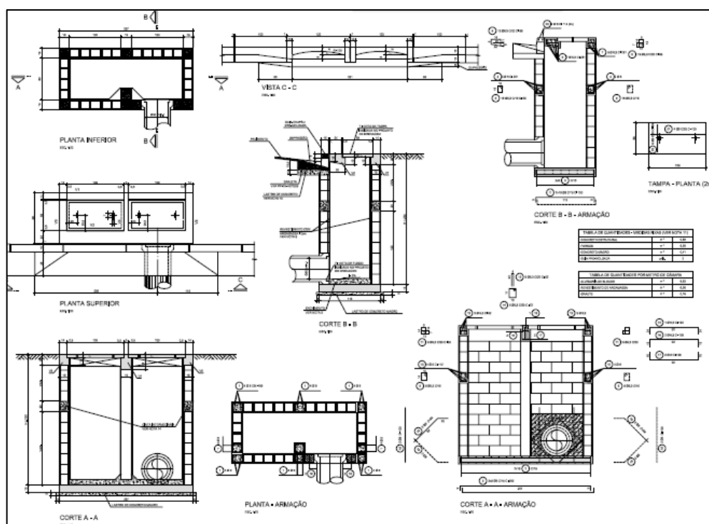
Figura 8.27 – Boca de lobo dupla
