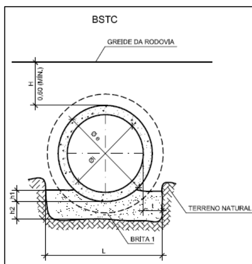
Figura 8.19 – Assentamento de tubos de concreto
