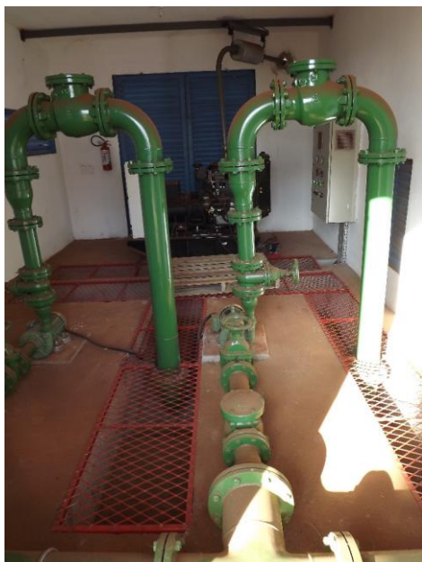
Foto 3.111 – Vista geral da EEAT I Vida Nova
