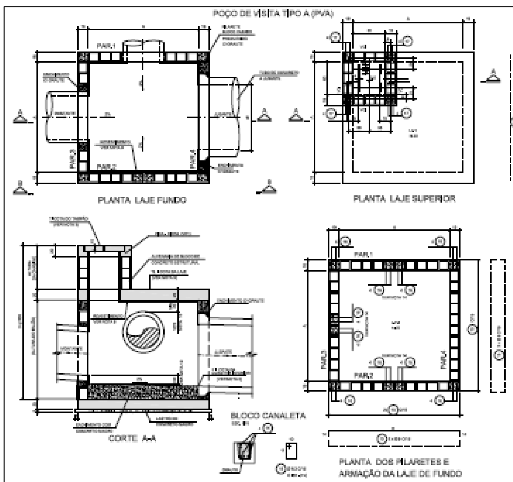
Figura 8.24 – Poço de visita
