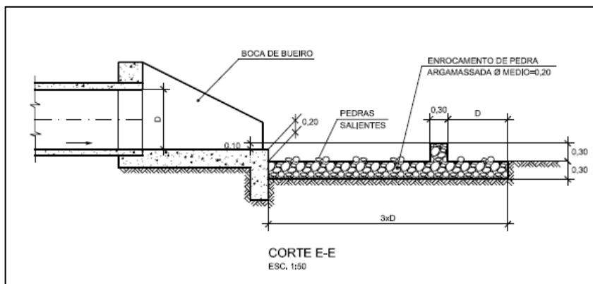
Figura 8.11 – Dissipador de energia
