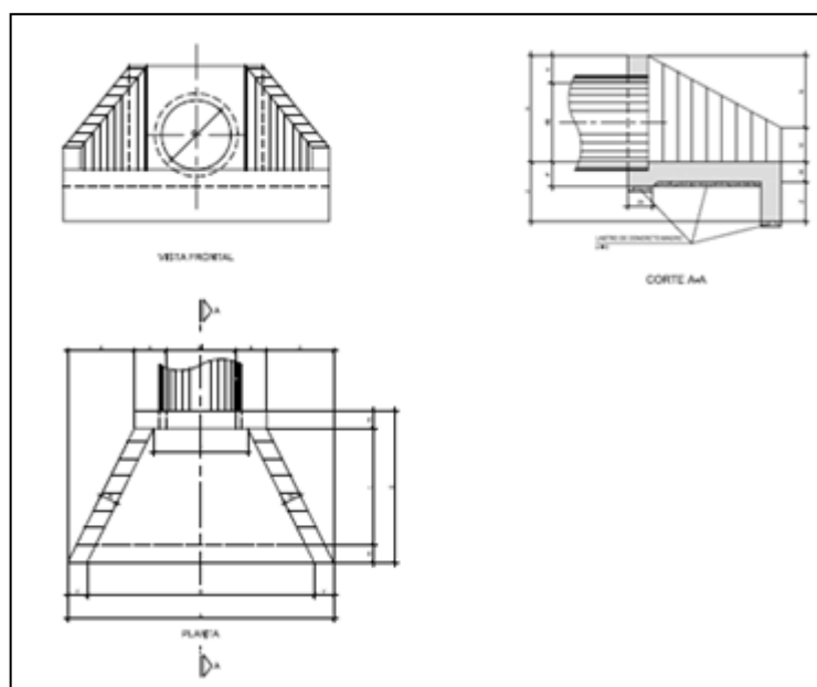
Figura 8.15 – Ala de saída de BSTC
