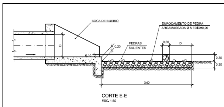
Figura 8.14 – Dissipador de energia
