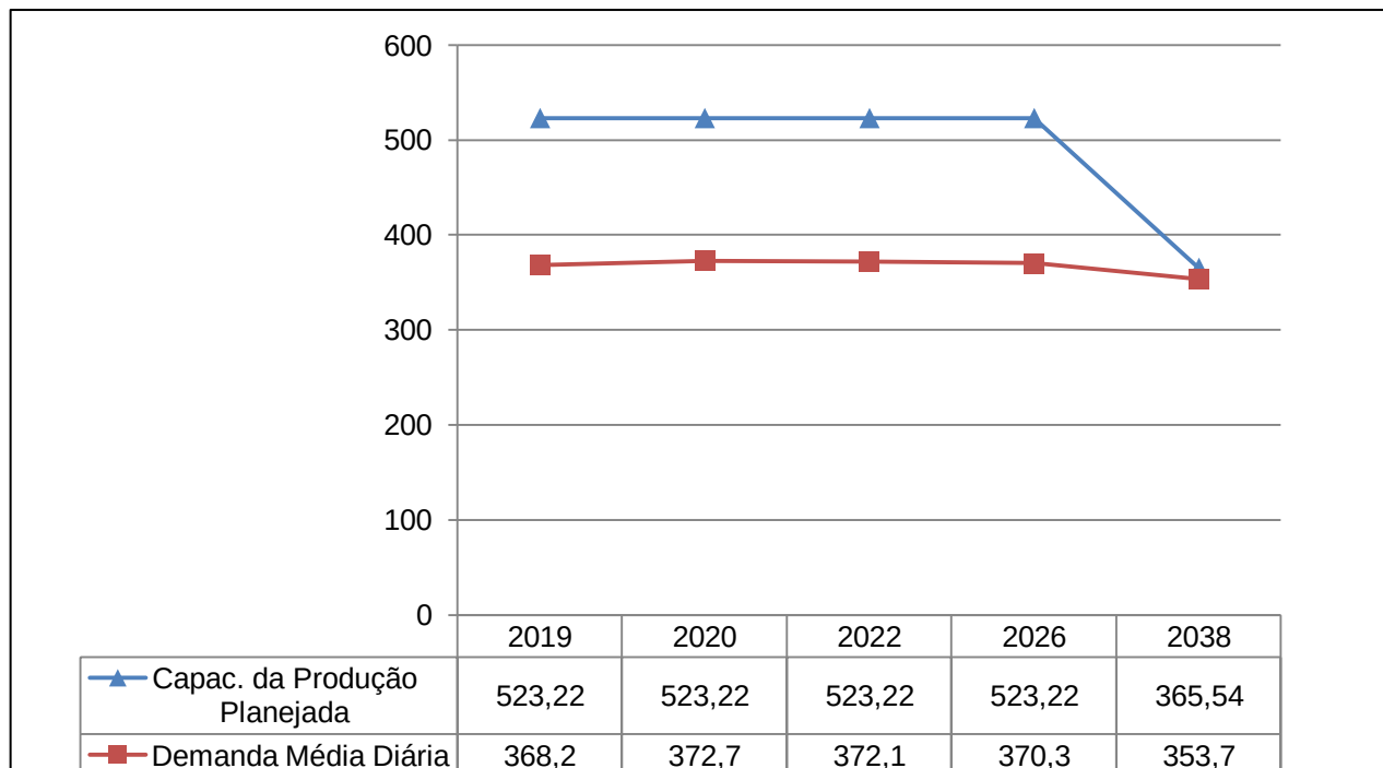
Gráfico 4.6 – Demandas Médias Diárias (l/s) x Capacidade de Produção (l/s) x Anos de Planejamento
