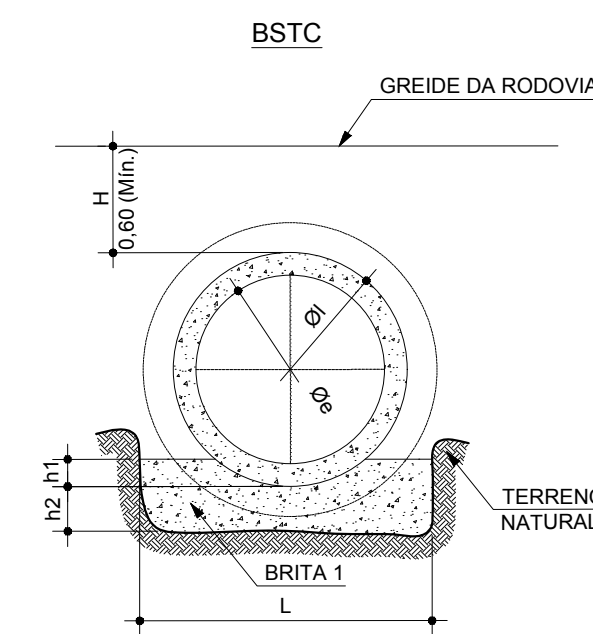
SEÇÃO PLANEJADA PARA O CANAL DE CONCRETO
