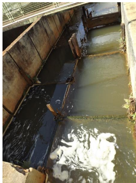
Foto 3.59 – Detalhe conjunto de floculadores retangulares chicaneados
