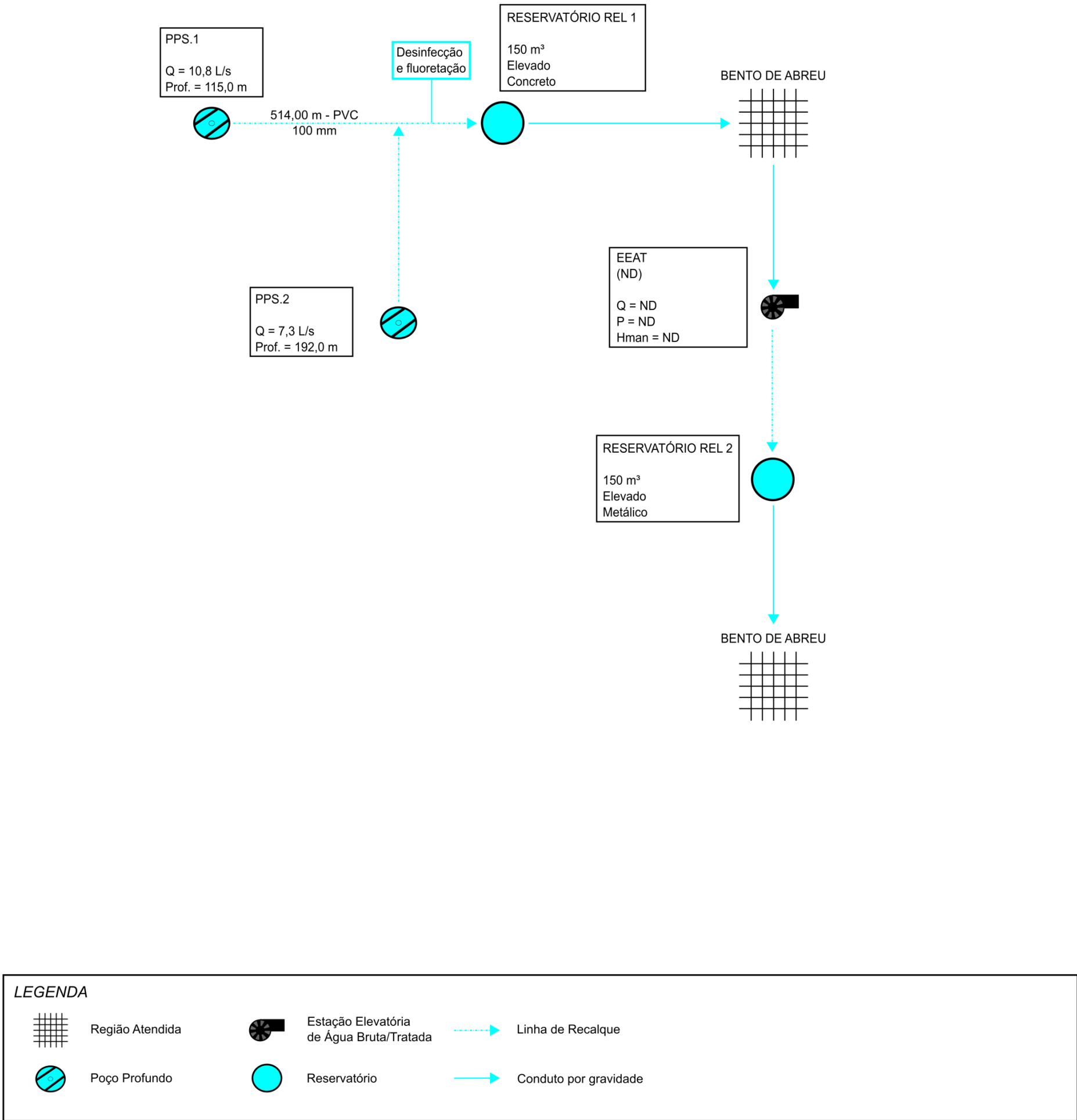
Figura 4.1 – Croqui do Sistema de Abastecimento de Água Sede ND: Não Disponível. Fonte: SABESP, 2021.
