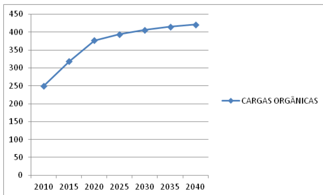
Gráfico 2.7 – Contribuições Diárias de Carga Orgânica (Kg DBO/dia) x Anos de Planejamento-Total Bofete
