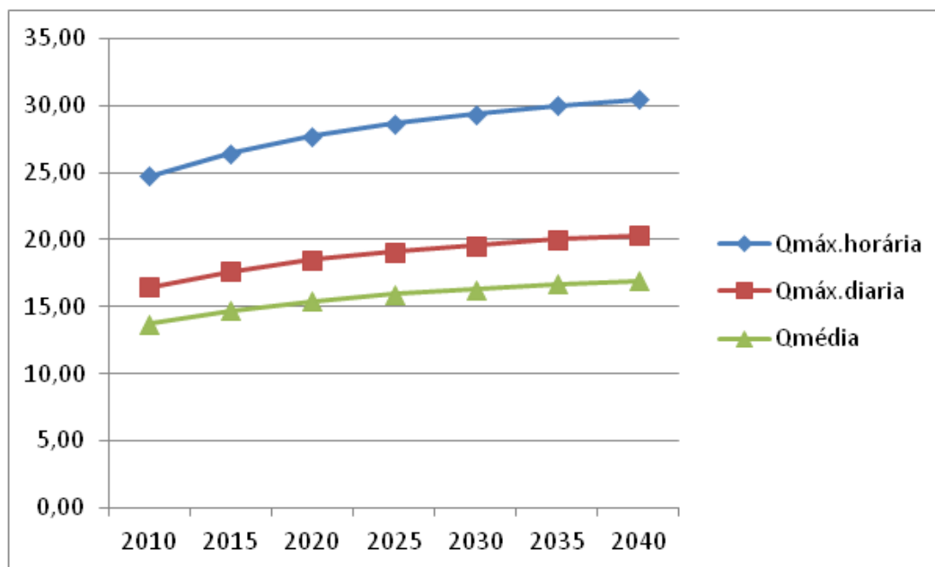
Gráfico 2.3– Demandas (l/s) x Anos de Planejamento-Total Bofete
