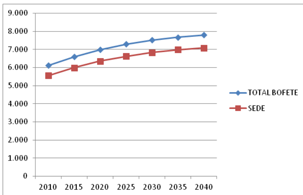
Gráfico 2.1– Populações Urbanas Atendidas (hab) x Anos de Planejamento-Total Bofete e Distrito Sede
