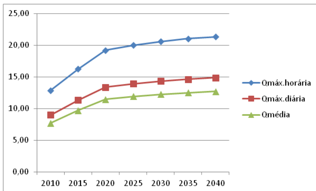
Gráfico 2.6 – Contribuições de Esgotos (l/s)x Anos de Planejamento-Total Bofete
