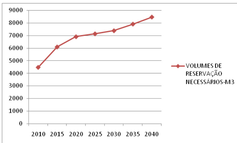
Gráfico 2.3 - Volumes de Reserva Necessários (l/s) x Anos de Planejamento
