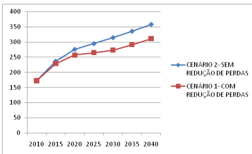
Gráfico 3.1 – Demandas Máximas Diárias (l/s) x Anos de Planejamento.
