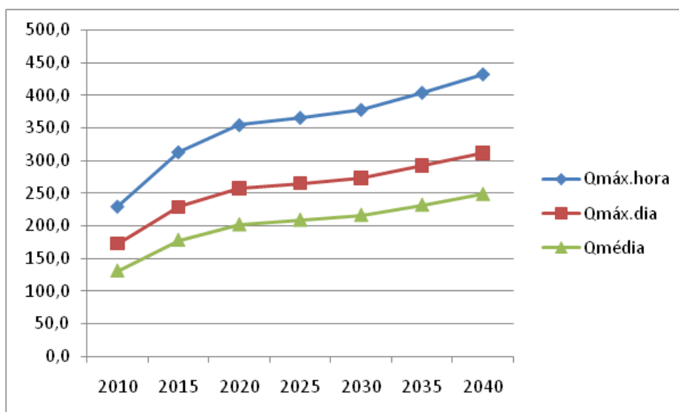
Gráfico 2.2 - Demandas (l/s) x Anos de Planejamento
