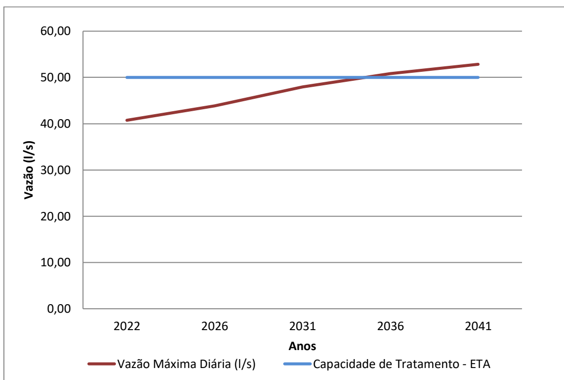
Gráfico 8.1 – Demandas Máximas Diárias (l/s) X Capacidade de Tratamento (l/s)
