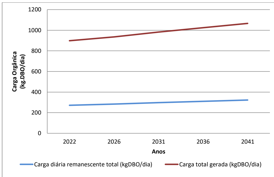
Gráfico 8.6 - Evolução de Cargas Orgânicas (Kg DBO/Dia)
