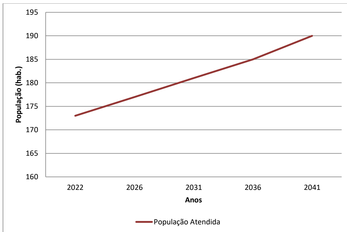
Gráfico 7.6 - População Atendida (hab.) x Anos de Planejamento – Bairro Aracaçu
