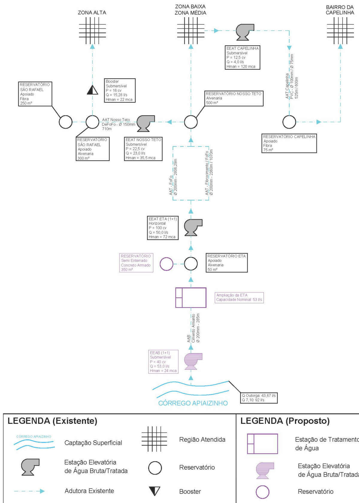
Figura 10.1 – Croqui do Sistema de Abastecimento de Água Proposto para Sede Urbana
