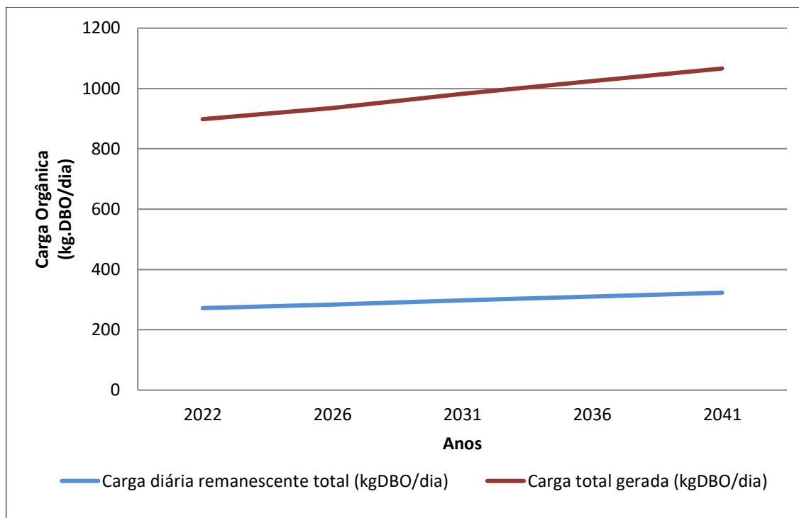
Gráfico 8.8 - Evolução de Cargas Orgânicas (Kg DBO/Dia)
