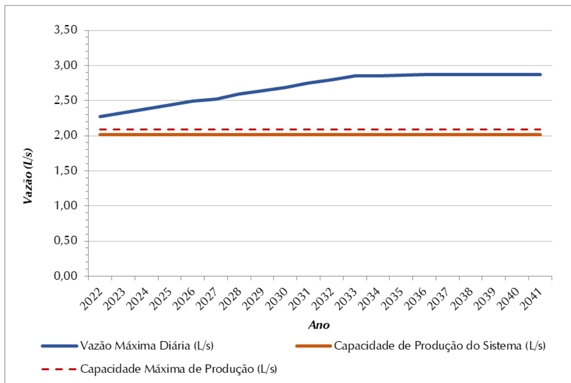
Figura 8.4 – Demandas Máximas Diárias (L/s) X Vazão Captada (L/s) – SAA Iubatinga/Esperança d'Oeste
