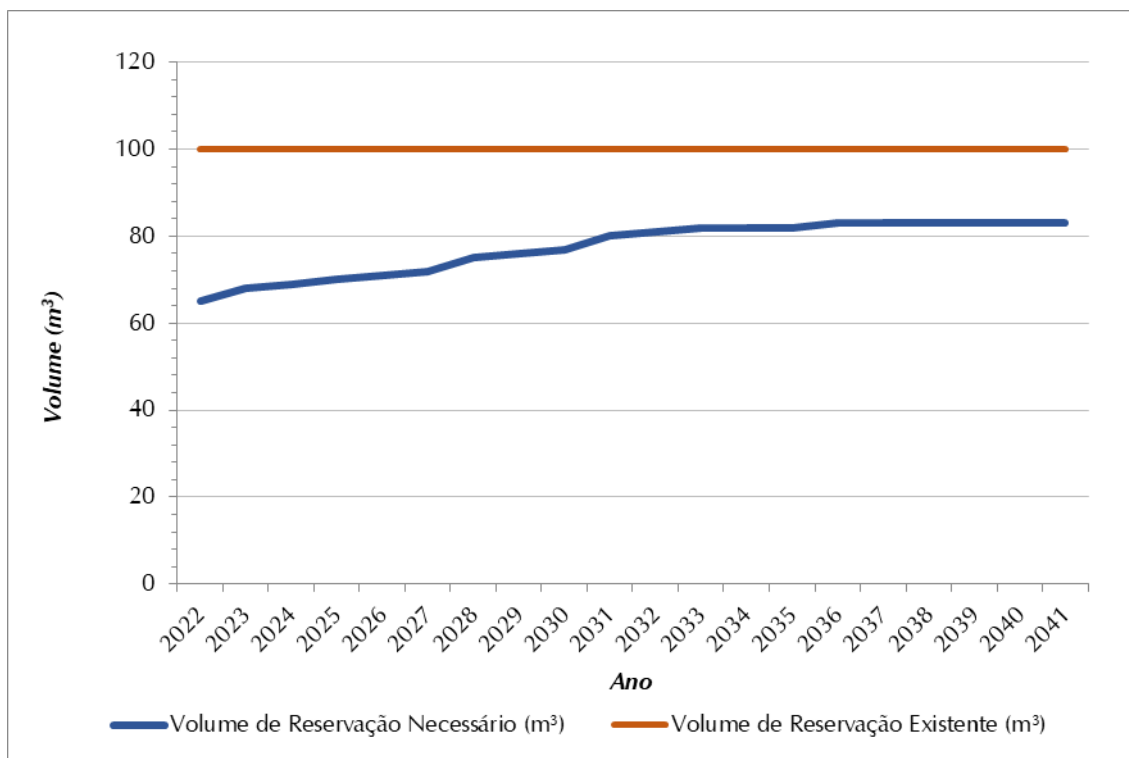
Figura 8.5 - Volume de Reservação Necessário (m³) x Volume de Reservação Atual (m³) – SAA Iubatinga/Esperança d'Oeste
