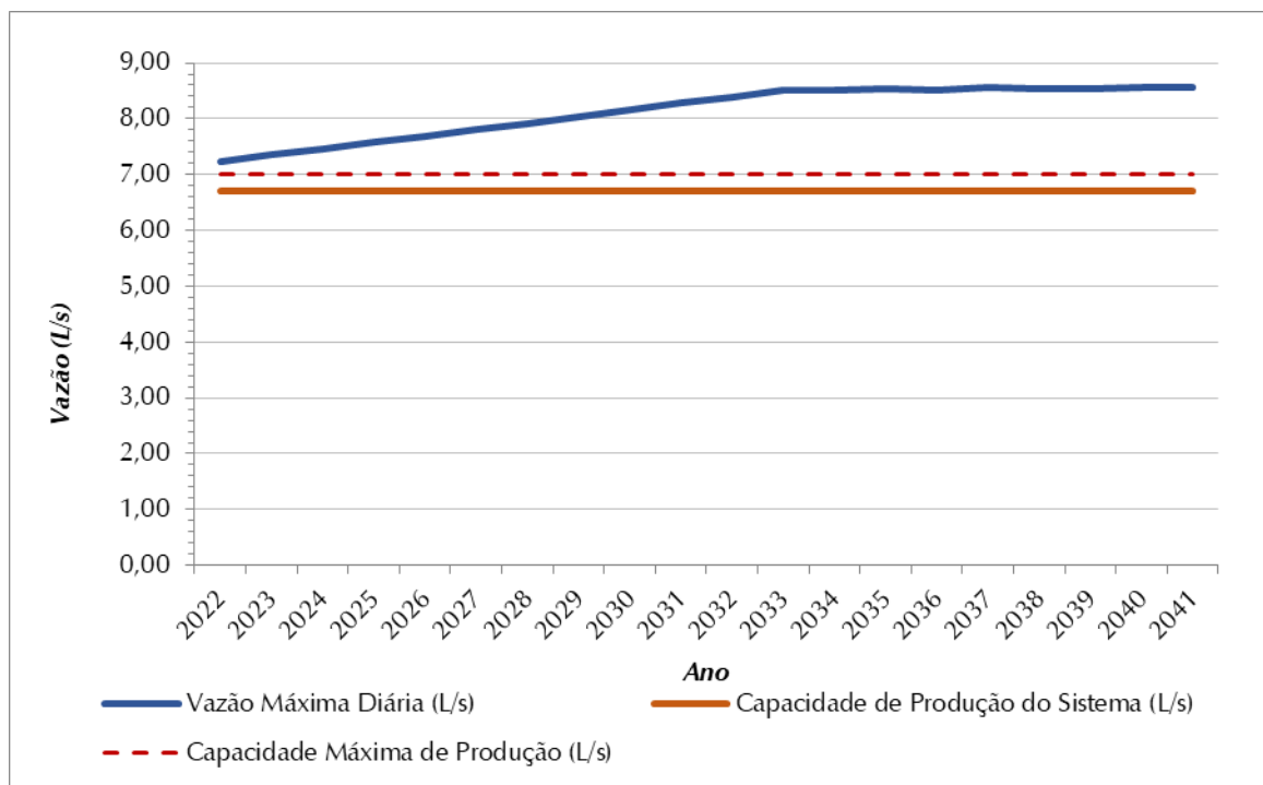
Figura 8.1 – Demandas Máximas Diárias (L/s) X Vazão Captada (L/s) – SAA Sede/Graminha
