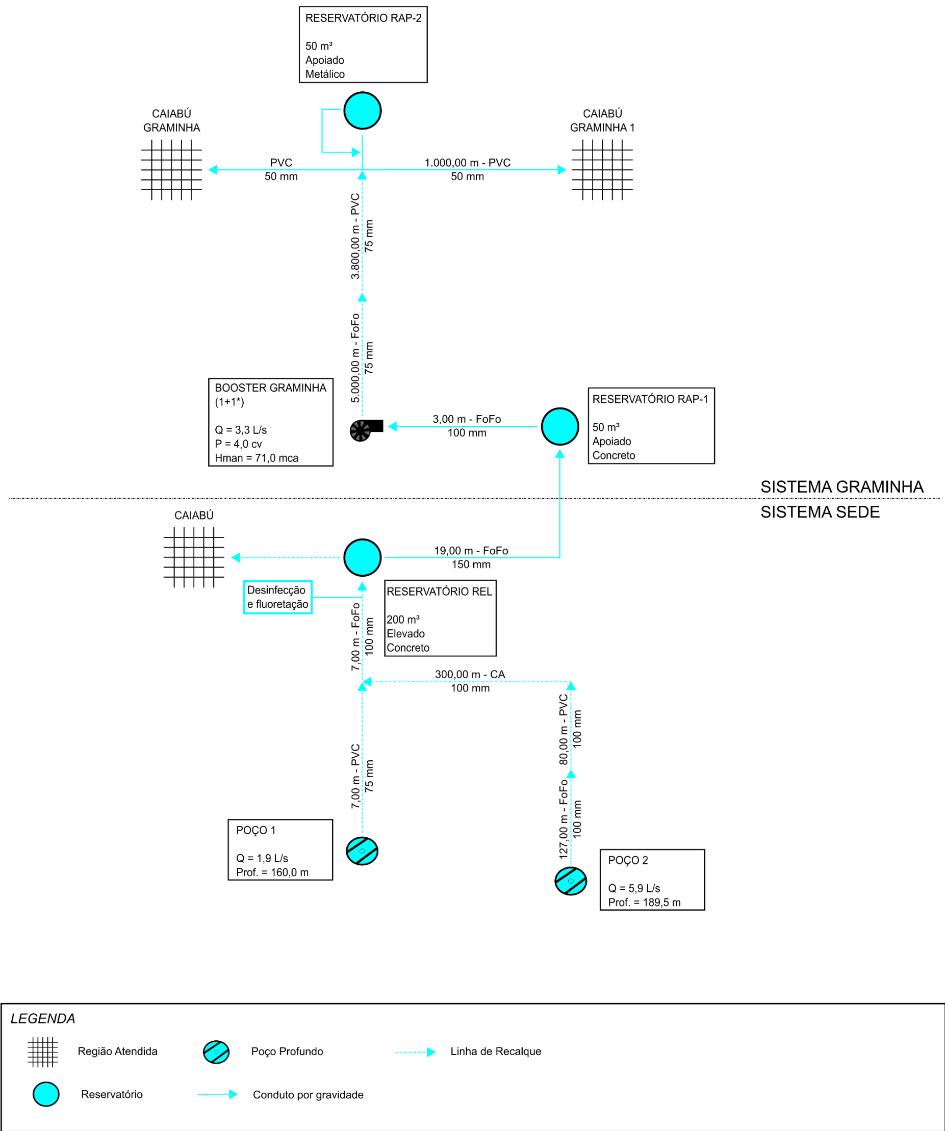
Figura 4.1 – Croqui do Sistema de Abastecimento de Água Sede/Graminha
