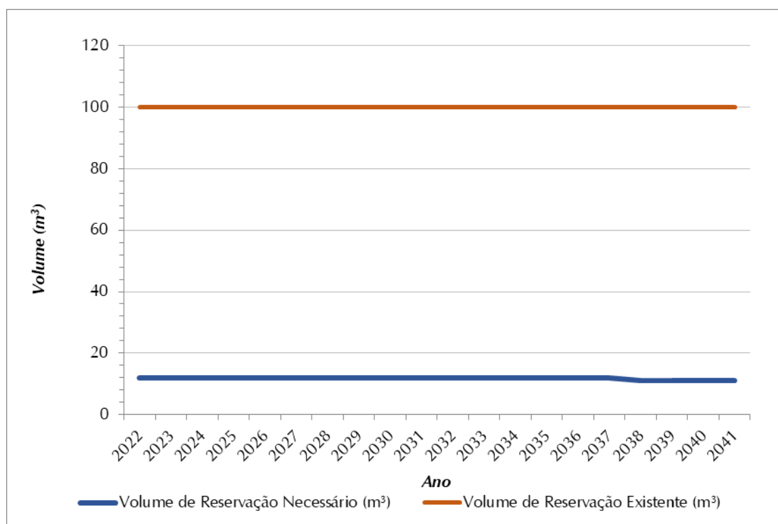
Figura 8.3 - Volume de Reservação Necessário (m³) x Volume de Reservação Atual (m³) – SAA Graminha
