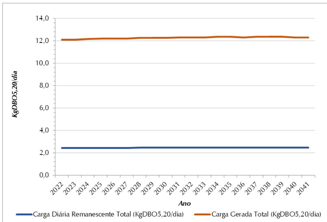
Figura 8.11 - Evolução de Cargas Orgânicas (Kg DBO 5,20 /Dia) – SES Esperança d'Oeste
