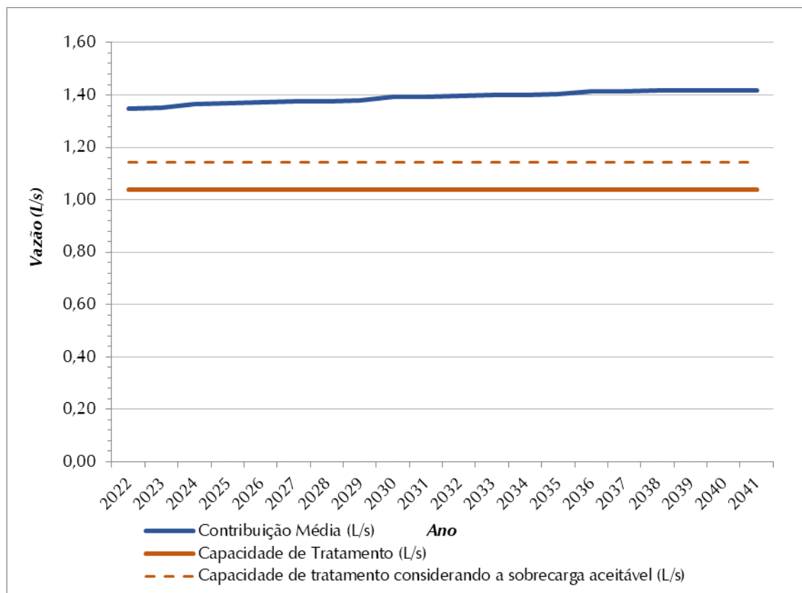
Figura 8.8 – Contribuição Média Total (L/s) x Capacidade de Tratamento de Esgoto (L/s) – SES Iubatinga
