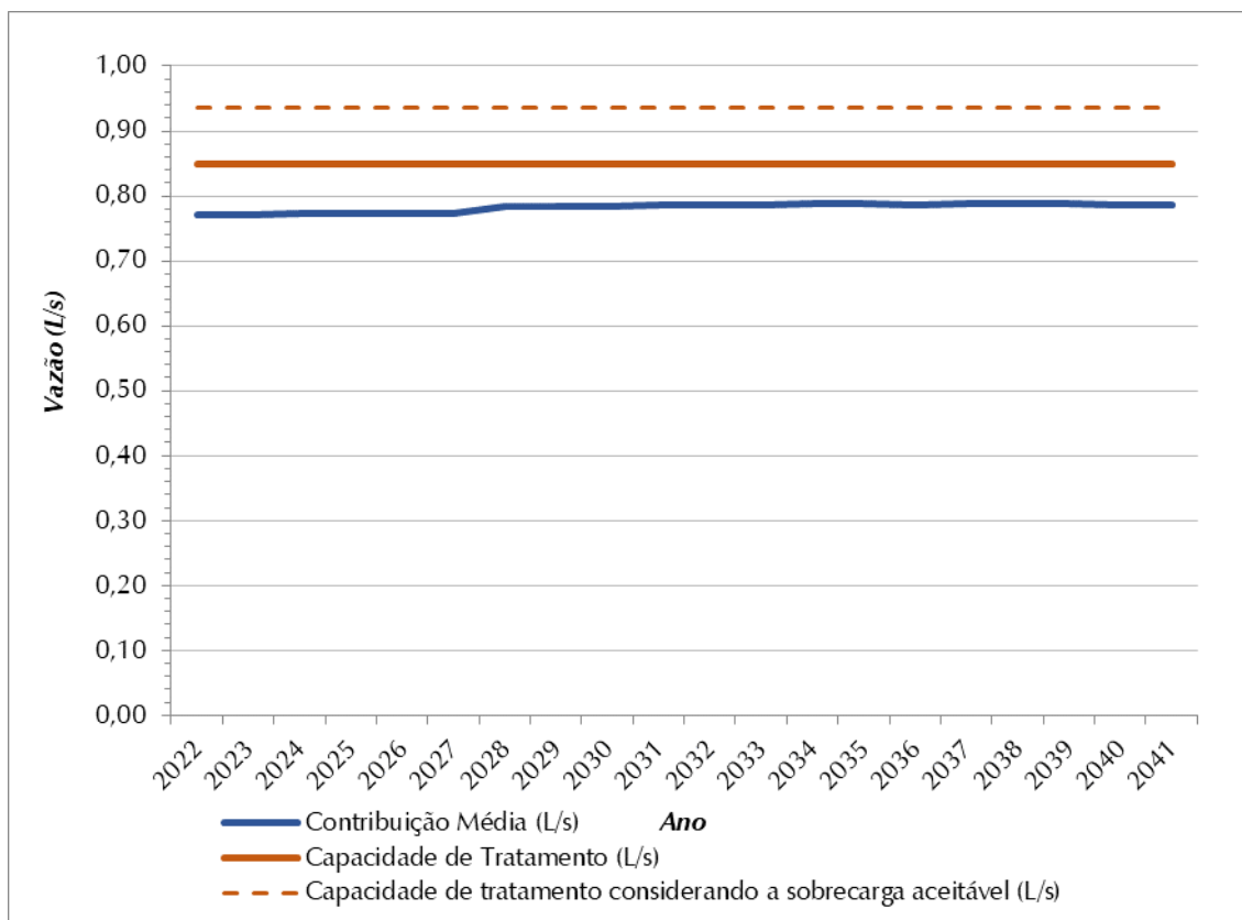
Figura 8.10 – Contribuição Média Total (L/s) x Capacidade de Tratamento de Esgoto (L/s) – SES Esperança d'Oeste
