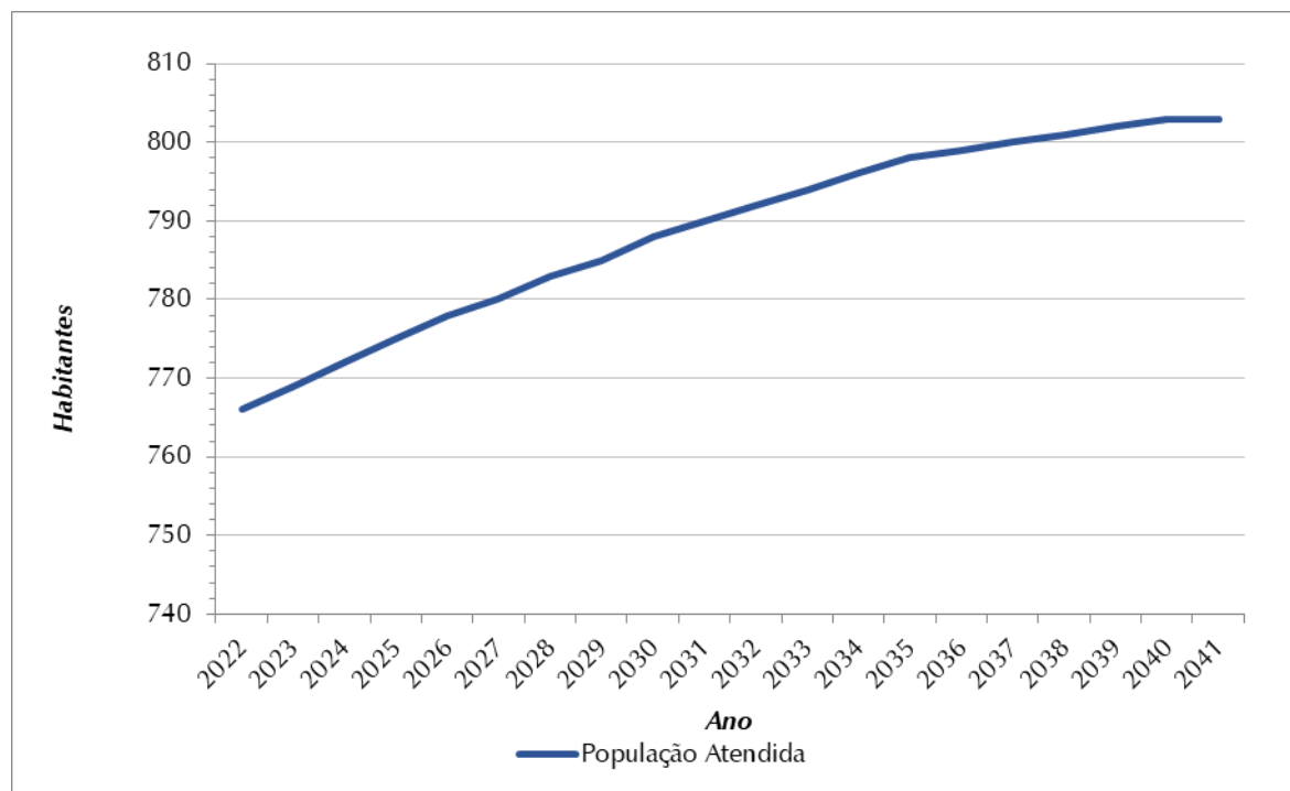
Figura 7.4 – Evolução da População Atendida (hab.) – SAA Iubatinga
