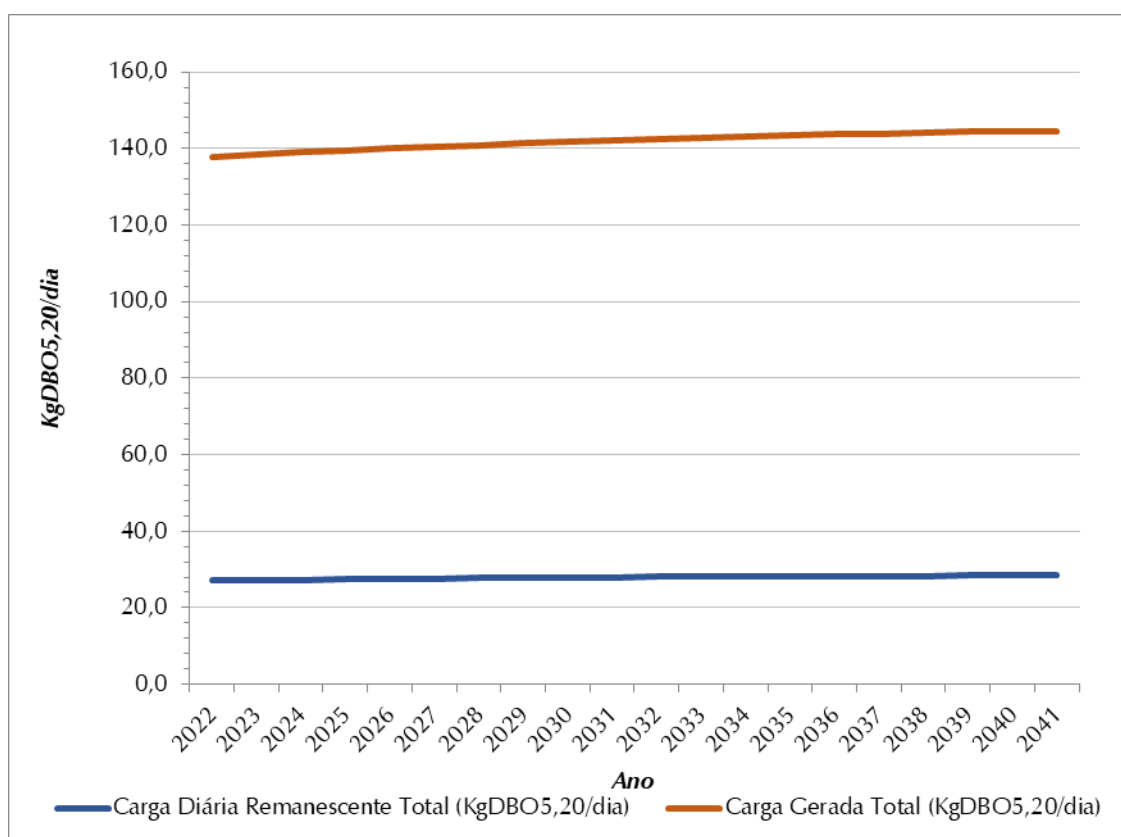
Figura 8.7 - Evolução de Cargas Orgânicas (Kg DBO 5,20 /Dia)
