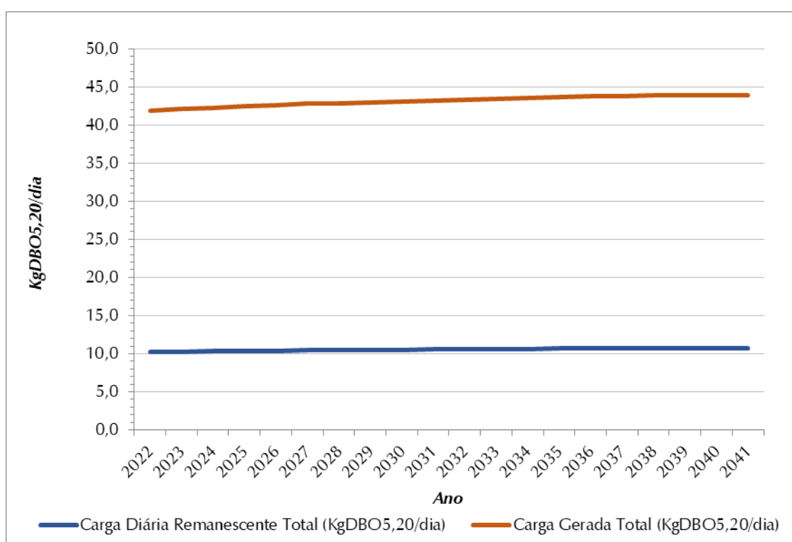
Figura 8.9 - Evolução de Cargas Orgânicas (Kg DBO 5,20 /Dia) – SES Iubatinga
