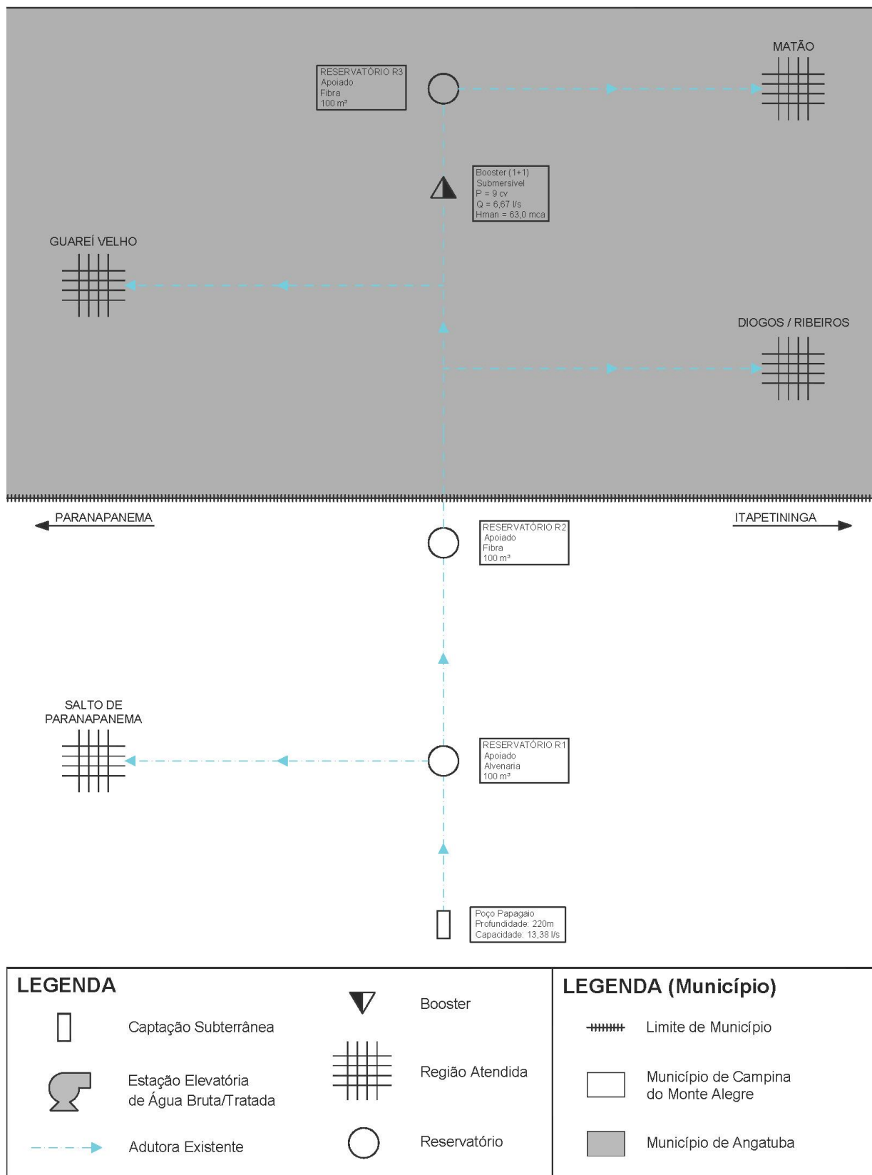
Figura 4.2 – Croqui do Sistema de Abastecimento de Água Existente – Distrito Salto de Paranapanema.
