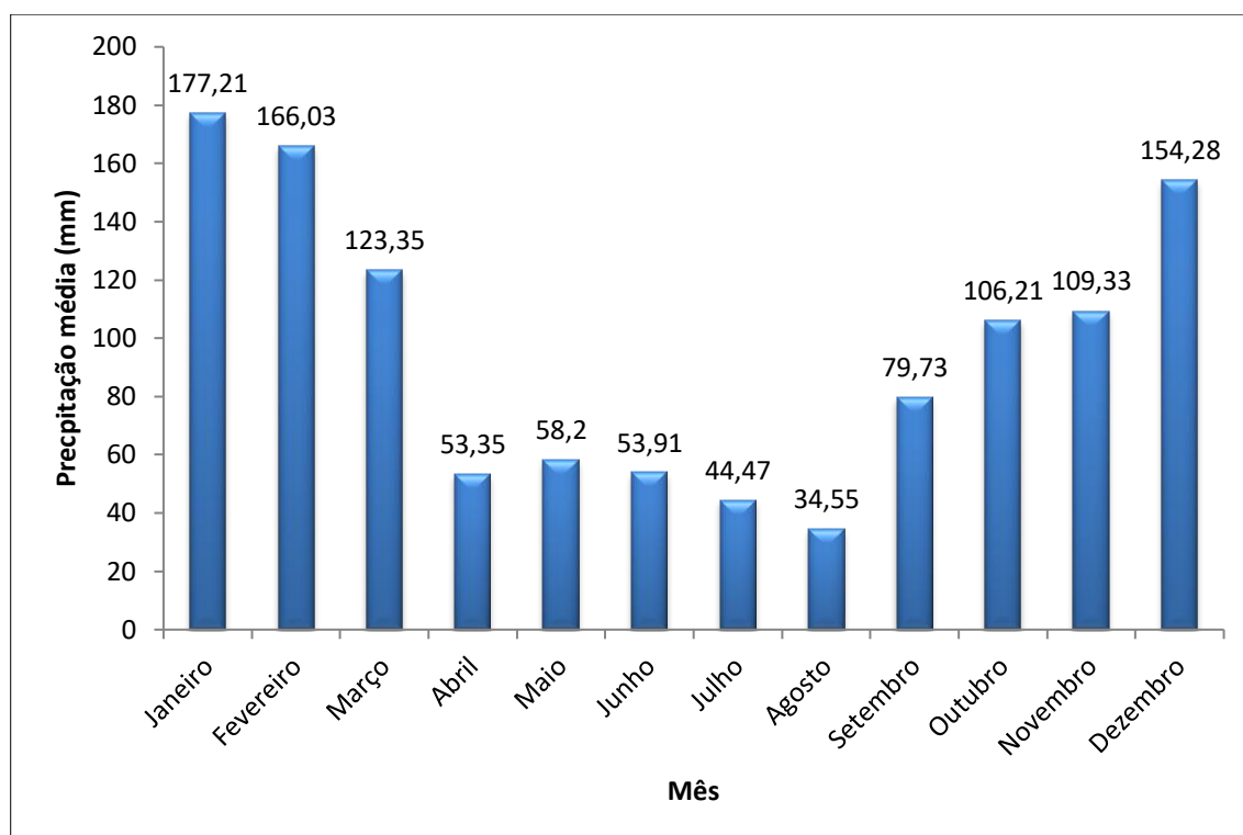
Gráfico 3.1 – Precipitação Média Mensal no Período de 1939 a 1998, Estação E5-018
