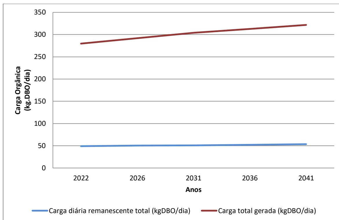
Gráfico 8.4 - Evolução de Cargas Orgânicas (Kg DBO/Dia)
