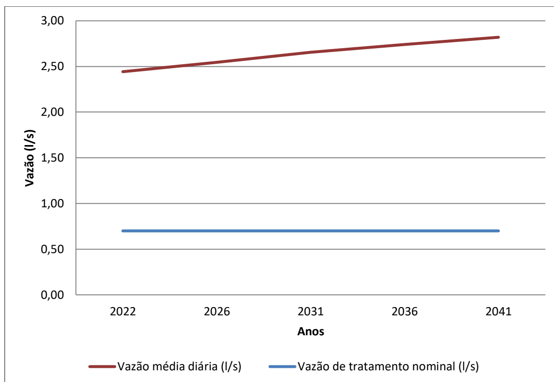
Gráfico 8.5 – Vazão Média Diária (l/s) x Capacidade nominal da ETE (l/s)
