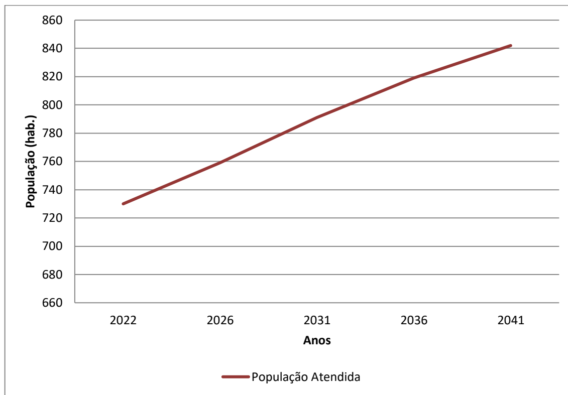
Gráfico 7.5 - População Atendida (hab.) x Anos de Planejamento – Distrito Salto de Paranapanema
