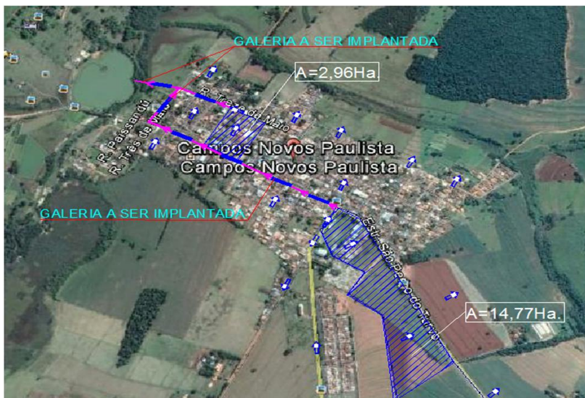
Ilustração 4.2 – Determinação das áreas das bacias de contribuição
