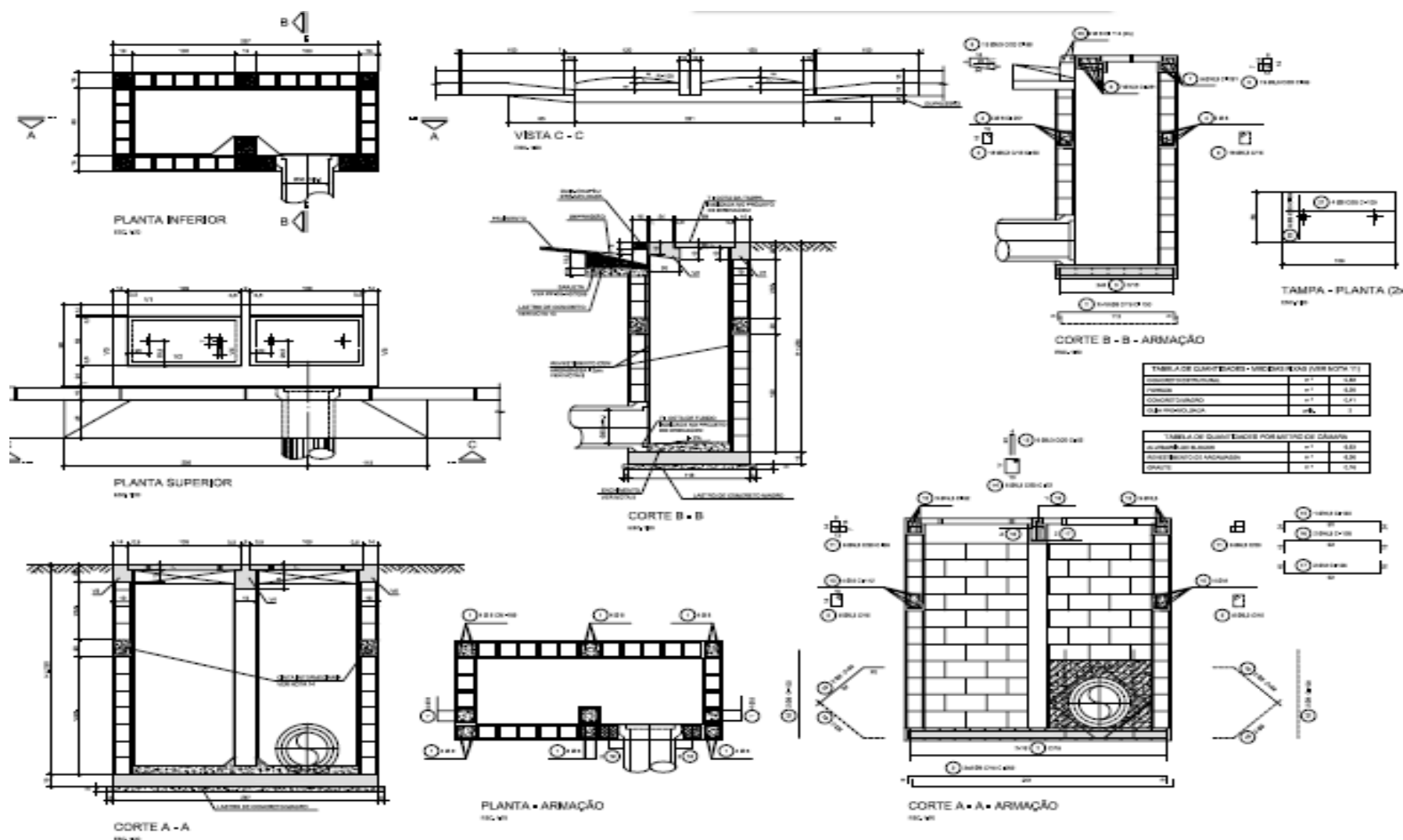
Ilustração 8.3 – Boca de lobo dupla
