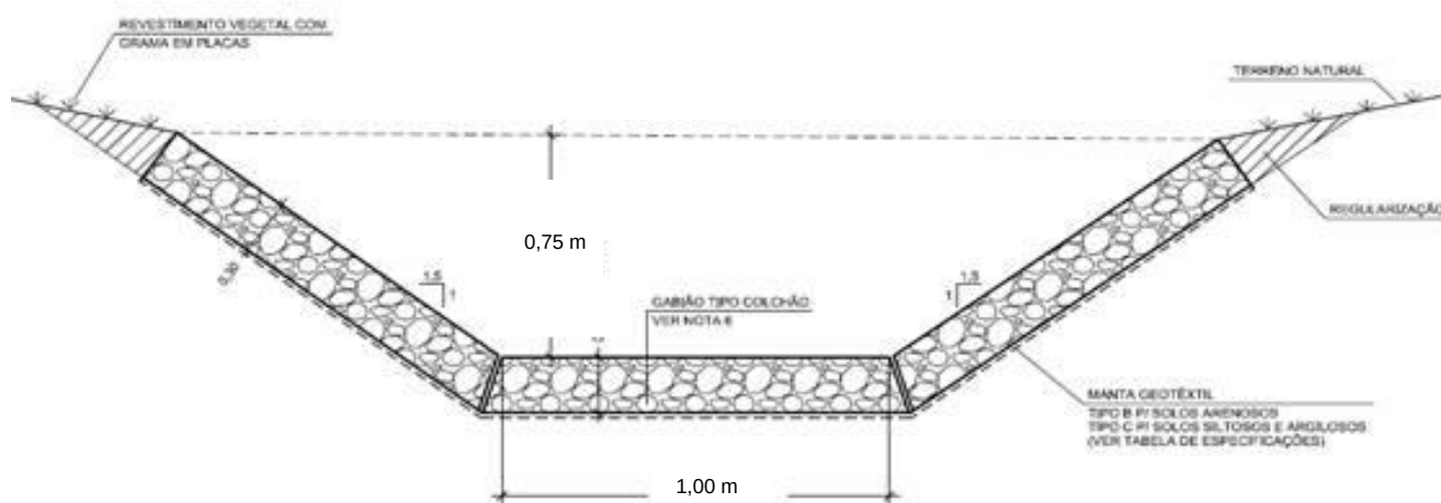
Ilustração 8.7 - Seção planejada para o canal trapezoidal.
