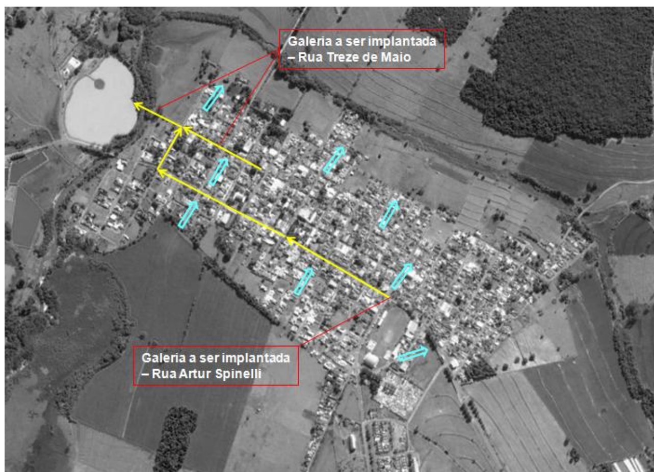
Ilustração 4.3 – Traçado preliminar das galerias
