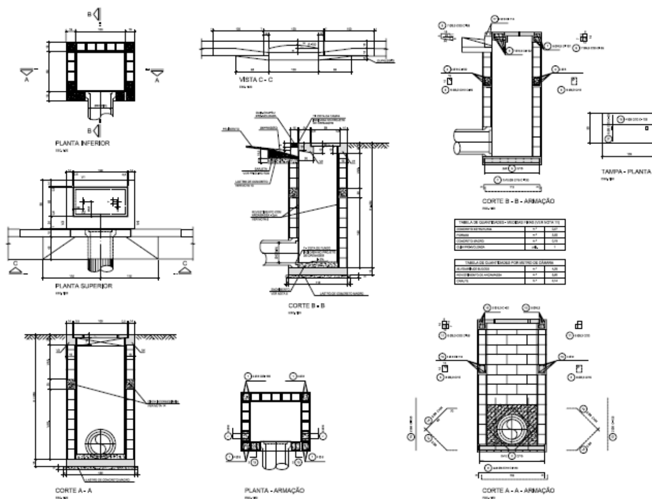
Ilustração 8.2 – Boca de lobo simples
