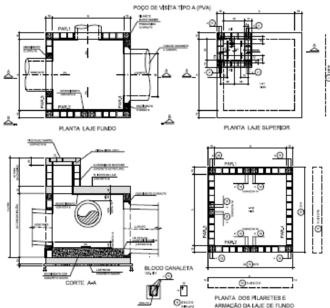
Ilustração 8.5 – Poço de Visita
