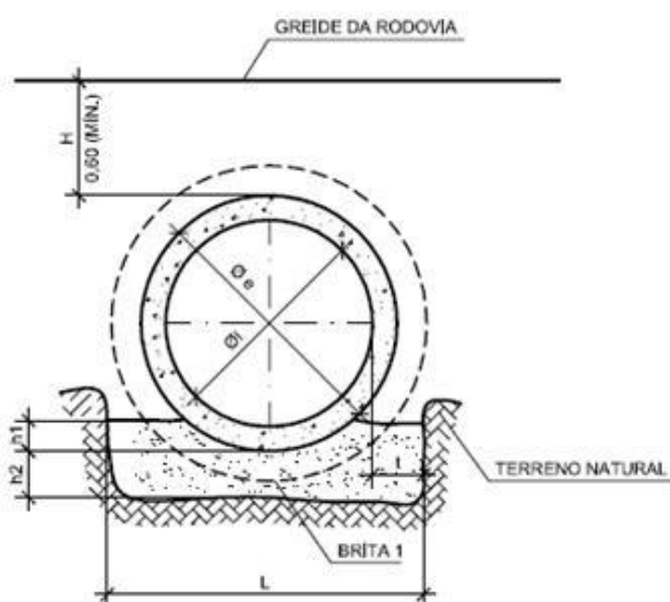
Ilustração 8.6 – Assentamento de tubulações
