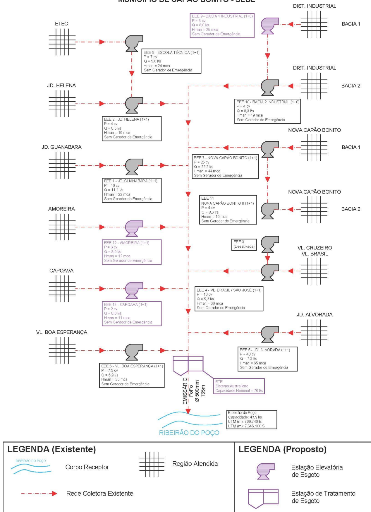
Figura 10.3 – Croqui do Sistema de Esgotamento Sanitário Proposto para o Subsistema da Sede Urbana
