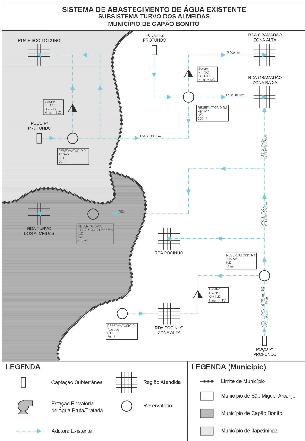
Figura 4.6 – Croqui do Sistema de Abastecimento de Água Existente – Turvo dos Almeida.
