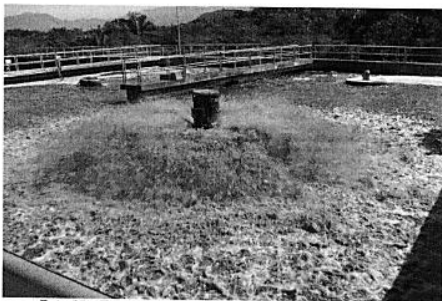
Foto 25 – Tanques de Aeração/Sedimentação da ETE Indaiá
