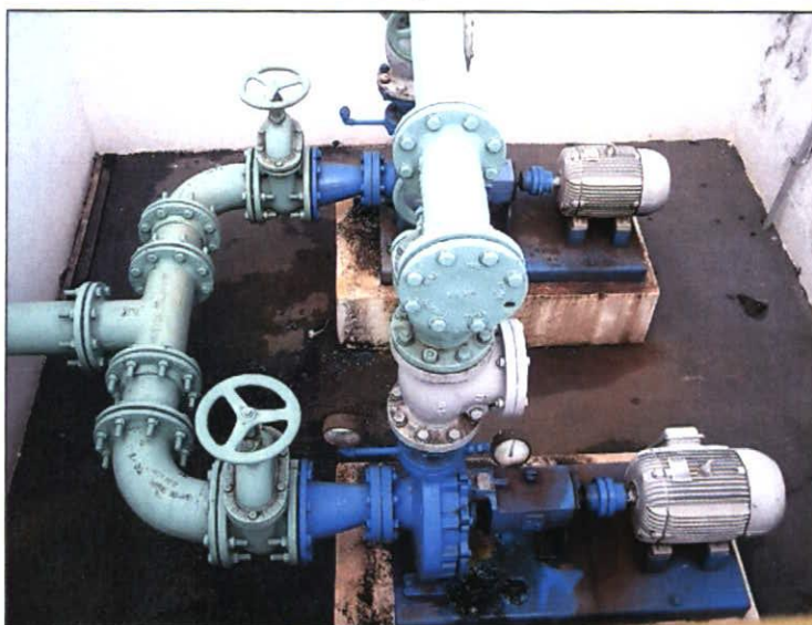
Foto 17 - Estação elevatória de água tratada EEAT02 - Colômbia
