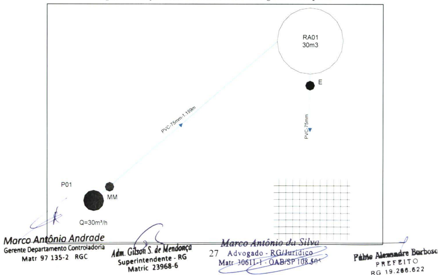
Figura 5 - Croqui: Sistema de abastecimento de água de Laranjeiras
