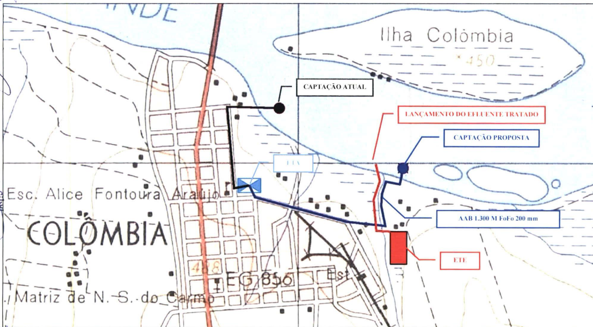
Figura 14 - Novo sistema de adução de água bruta
