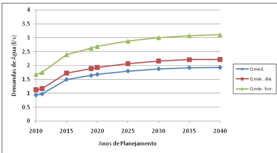
Gráfico 2.5 – Evolução das Demandas/Vazões Disponibilizadas para Distribuição – Distrito de Juquiratiba
