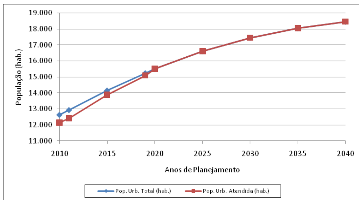
Gráfico 2.7 – População Urbana Total X População Esgotada – Distrito Sede
