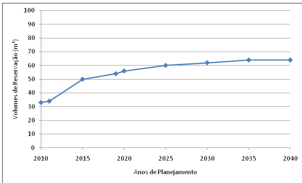
Gráfico 2.6 – Evolução dos Volumes de Reservação Necessários – Distrito de Juquiratiba
