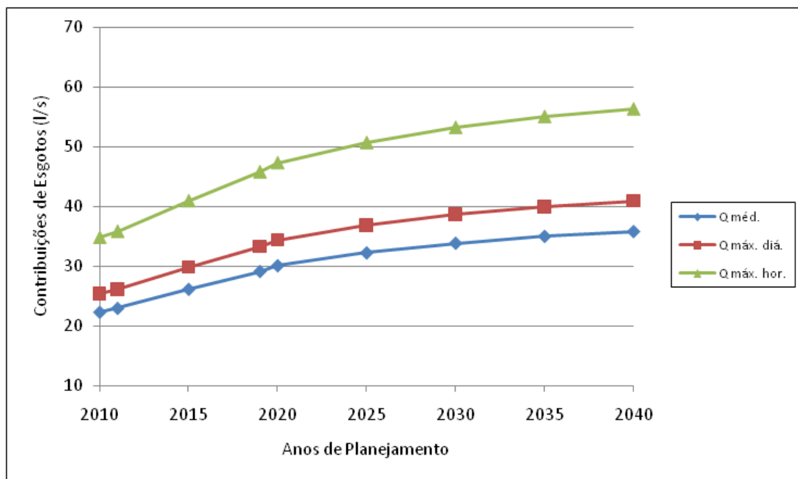
Gráfico 2.9 – Evolução das Contribuições de Esgotos – Distrito Sede
