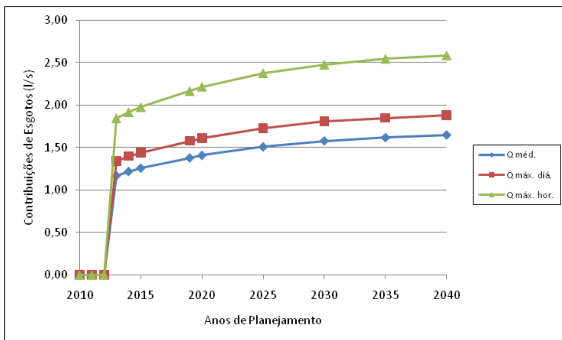
Gráfico 2.11 – Evolução das Contribuições de Esgotos – Distrito de Juquiratiba
