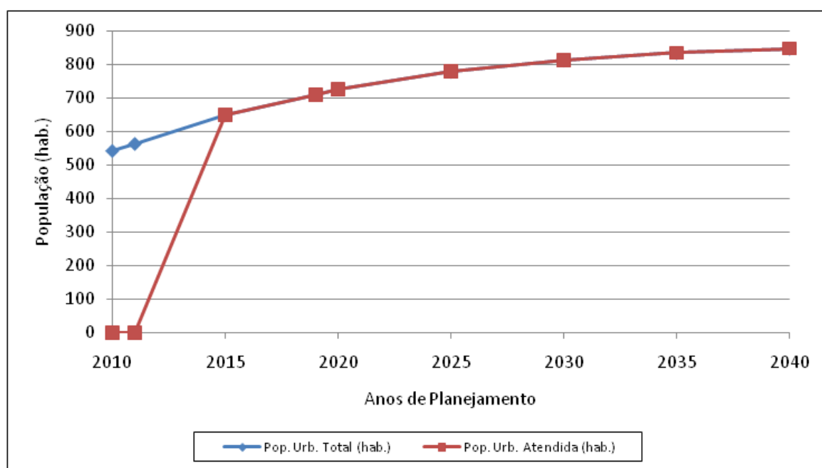
Gráfico 2.8 – População Urbana Total X População Esgotada – Distrito de Juquiratiba
