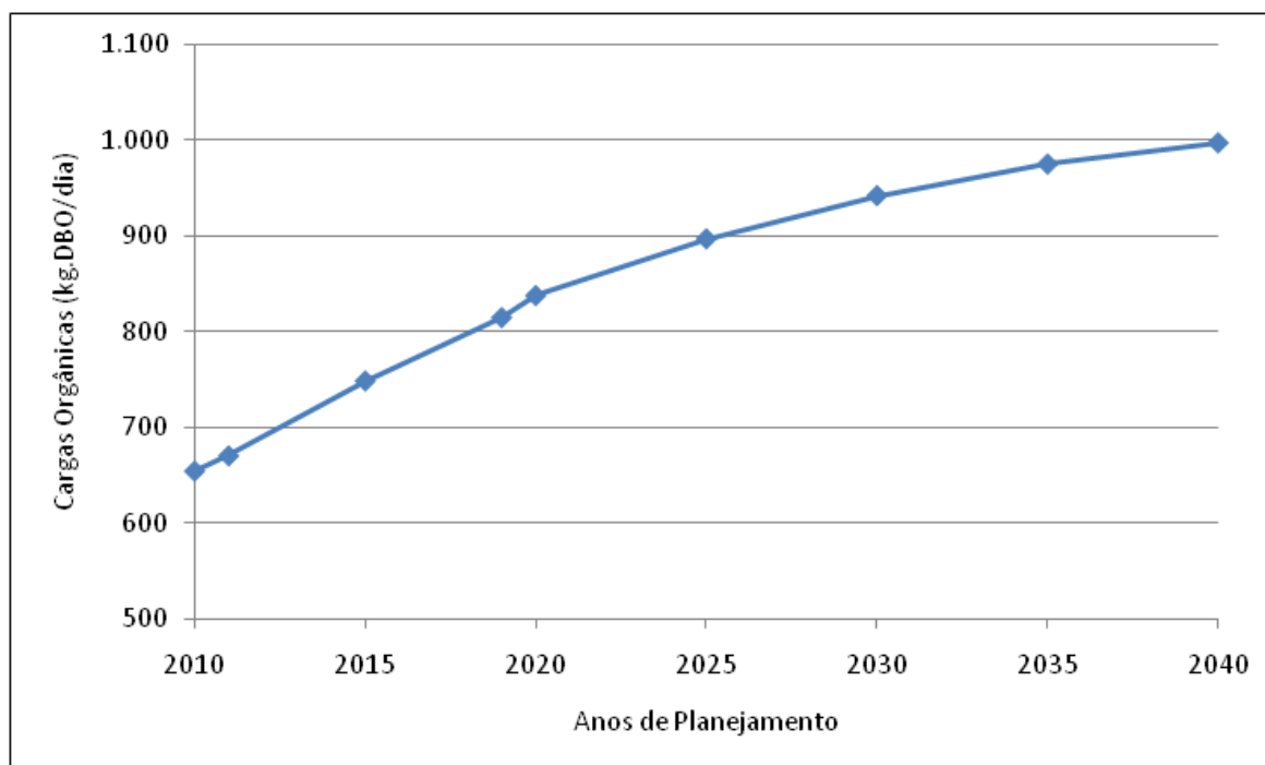
Gráfico 2.10 – Evolução das Cargas Orgânicas Diárias – Distrito Sede
