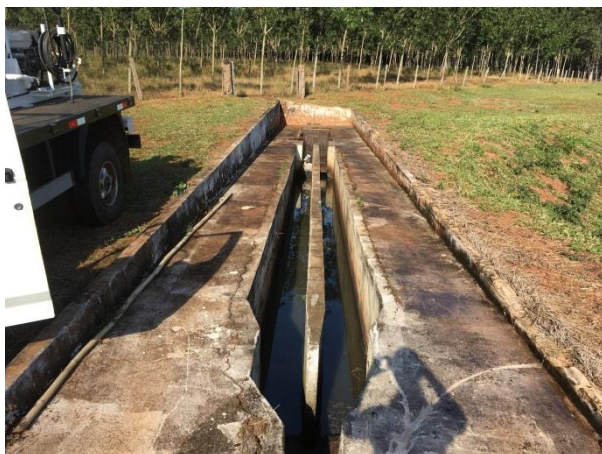
Foto 3.41 – Vista geral do tratamento preliminar ETE Vila Nova
