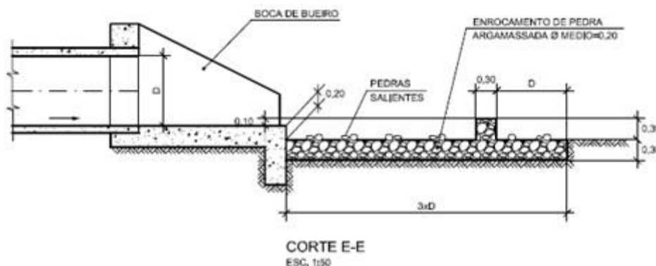
Ilustração 8.3 – Dissipador de energia
