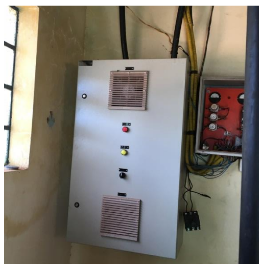
Foto 3.15 – Painel elétrico das bombas da EEAT 01
