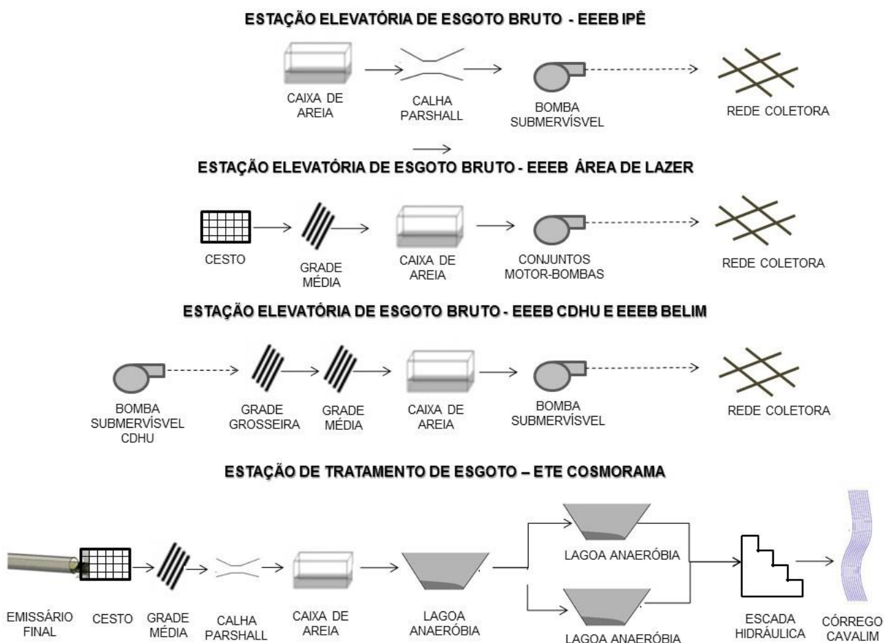
Ilustração 3.3 – Fluxograma do sistema de esgotamento sanitário Sede Cosmorama
