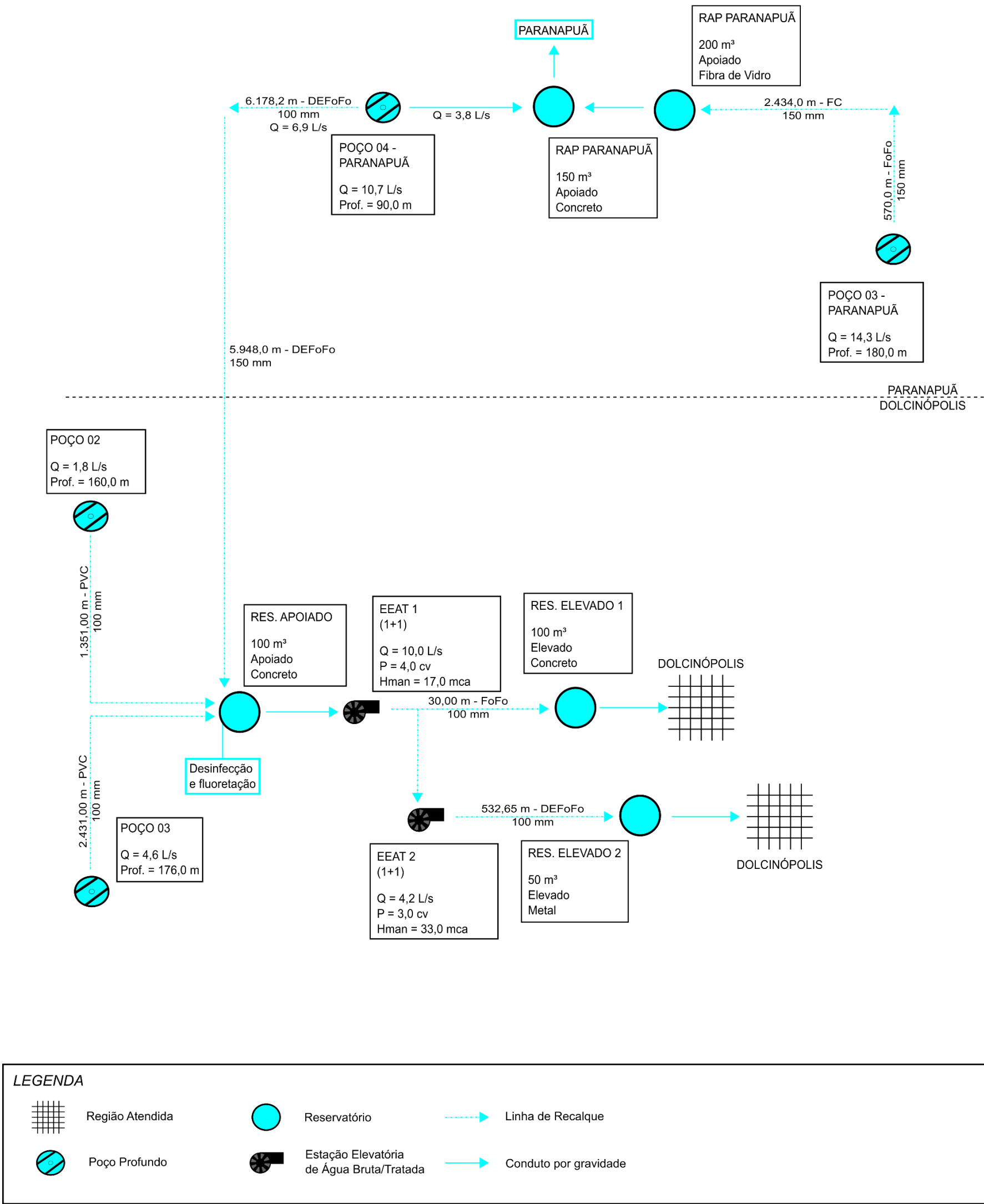
Figura 4.1 – Croqui do Sistema de Abastecimento de Água Sede Fonte: SABESP, 2020.
