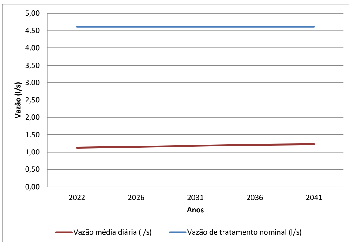
Gráfico 8.9 – Vazão Média Diária (l/s) x Capacidade nominal da ETE (l/s)
