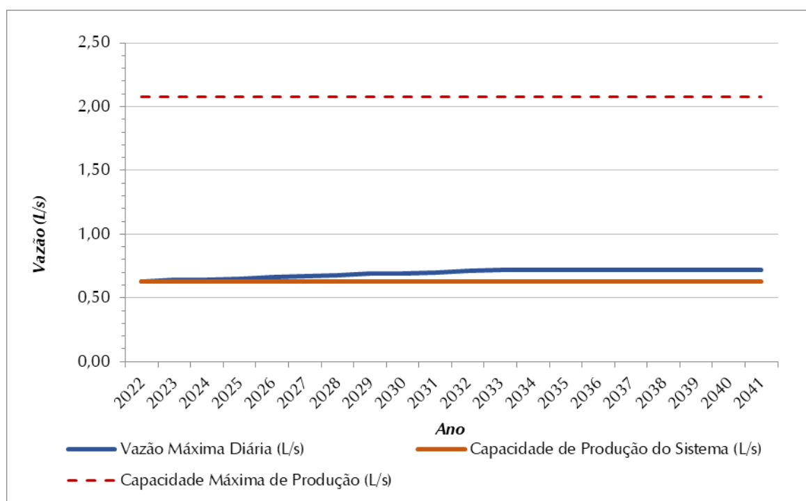
Figura 8.5 – Demandas Máximas Diárias (L/s) X Vazão Captada (L/s) – SAA Rosanela
