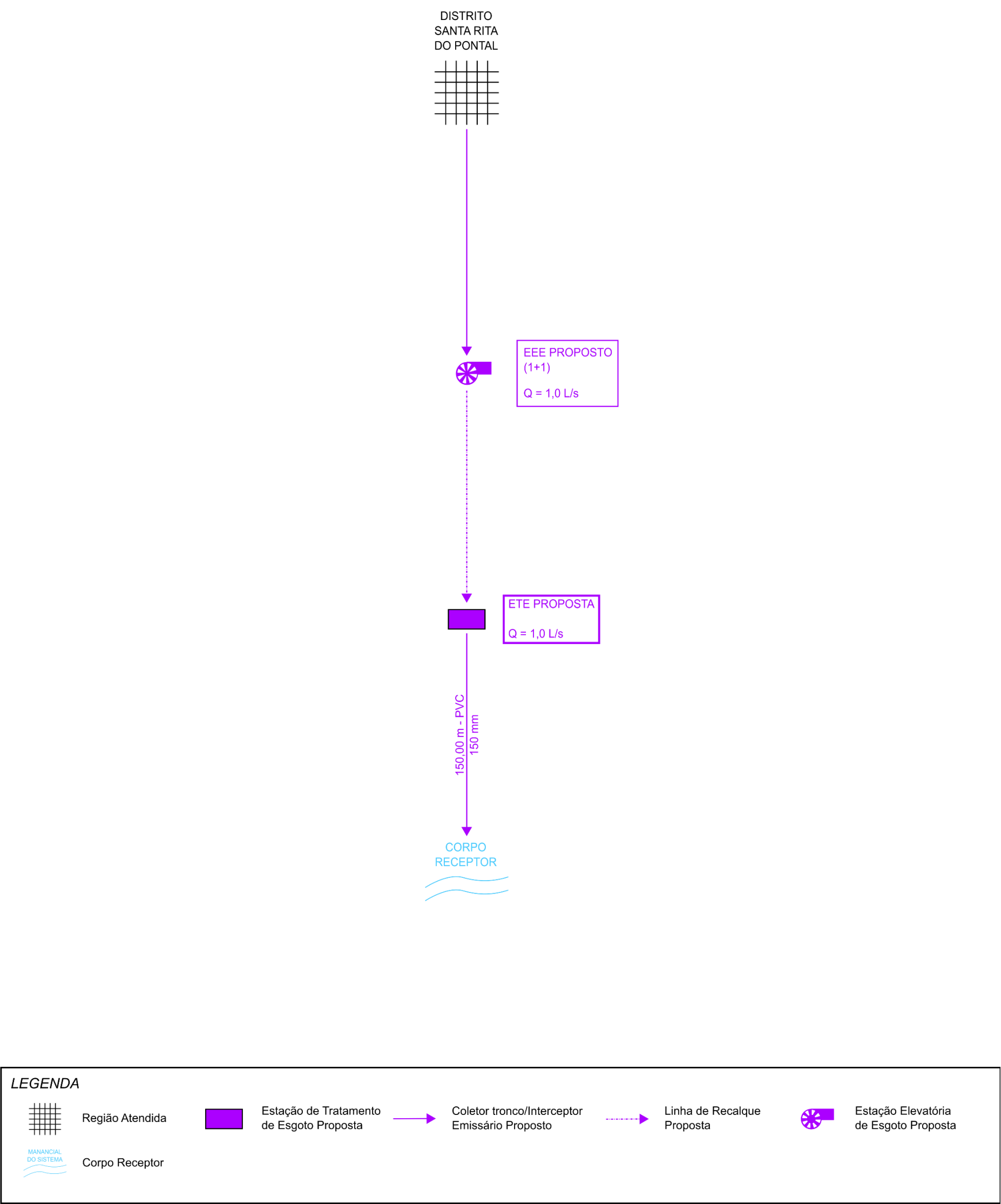
Figura 10.3 – Croqui das intervenções propostas para o sistema de esgotamento sanitário Santa Rita do Pontal
