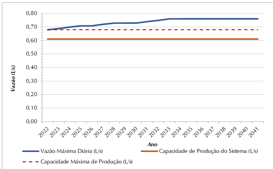
Figura 8.3 – Demandas Máximas Diárias (L/s) X Vazão Captada (L/s) – SAA Santa Rita do Pontal
