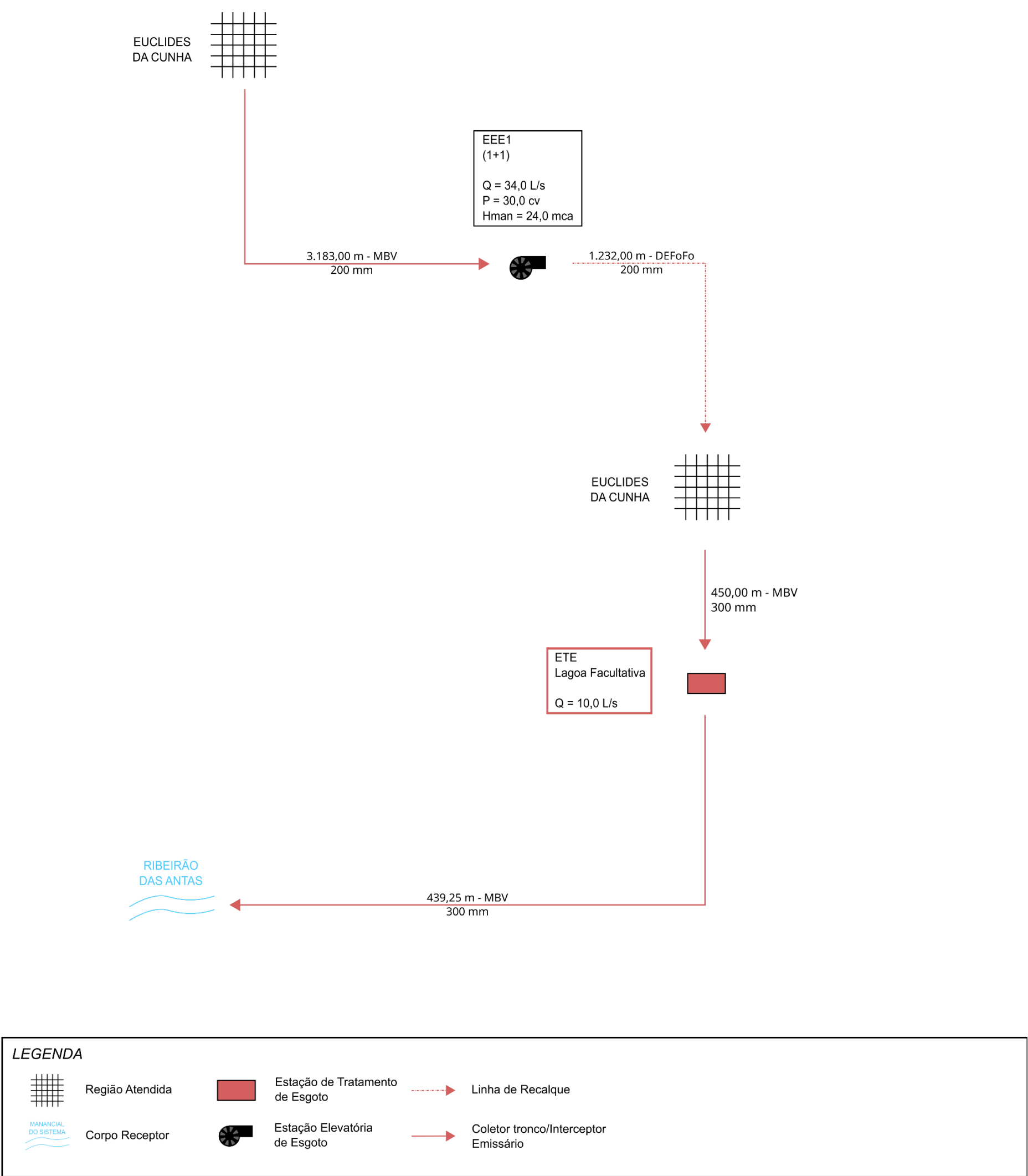
Figura 4.4 – Croqui do Sistema de Esgotamento Sanitário da Sede de Euclides da Cunha Paulista
