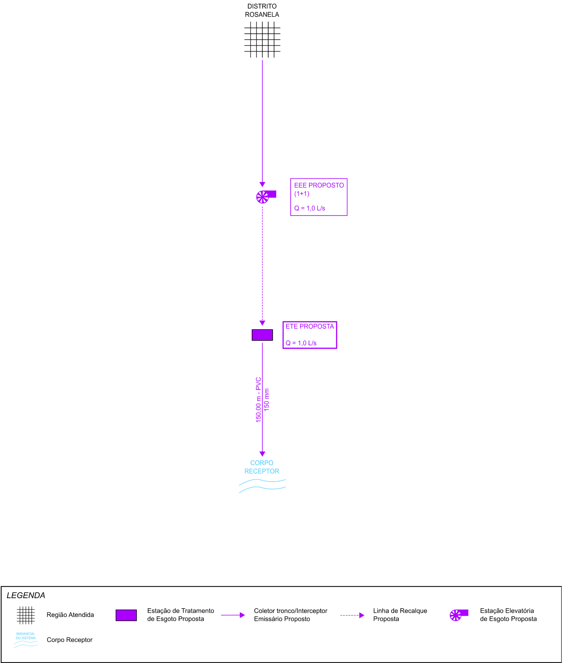
Figura 10.4 – Croqui das intervenções propostas para o sistema de esgotamento sanitário Rosanela
