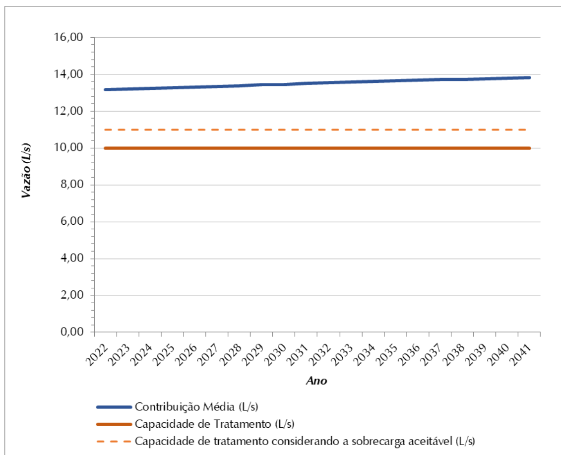
Figura 8.7 – Contribuição Média Total (L/s) x Capacidade de Tratamento de Esgoto (L/s) – SES Sede
