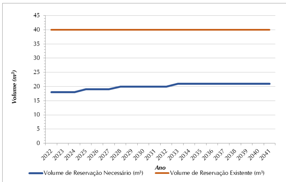
Figura 8.6 - Volume de Reservação Necessário (m³) x Volume de Reservação Atual (m³) SAA Rosanela
