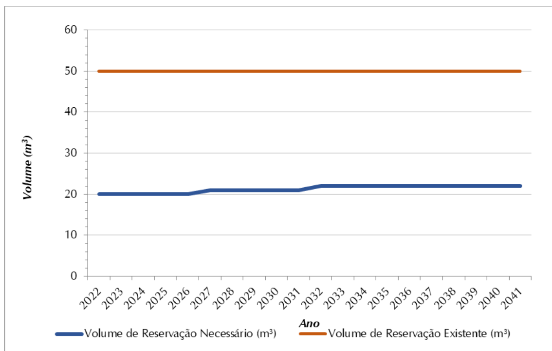
Figura 8.4 - Volume de Reservação Necessário (m³) x Volume de Reservação Atual (m³) SAA Santa Rita do Pontal
