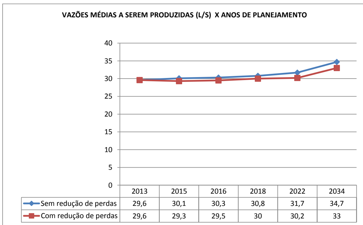
Gráfico 3.3 – Vazões Médias a serem Produzidas (L/s) x Anos de Planejamento
