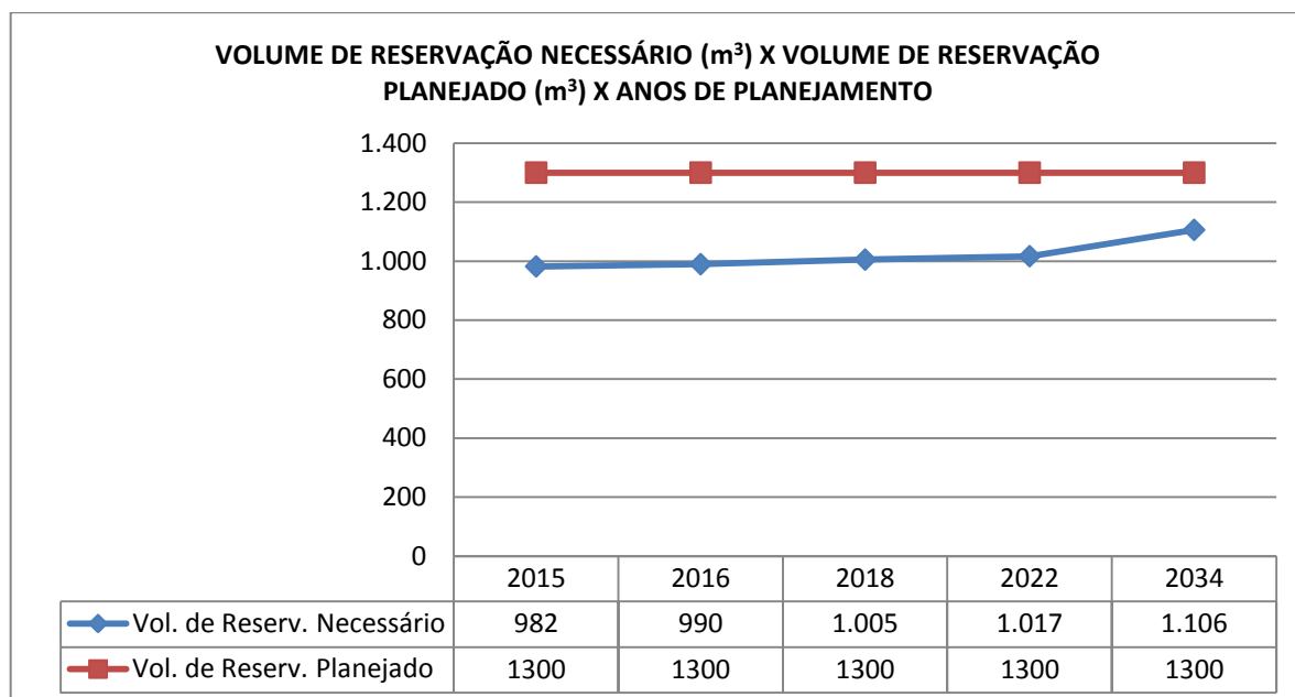
Gráfico 3.3 – Volumes de Reservação Necessários (m³) x Volume de Reservação Planejado (m³) x Anos de Planejamento
