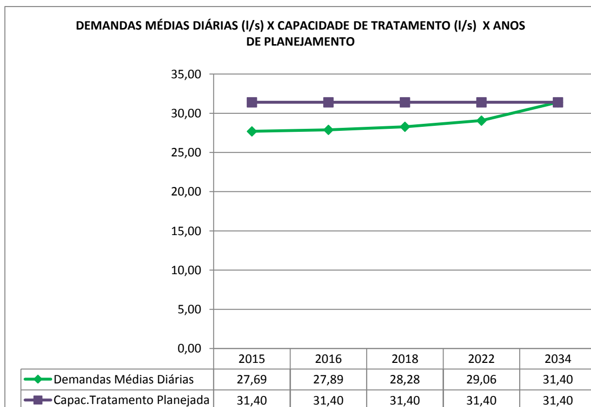
Gráfico 3.5 – Demandas Médias Diárias (l/s) x Capacidade de Tratamento (l/s) x Anos de Planejamento
