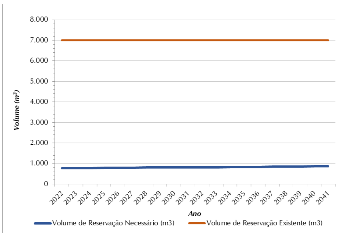
Figura 8.1 - Volume de Reservação Necessário (m³) x Volume de Reservação Atual (m³) – Setor de Abastecimento Morato Centro e Vila Santista
