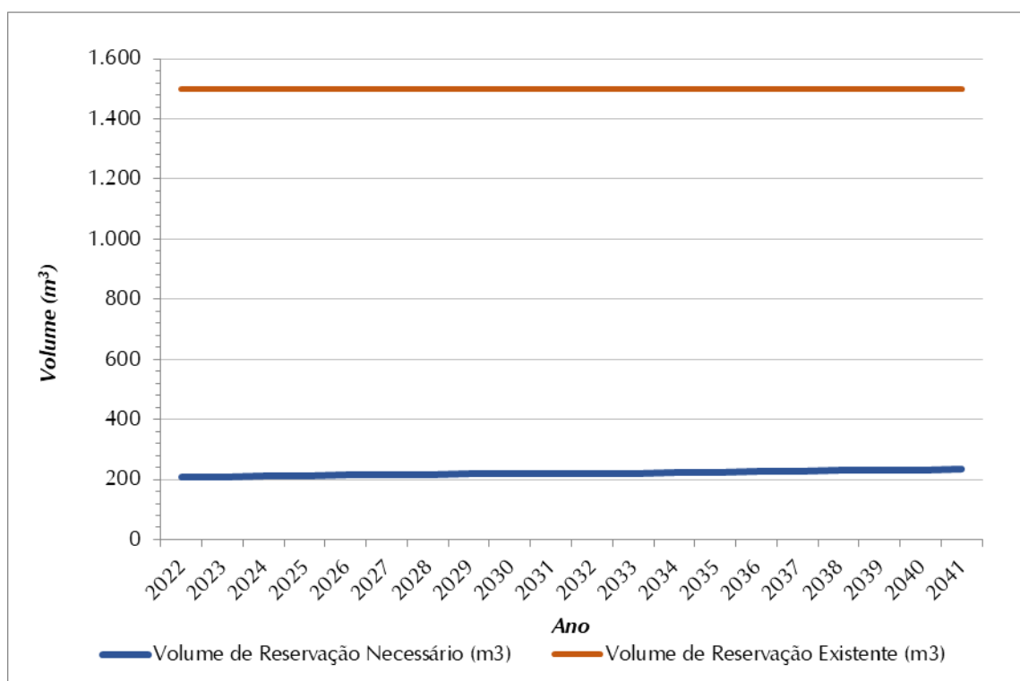
Figura 8.4 - Volume de Reservação Necessário (m³) x Volume de Reservação Atual (m³) – Setor de Abastecimento Jardim Arpoador
