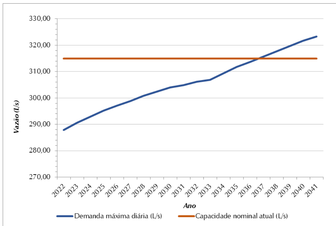
Figura 8.5 – Evolução da Demanda Máxima Diária (L/s) x Capacidade Nominal Atual (L/s) – EEAT Jardim Liliane
