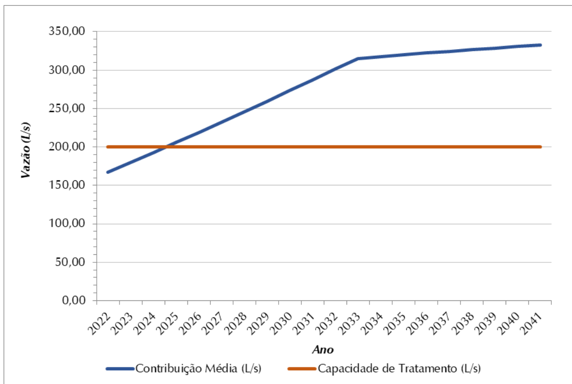
Figura 8.7 – Contribuição Média Total (L/s) x Capacidade de Tratamento de Esgoto (L/s) – SES ETE Vermelha
