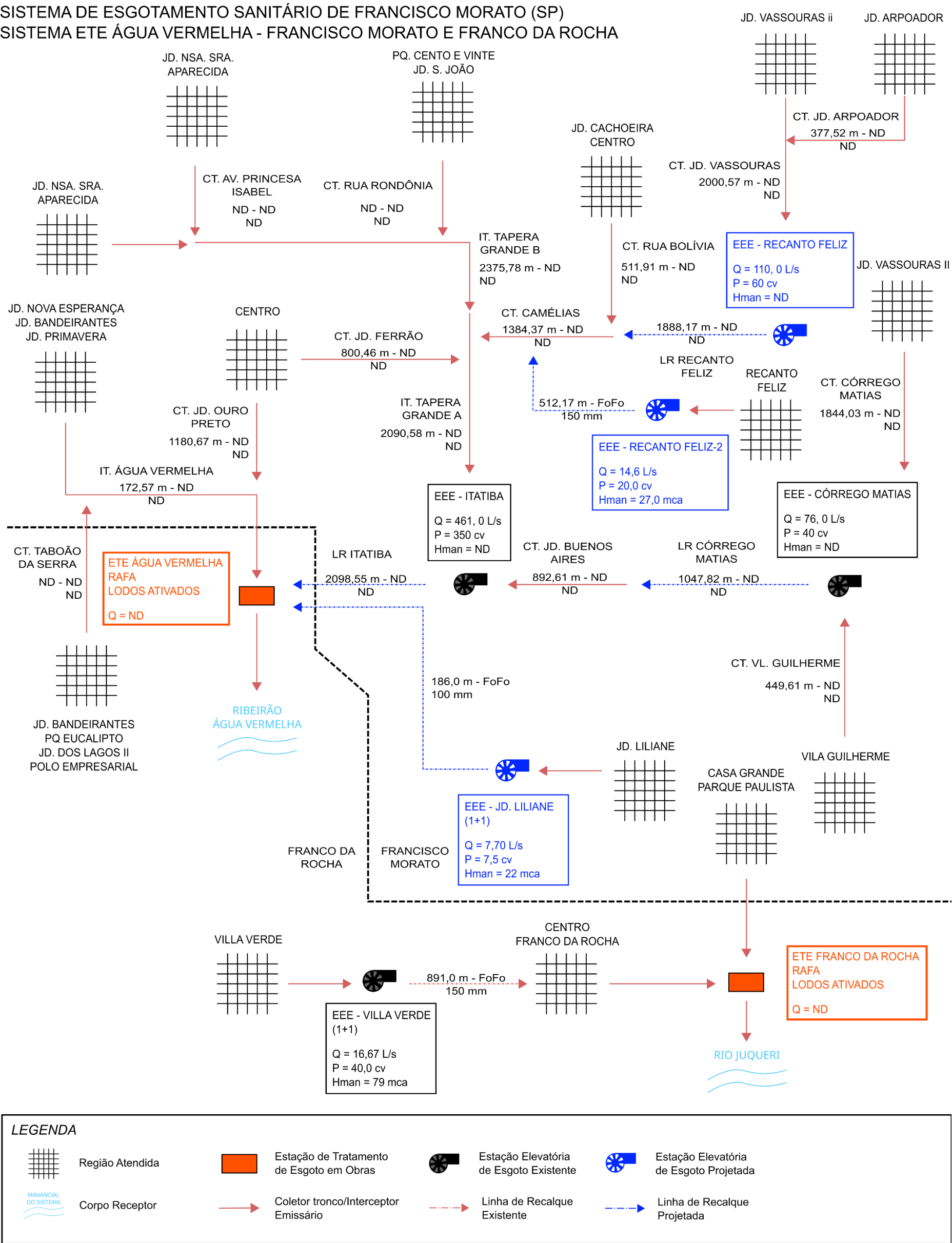
Figura 4.3 – Croqui do Sistema de Esgotamento Sanitário de Franco da Rocha e Francisco Morato. Fonte: SABESP, 2020.
