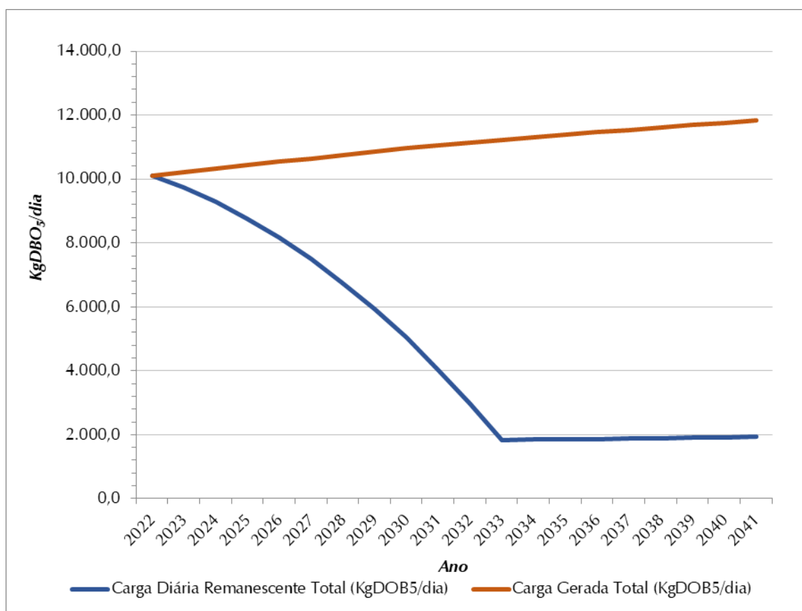
Figura 8.8 - Evolução de Cargas Orgânicas (Kg DBO 5,20 /Dia) – ETE Água Vermelha
