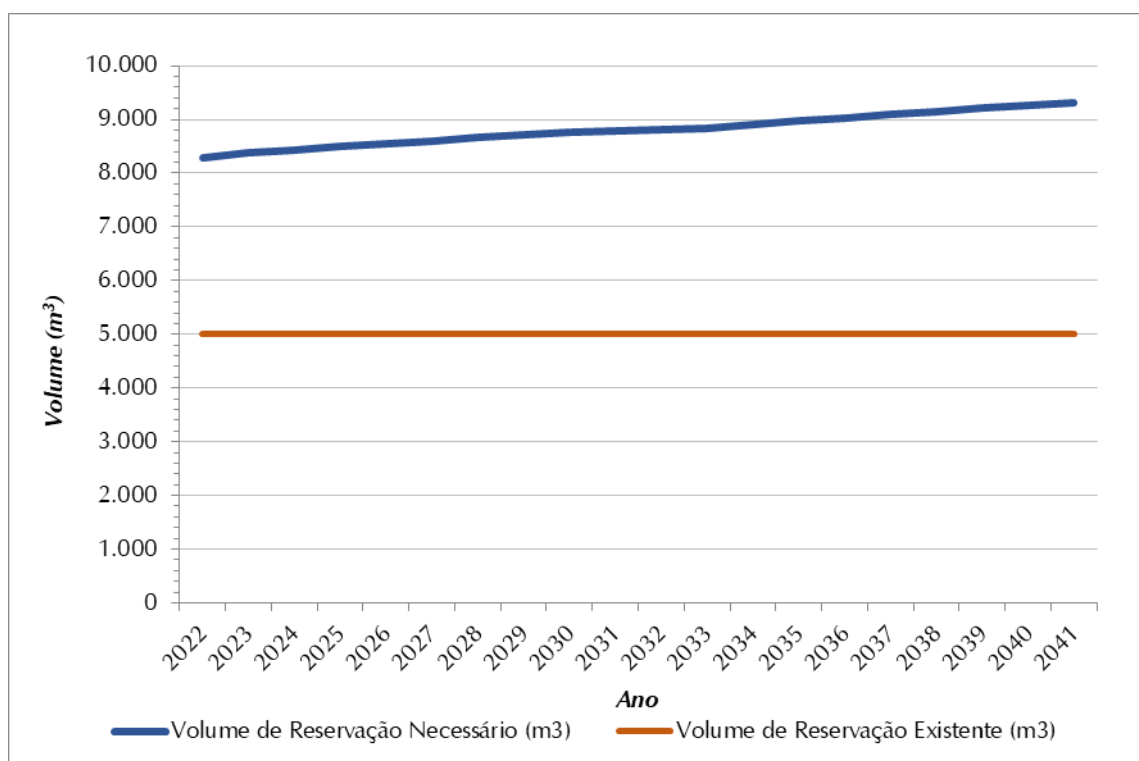
Figura 8.2 - Volume de Reservação Necessário (m³) x Volume de Reservação Atual (m³) – Setor de Abastecimento Jardim Liliane
