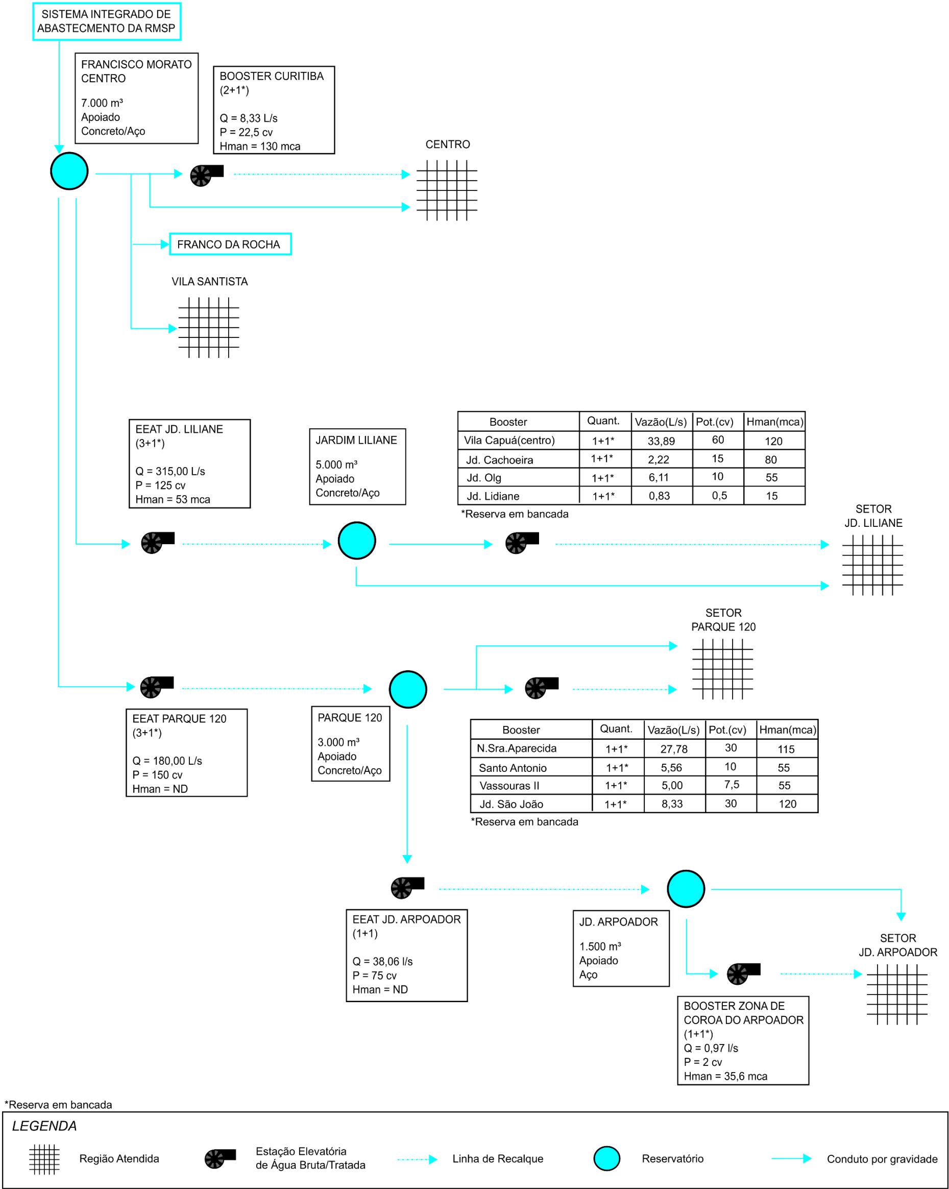
Figura 4.2 – Croqui do Sistema de Abastecimento de Água Sede
