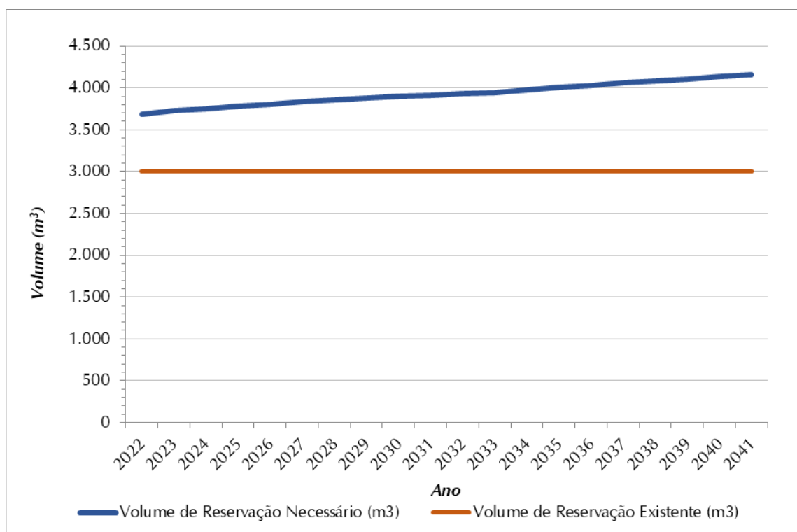
Figura 8.3 - Volume de Reservação Necessário (m³) x Volume de Reservação Atual (m³) – Setor de Abastecimento Parque 120
