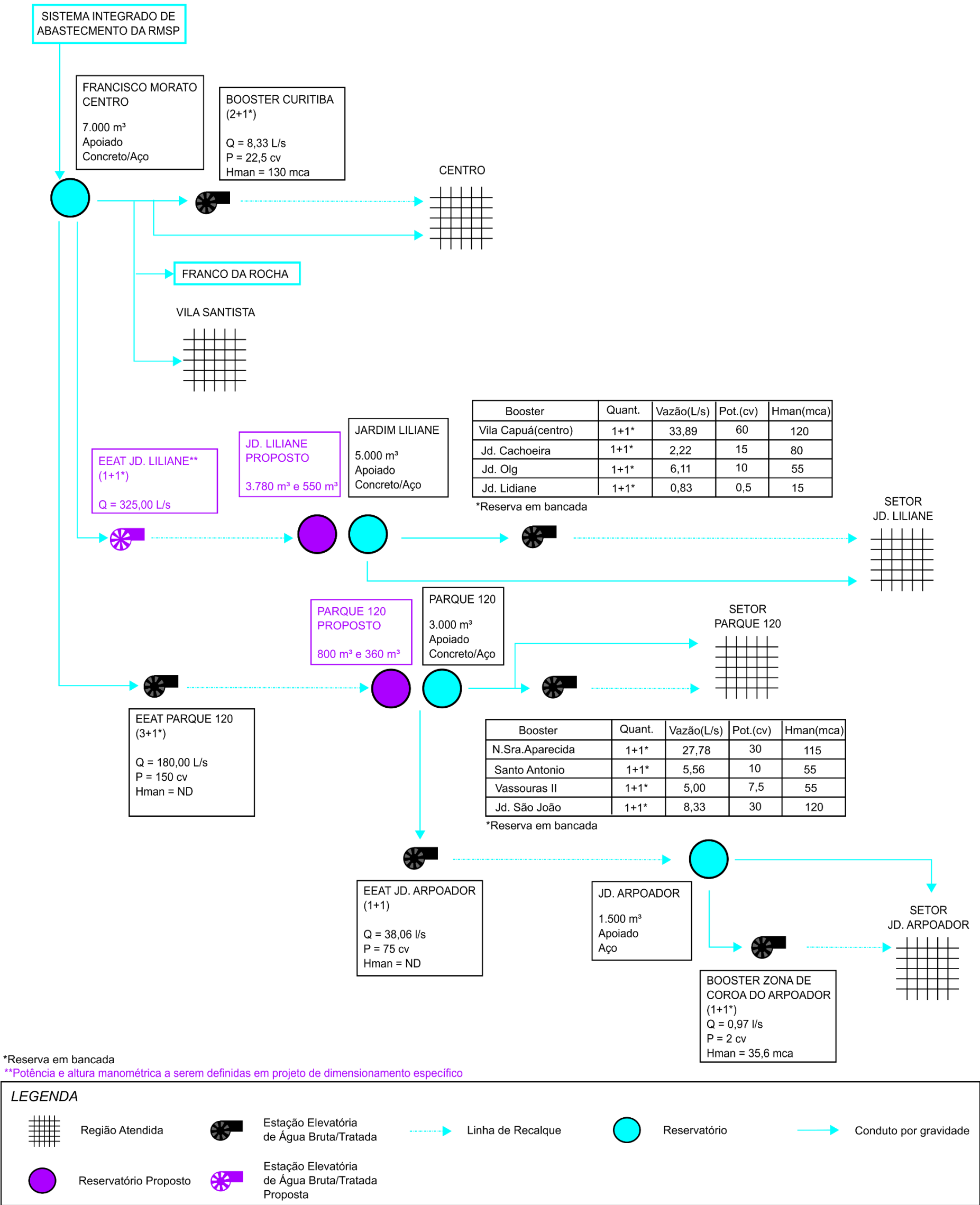
Figura 10.1 – Croqui das intervenções propostas para o sistema de abastecimento de água
