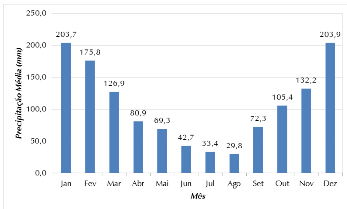
Figura 3.2 - Precipitação Média Mensal no Período de 1971 a 2021, Estação C7-078
