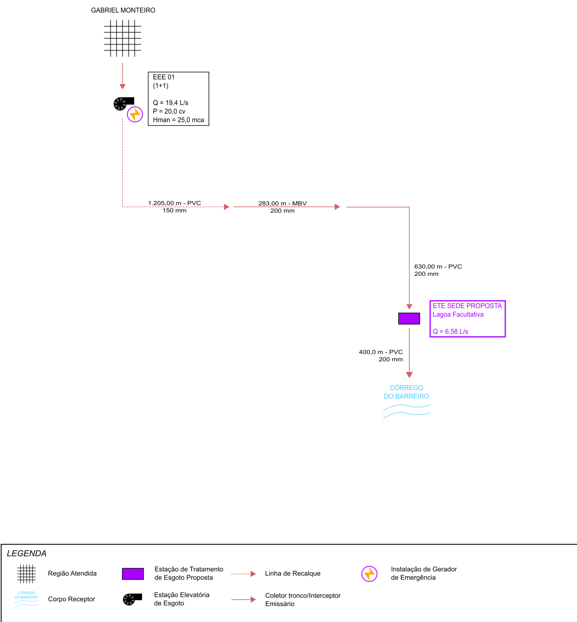
Figura 10.1 – Croqui das intervenções propostas no sistema de esgotamento sanitário Sede
