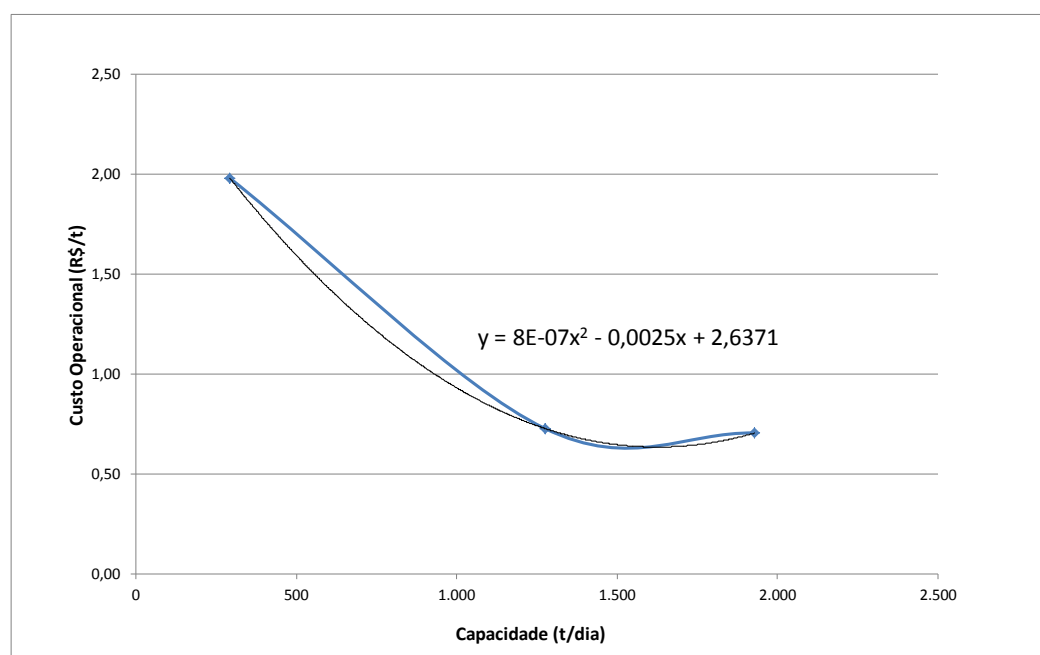
Gráfico 9.7 – Variação do custo operacional do ARCC em função da capacidade
