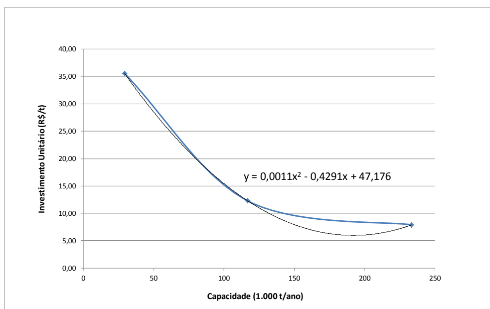
Gráfico 9.4 – Variação do custo de implantação da CB em função da capacidade
