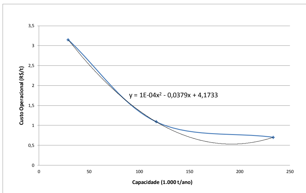
Gráfico 9.5 – Variação do custo operacional da CB em função da capacidade
