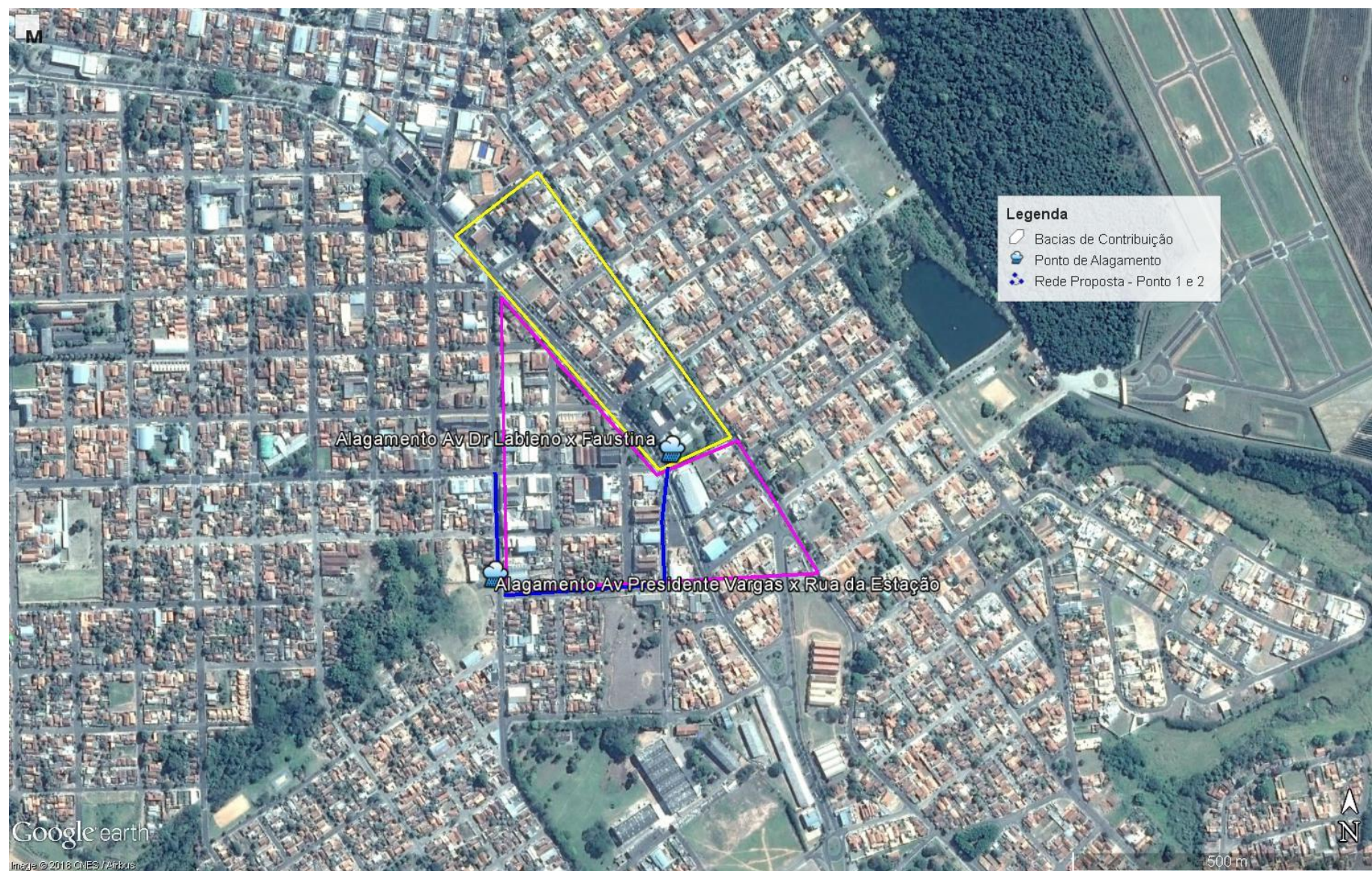
Ilustração 8.1 – Intervenções Propostas para os Pontos 1 e 2
