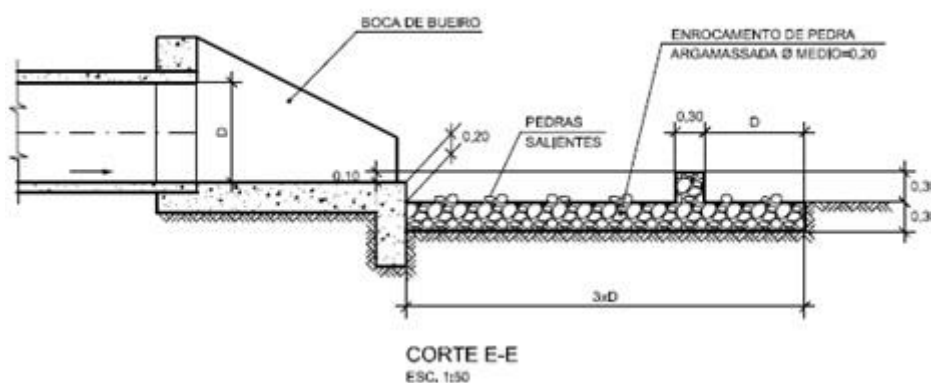
Ilustração 8.5 – Dissipador de Energia a ser Utilizado
