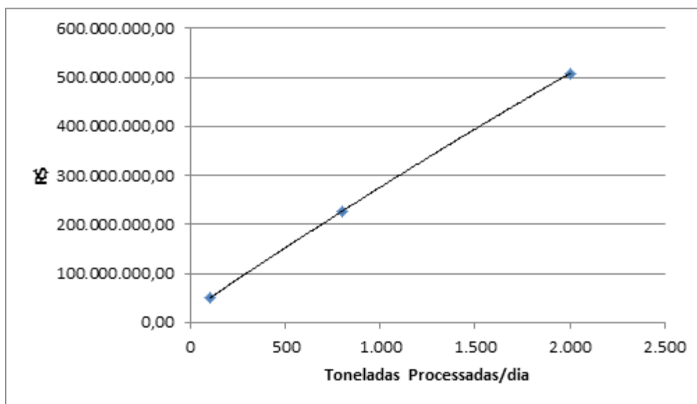
Gráfico 9.3 – Variação do custo de implantação do ATS em função da quantidade de resíduos processados por dia
