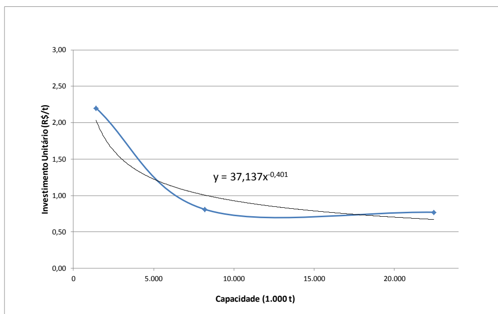
Gráfico 9.6 – Variação do custo da implantação do ARCC em função da capacidade
