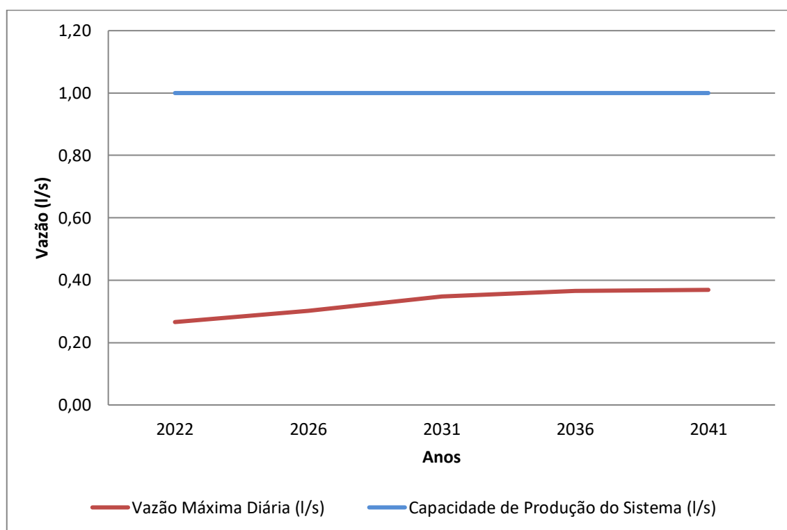
Gráfico 8.11 – Demandas Máximas Diárias (l/s) X Capacidade de Produção do Sistema (l/s)
