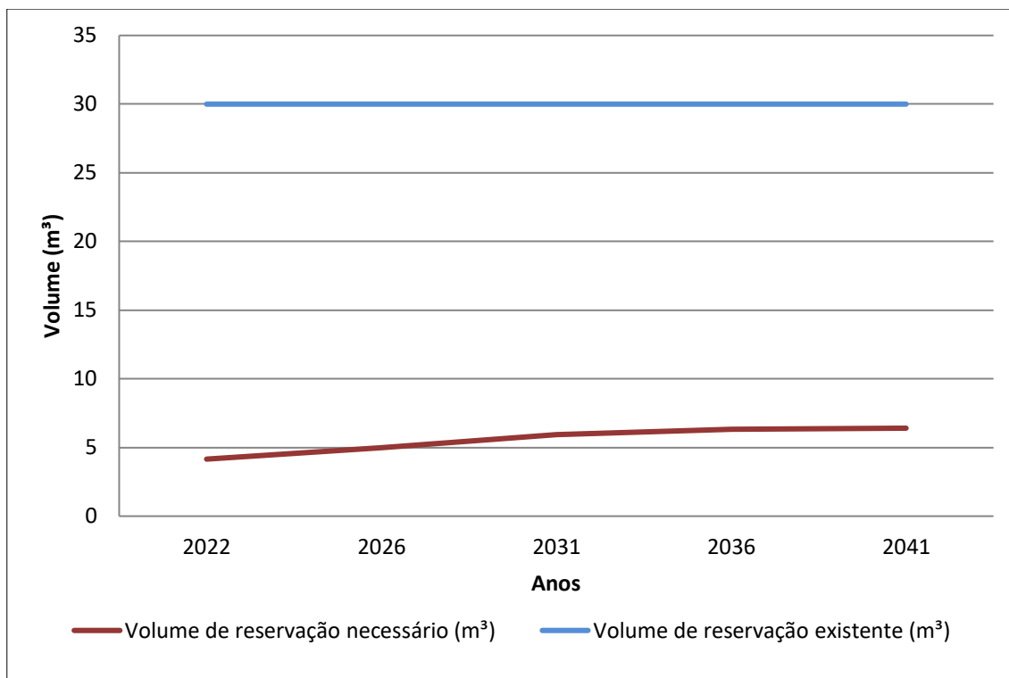
Gráfico 8.15 - Volume de Reservação Necessário (m³) x Volume de Reservação Atual (m³)
