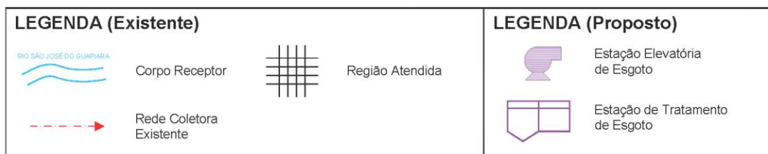
Figura 10.6 – Croqui do Sistema de Esgotamento Sanitário Proposto para Sede Urbana
