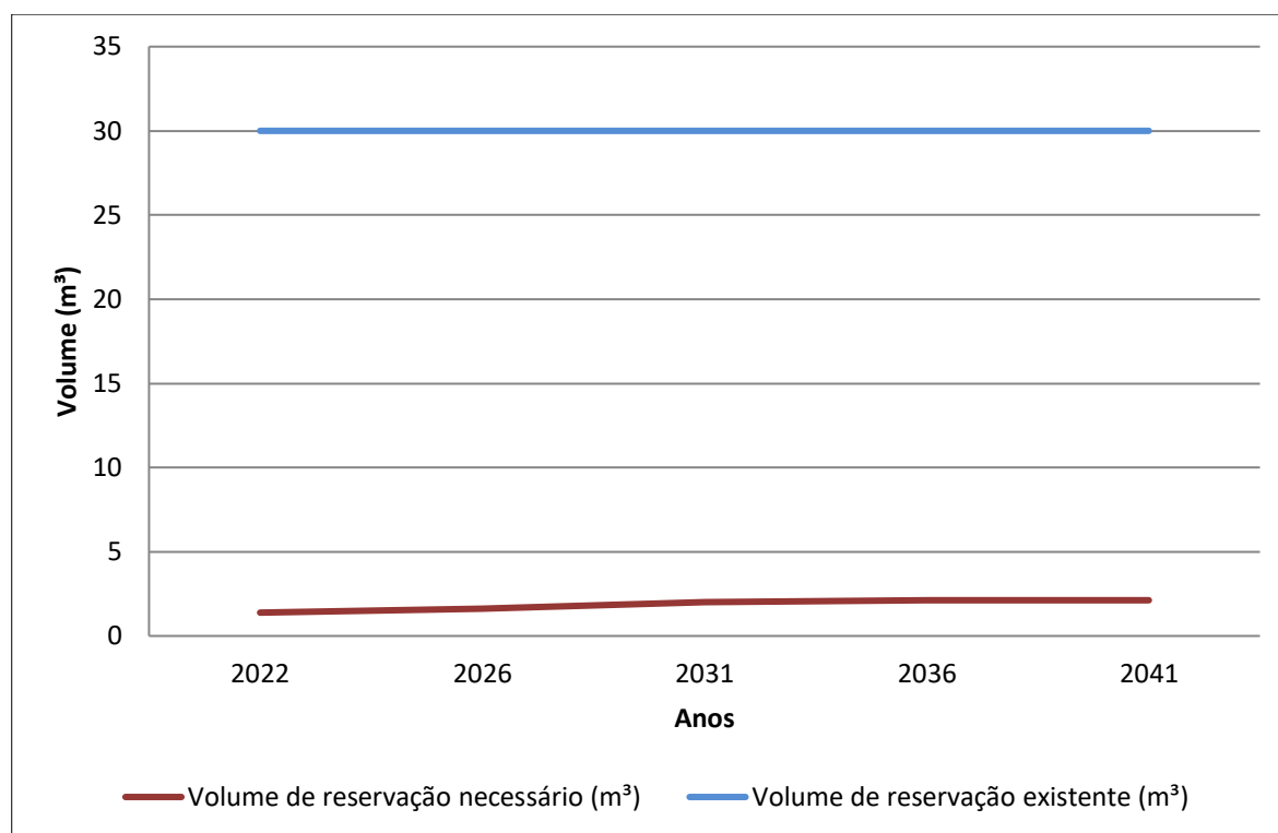
Gráfico 8.9 - Volume de Reservação Necessário (m³) x Volume de Reservação Atual (m³)
