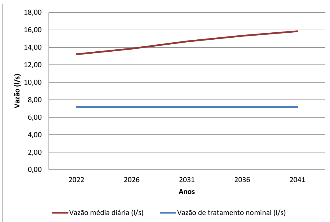
Gráfico 8.16 – Vazão Média Diária (l/s) x Capacidade nominal da ETE (l/s)
