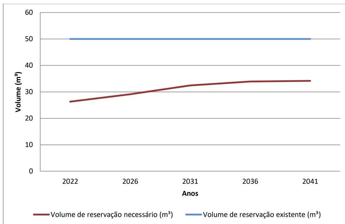
Gráfico 8.10 - Volume de Reservação Necessário (m³) x Volume de Reservação Atual (m³)
