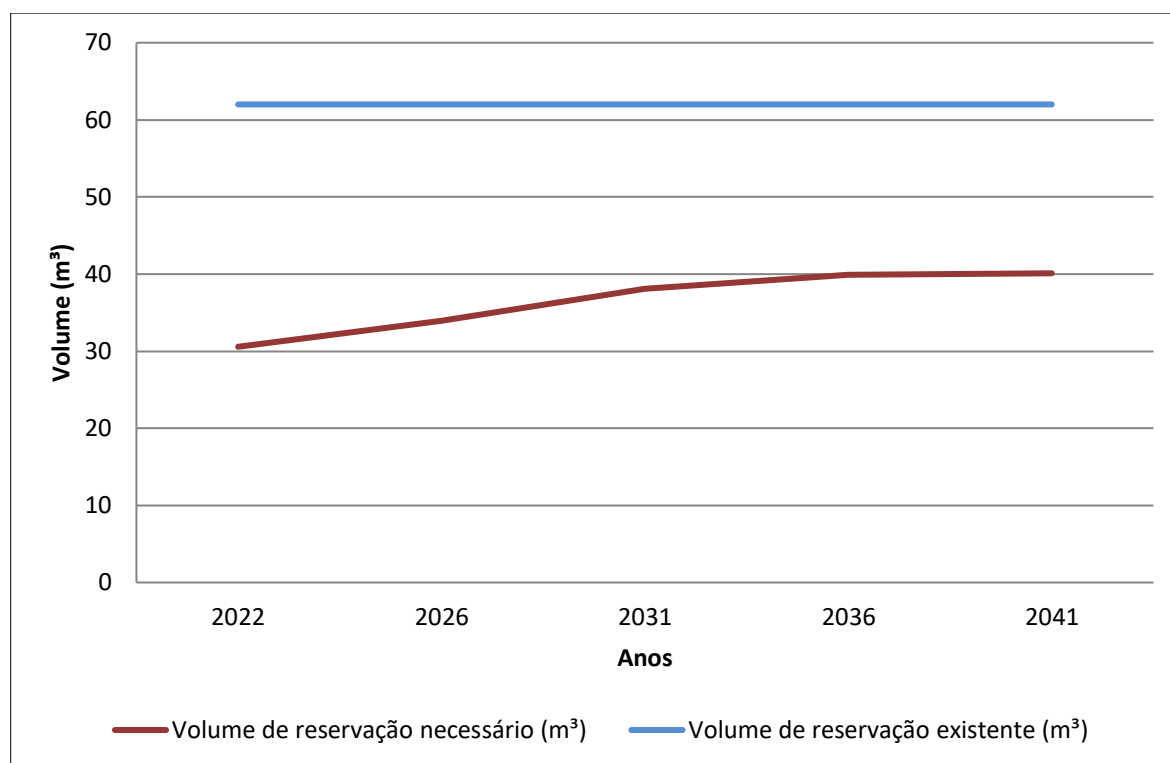
Gráfico 8.14 - Volume de Reservação Necessário (m³) x Volume de Reservação Atual (m³)
