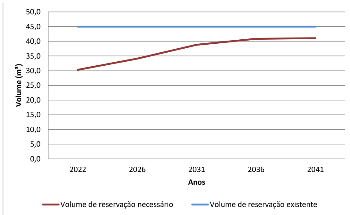
Gráfico 8.8 - Volume de Reservação Necessário (m³) x Volume de Reservação Atual (m³)
