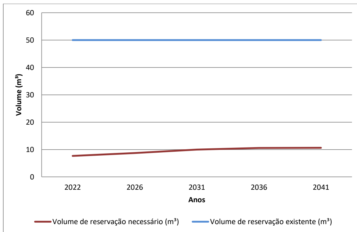
Gráfico 8.12 - Volume de Reservação Necessário (m³) x Volume de Reservação Atual (m³)
