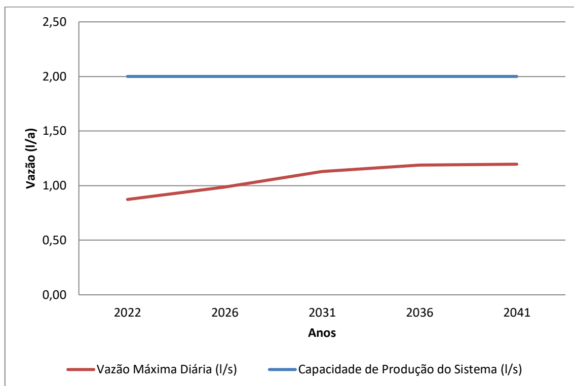
Gráfico 8.6 – Demandas Máximas Diárias (l/s) X Capacidade de Produção do Sistema (l/s)
