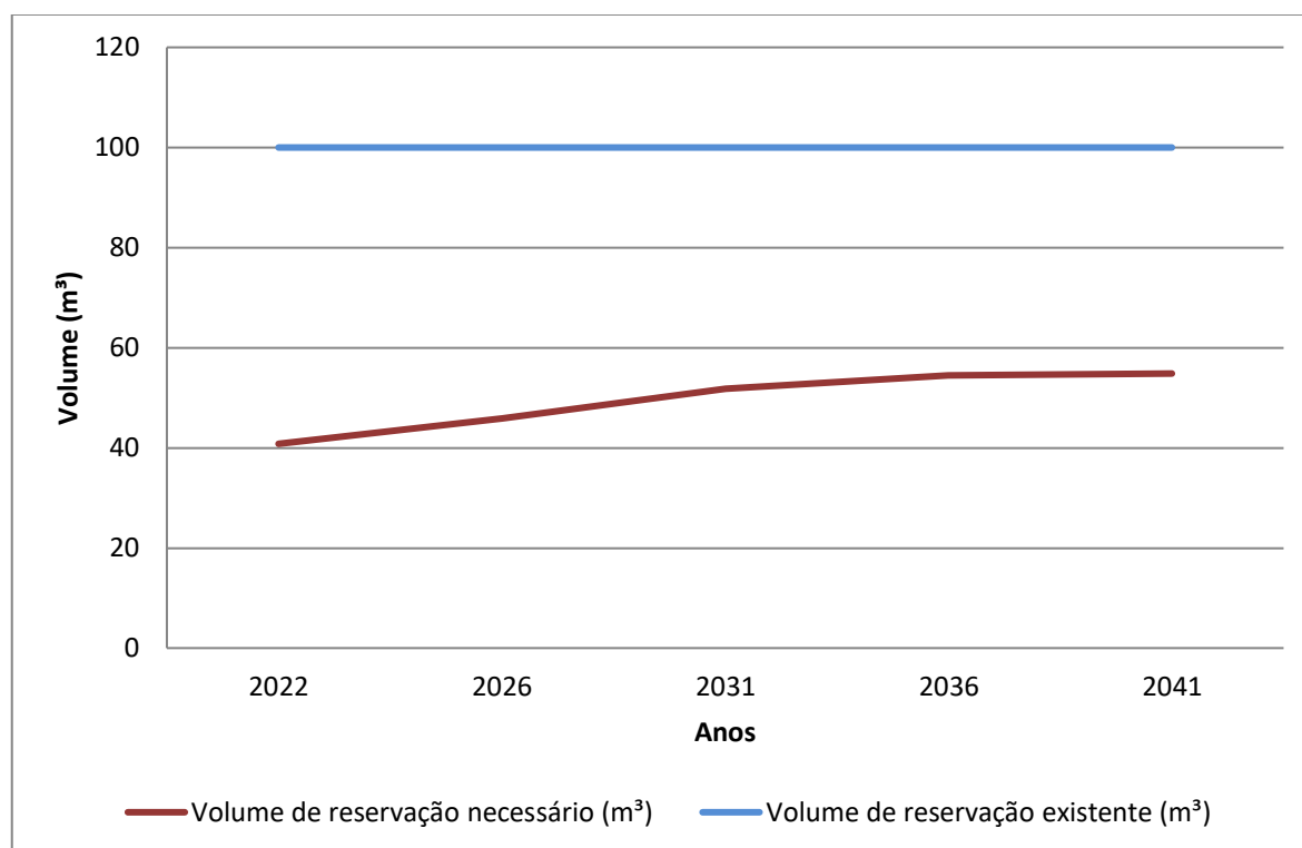
Gráfico 8.13 - Volume de Reservação Necessário (m³) x Volume de Reservação Atual (m³)
