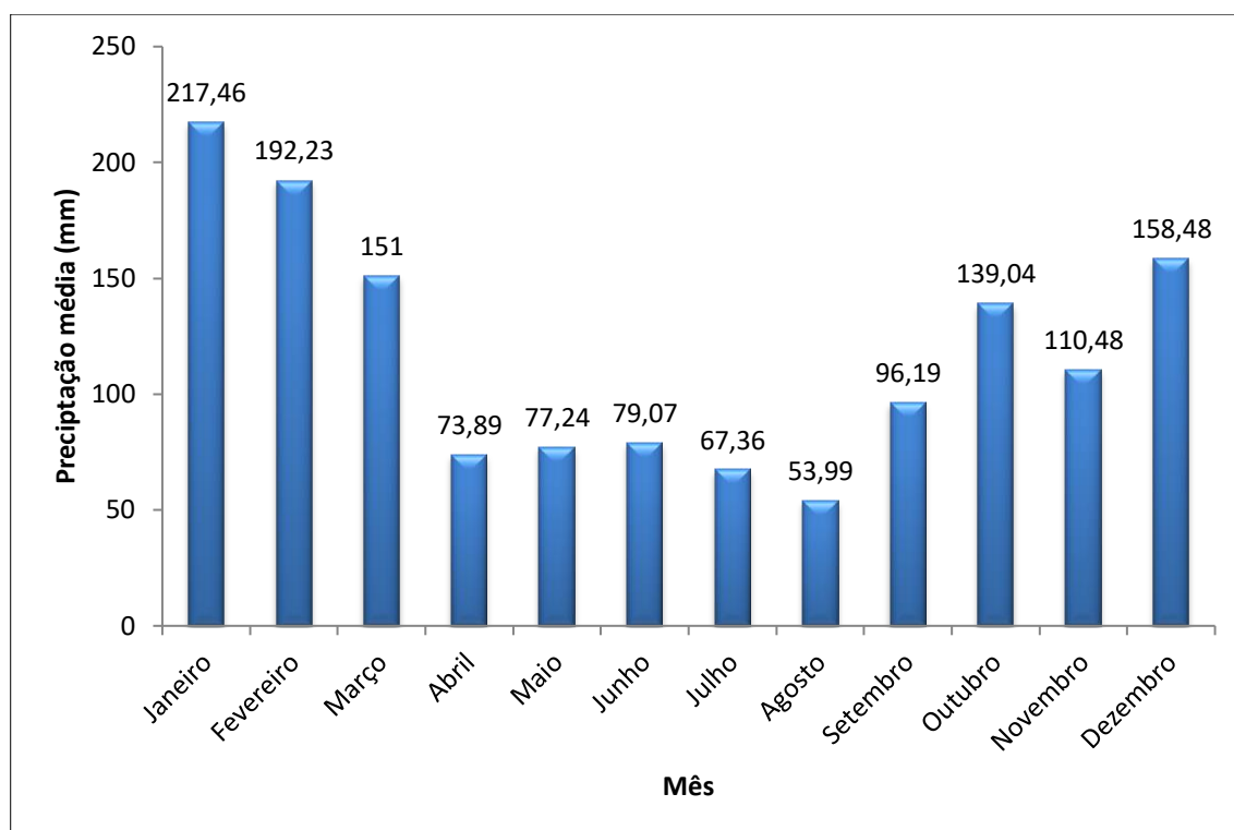
Gráfico 3.1 – Precipitação Média Mensal no Período de 1939 a 1998, Estação F5-010
