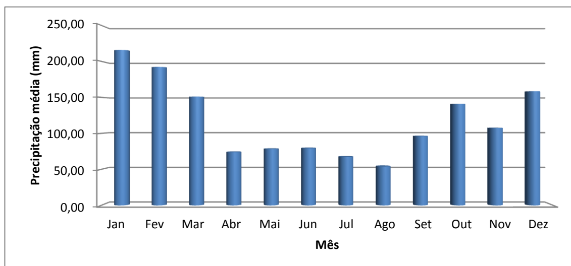
Gráfico 2.1 – Precipitação média mensal no período de 1939 a 1998 – Estação F5-010.
