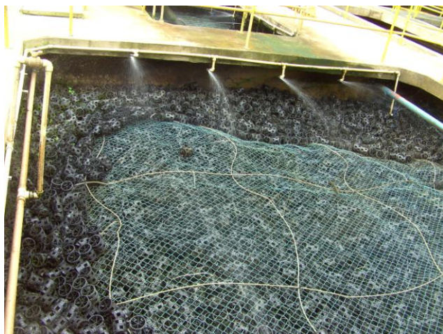
FOTO 4.22 – ETE SEDE – TANQUES AERÓBIOS
