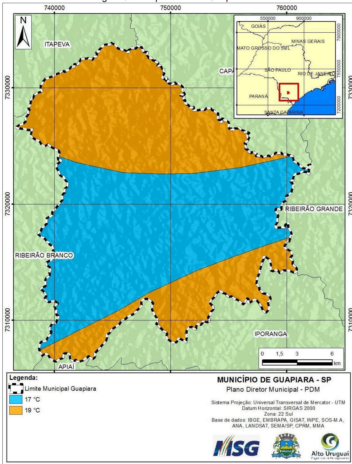
Figura 9 - Temperatura em Guapiara.
