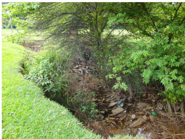
Foto 3.12 - Erosão causada pela falta de dissipador de energia no lançamento.
