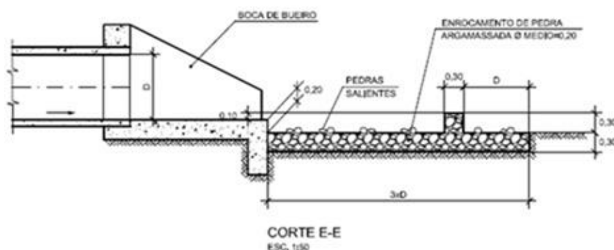
Ilustração 8.2 – Dissipador.
