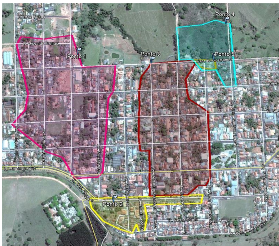
Figura 4.1 - Pontos críticos do sistema de microdrenagem
