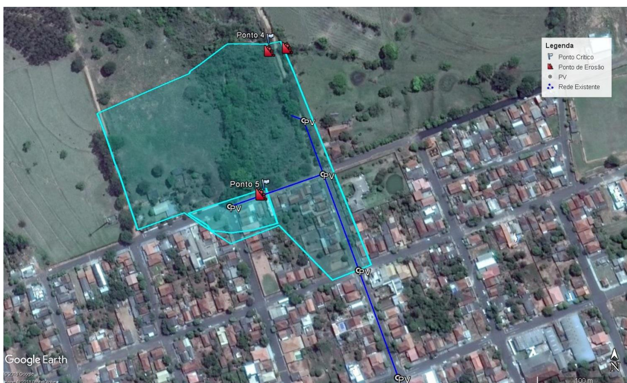
Ilustração 8.3 – Intervenções Propostas para os Pontos 4 e 5
