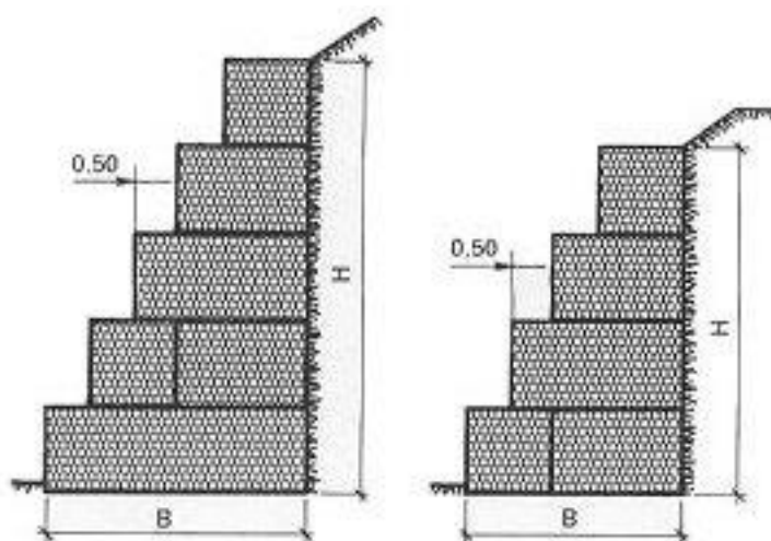
Ilustração 8.5 –Contenção de taludes com gabião tipo caixa.
