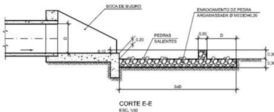
Ilustração 8.4 –Dissipador de energia.
