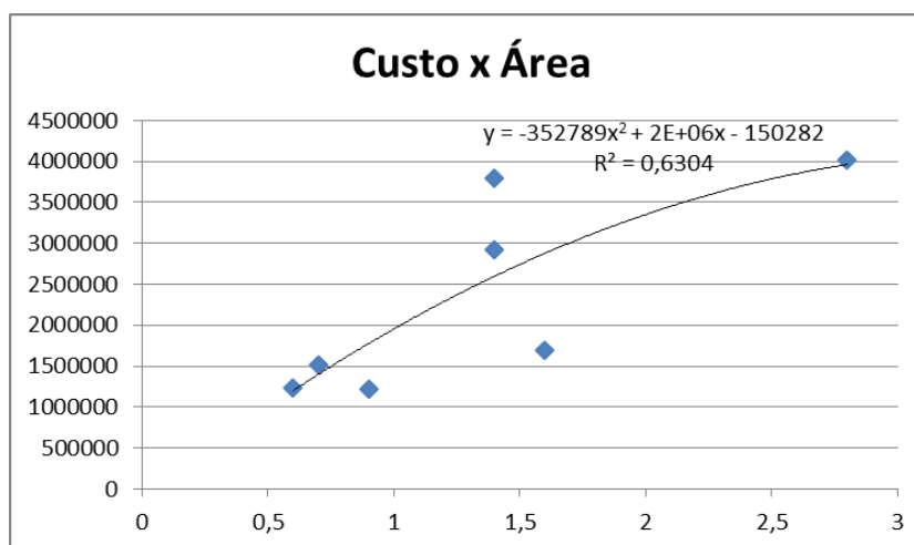
Gráfico 9.1 – Curva paramétrica de investimento por área no sistema de drenagem
