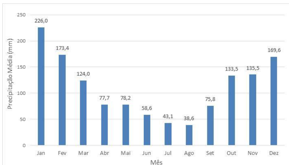
Gráfico 2.1 - Precipitação Média Mensal no Período de 1950 a 2016, Estação D8-047
