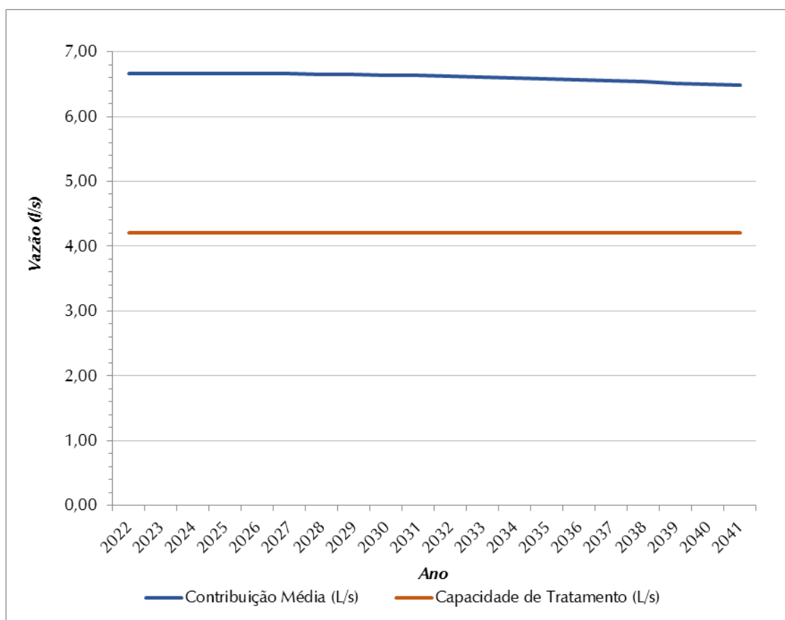
Figura 8.5 – Contribuição Média Total (L/s) x Capacidade de Tratamento de Esgoto (L/s) – SES Sede – ETE.1
