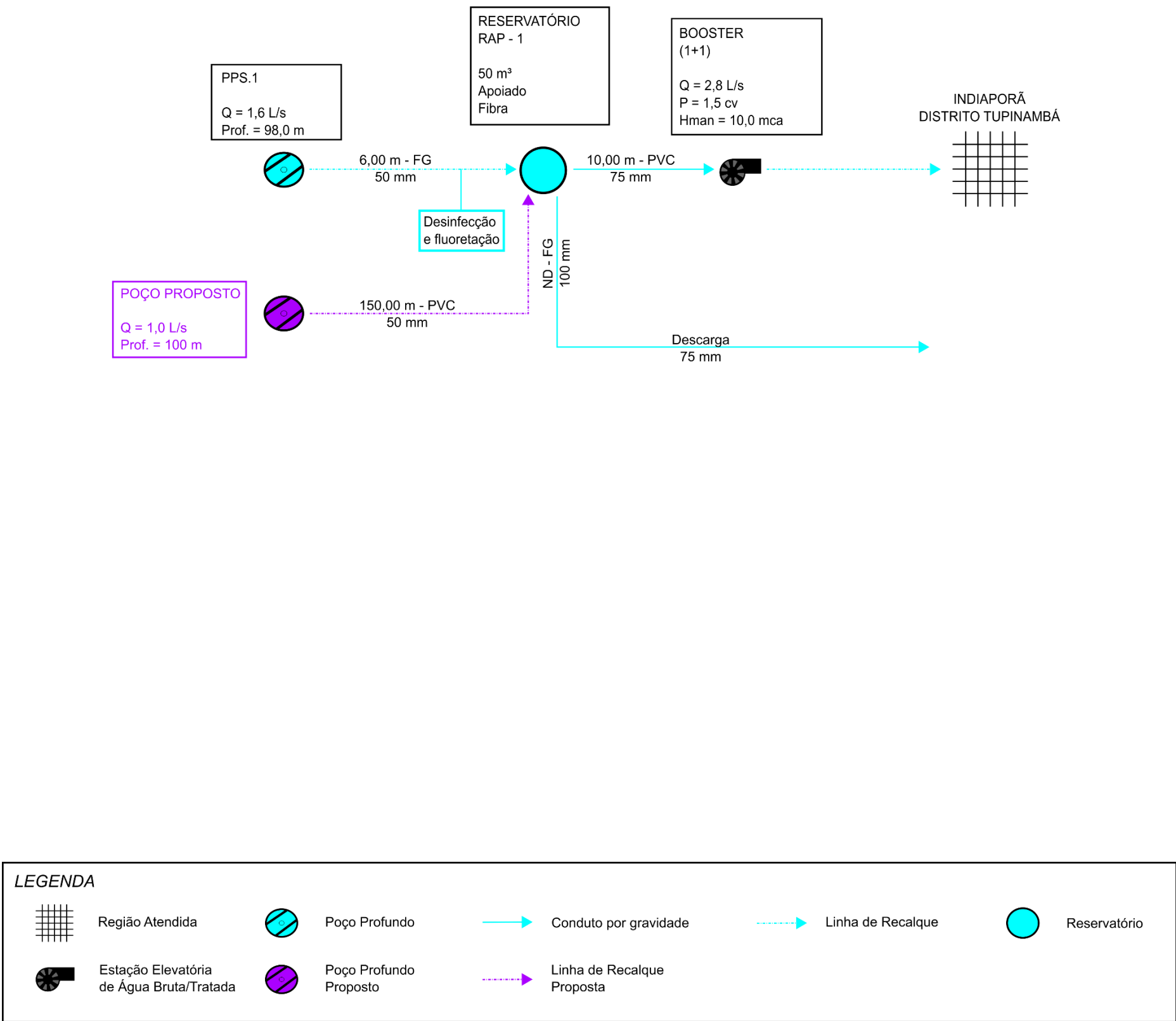
Figura 10.2 – Croqui das intervenções propostas para o sistema de abastecimento de água do Distrito Tupinambá.
