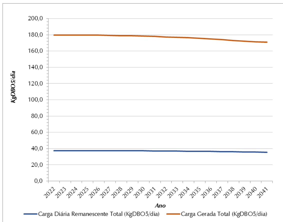
Figura 8.7 - Evolução de Cargas Orgânicas (Kg DBO 5,20 /Dia)
