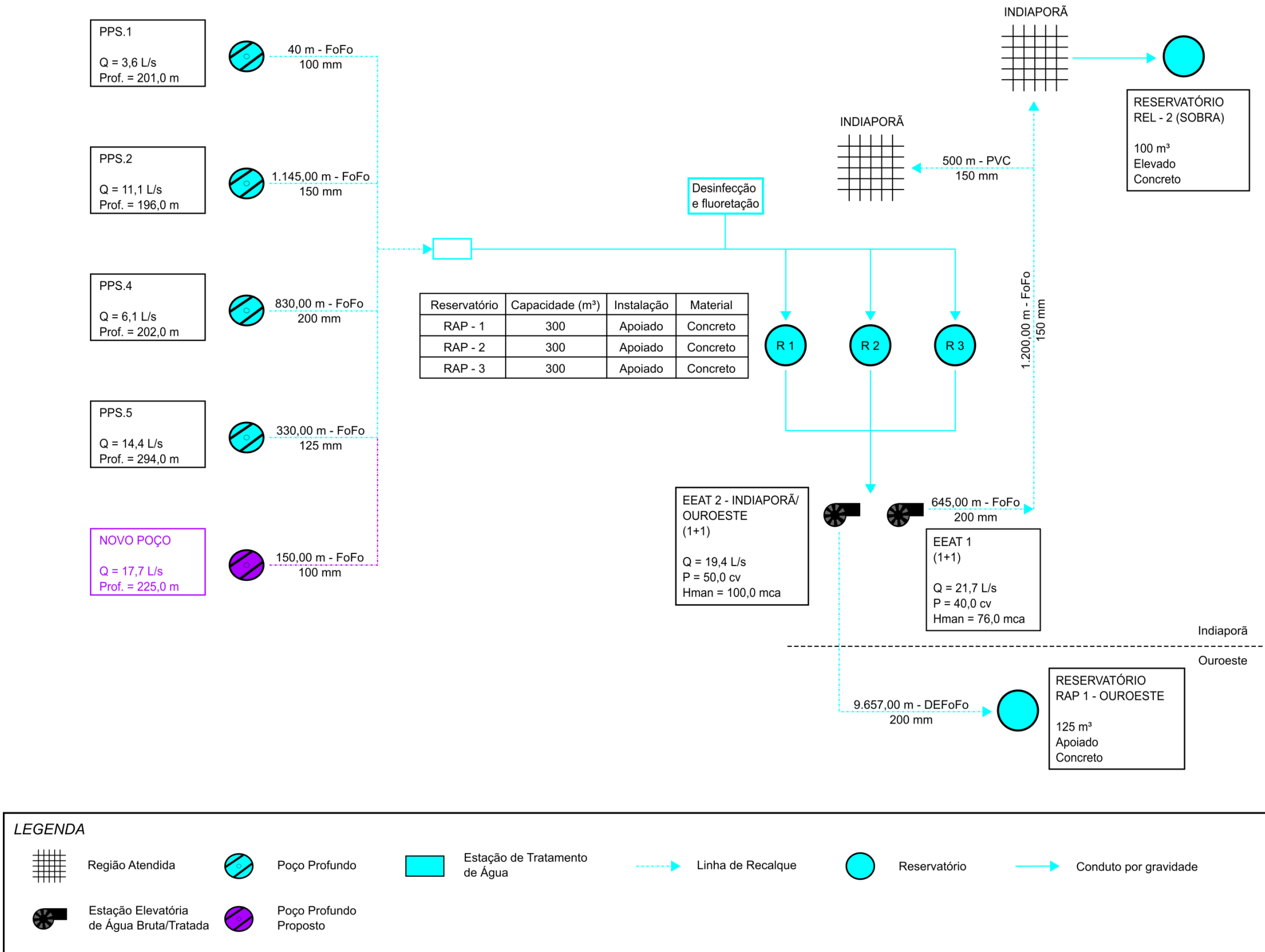
Figura 10.1 – Croqui das intervenções propostas para o sistema de abastecimento de água Sede
