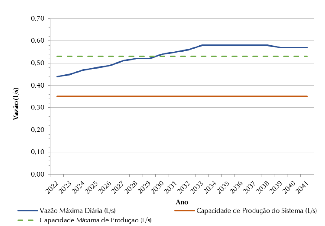
Figura 8.3 – Demandas Máximas Diárias (L/s) X Vazão Captada (L/s) – SAA Distrito Tupinambá
