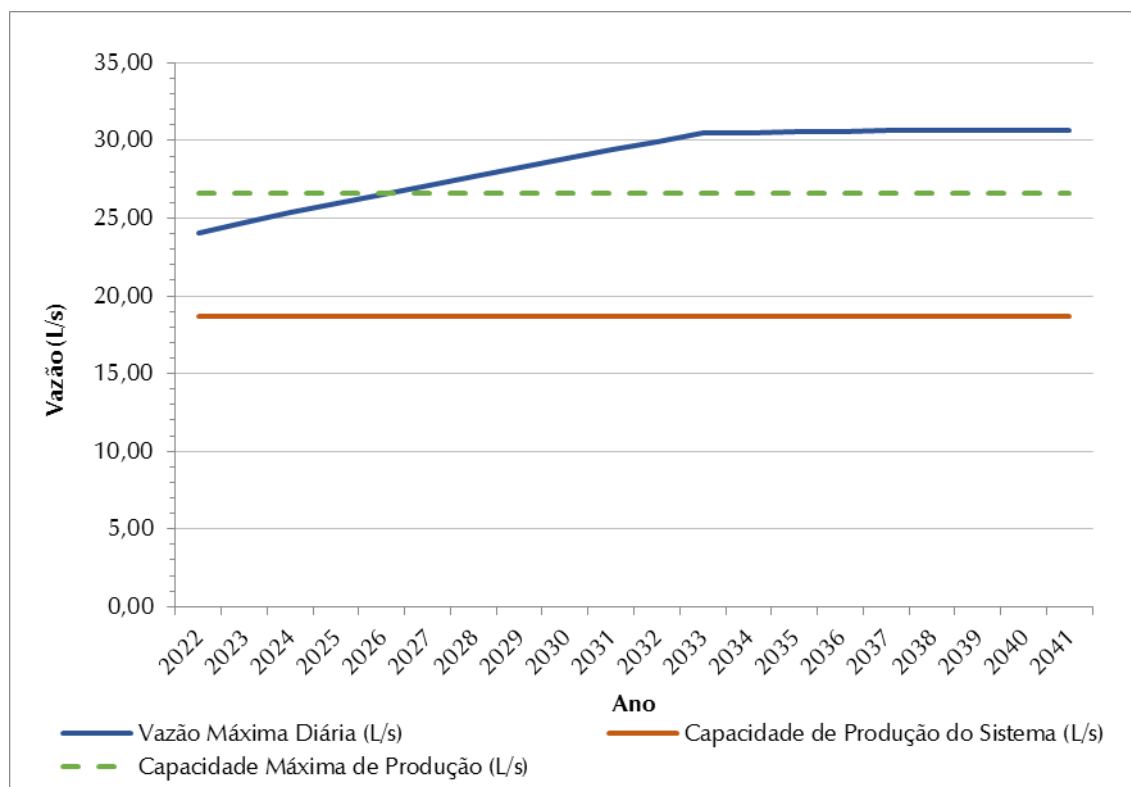
Figura 8.1 – Demandas Máximas Diárias (L/s) X Vazão Captada (L/s) – SAA Sede
