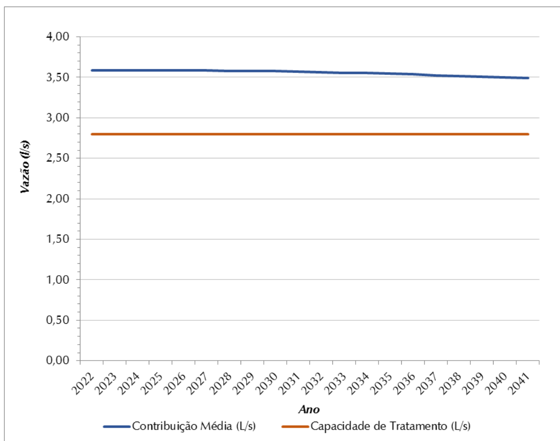
Figura 8.6 – Contribuição Média Total (L/s) x Capacidade de Tratamento de Esgoto (L/s) – SES Sede – ETE.2
