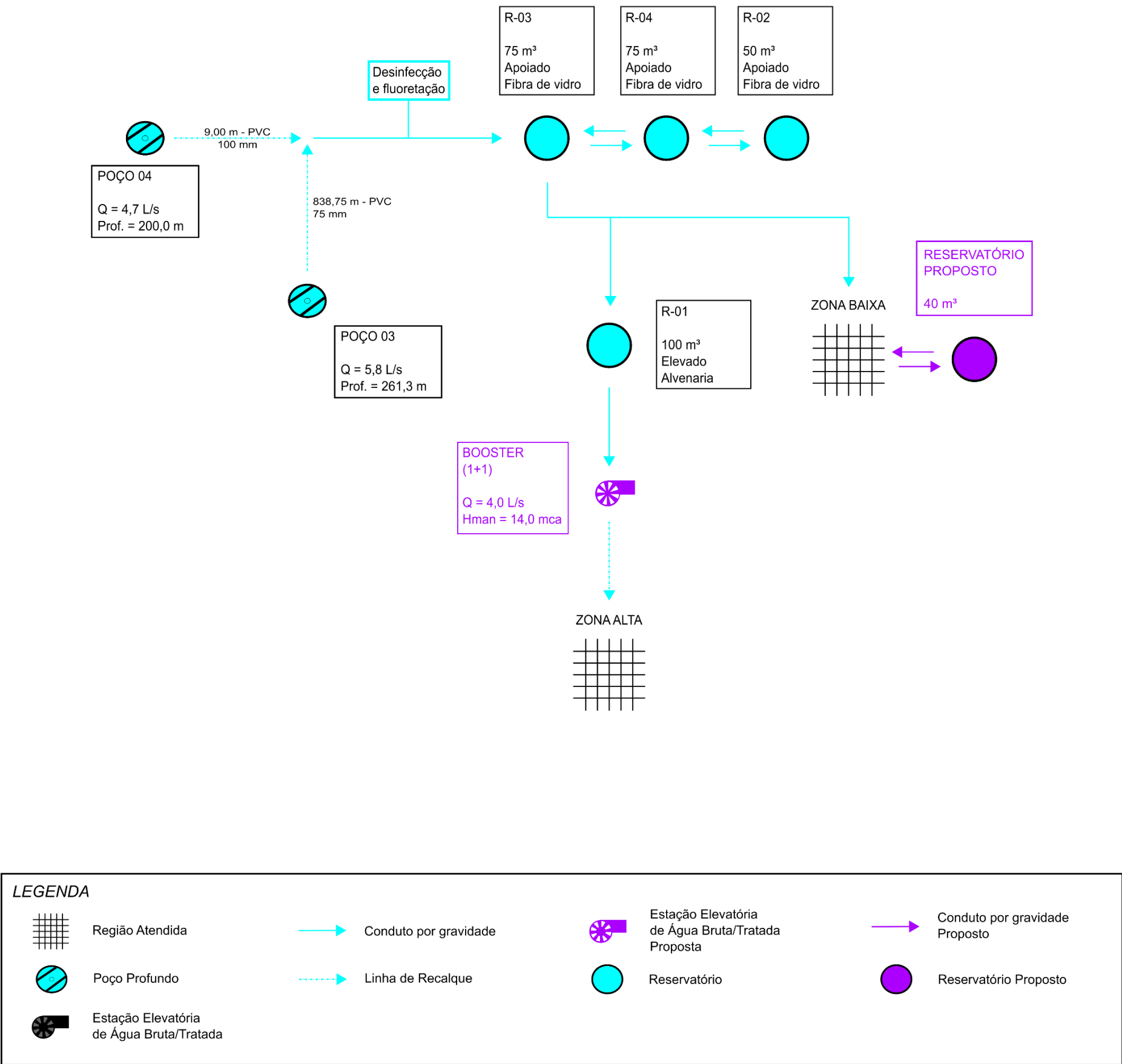
Figura 10.1 – Croqui das intervenções propostas para o sistema de abastecimento de água Sede
