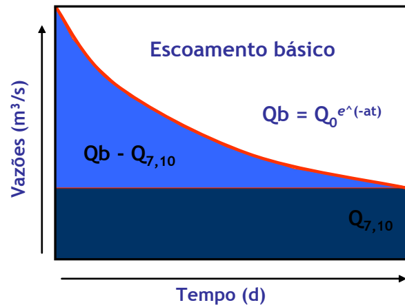
Figura 4.1 - Representação Esquemática da Hidrógrafa de Escoamento Básico, com Separação das Vazões Mínimas ( Q_{7,10} ) e Reservas Ativas ( Q_b - Q_{7,10} )
