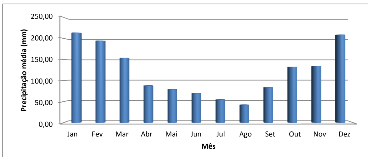
Gráfico 2.1 – Precipitação média mensal no período de 1941 a 2004 – Estação E6-007.
