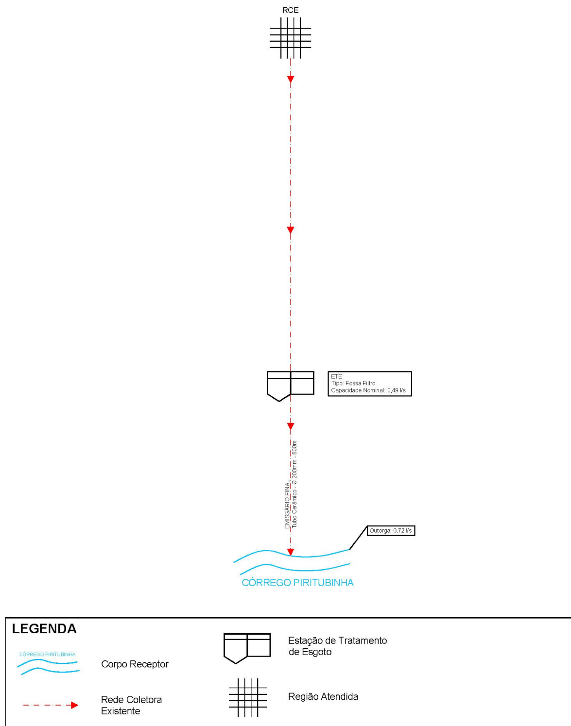
Figura 4.7 – Croqui do Sistema de Esgotamento Sanitário Existente – Bairro Engenheiro Maia
