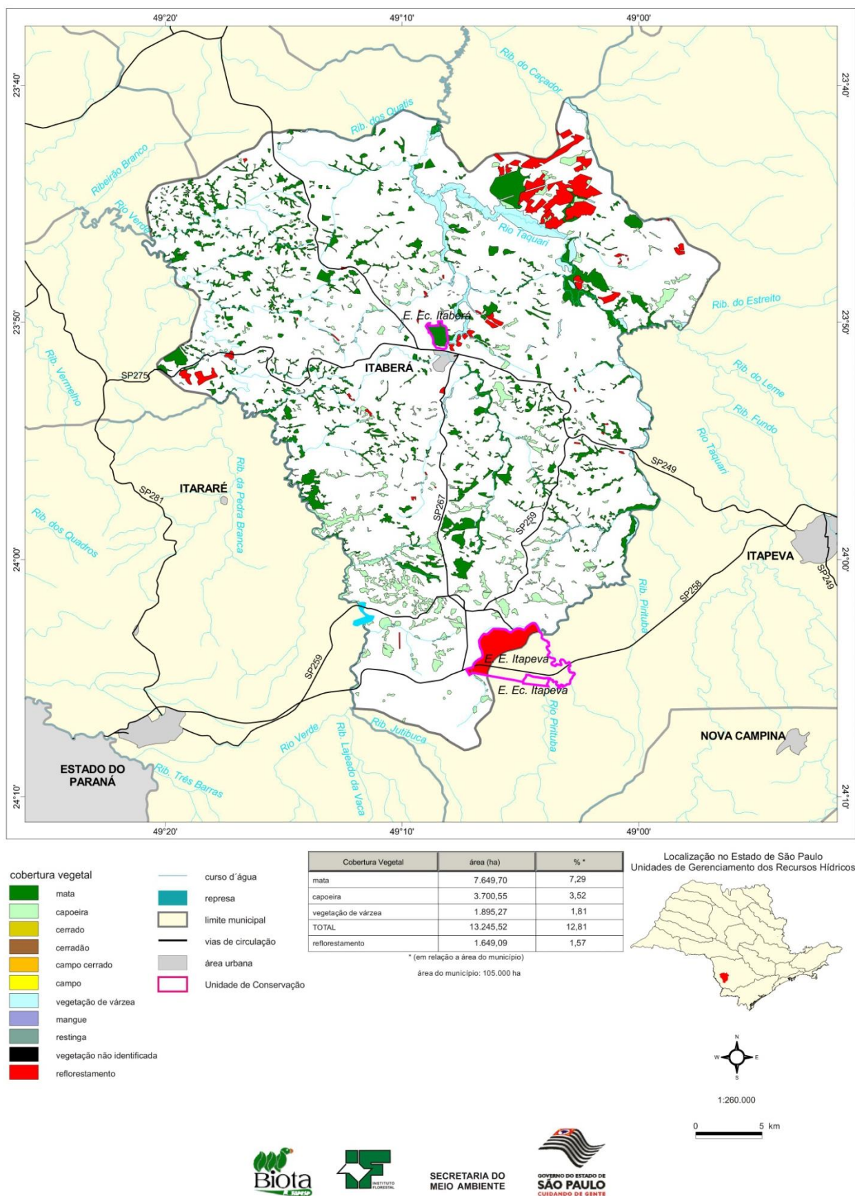
Figura 3.2 – Cobertura Vegetal no Município de Itaberá
