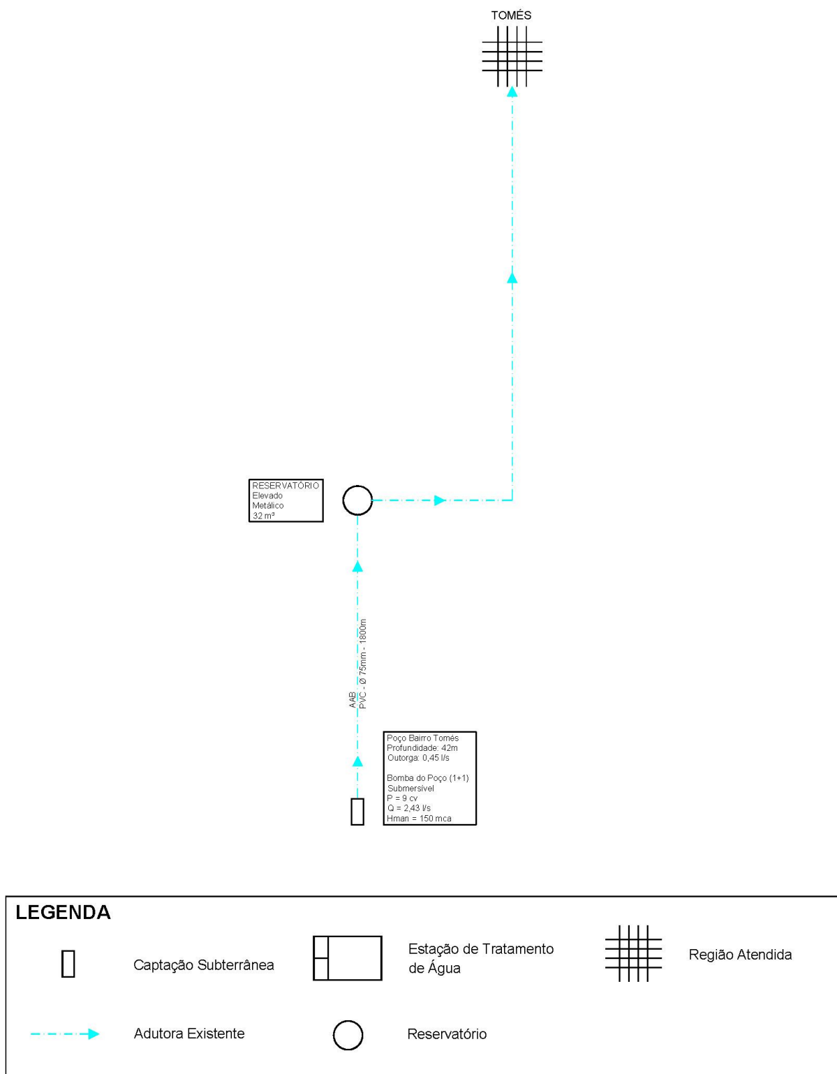
Figura 4.3 – Croqui do Sistema de Abastecimento de Água Existente – Bairro Tomés.
