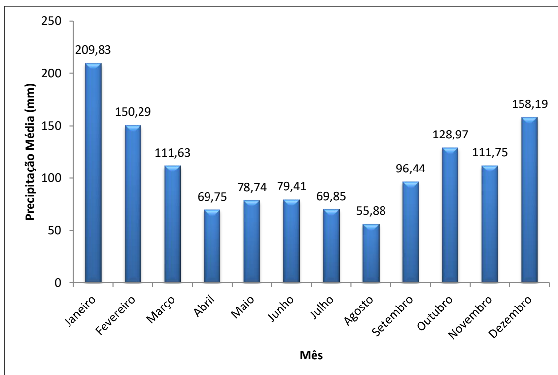
Gráfico 3.1 – Precipitação Média Mensal no Período de 1939 a 2021, Estação F6-003
