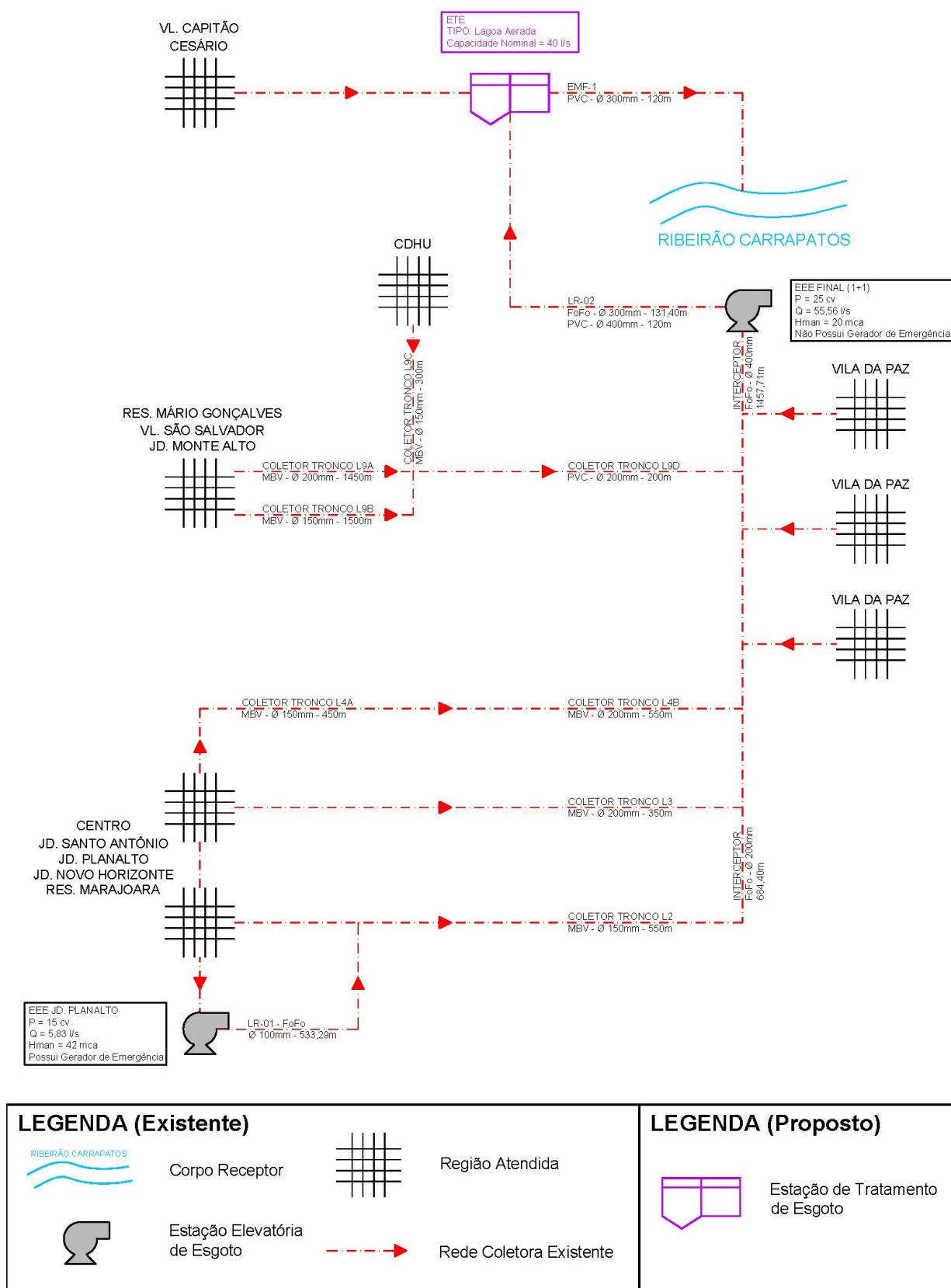
Figura 10.2 – Croqui do Sistema de Esgotamento Sanitário Proposto para o Subsistema da Sede Urbana
