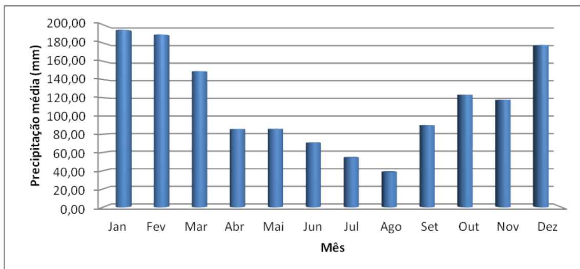
Gráfico 2.1 – Precipitação média mensal no período de 1971 a 2000 – Estação E6-034.
