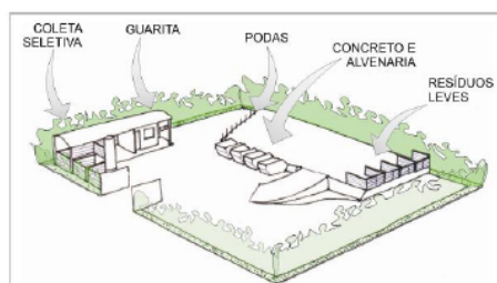
Figuras 14 – Esquema de Posto de Entrega Voluntária para RCC, podas, resíduos leves e recicláveis
