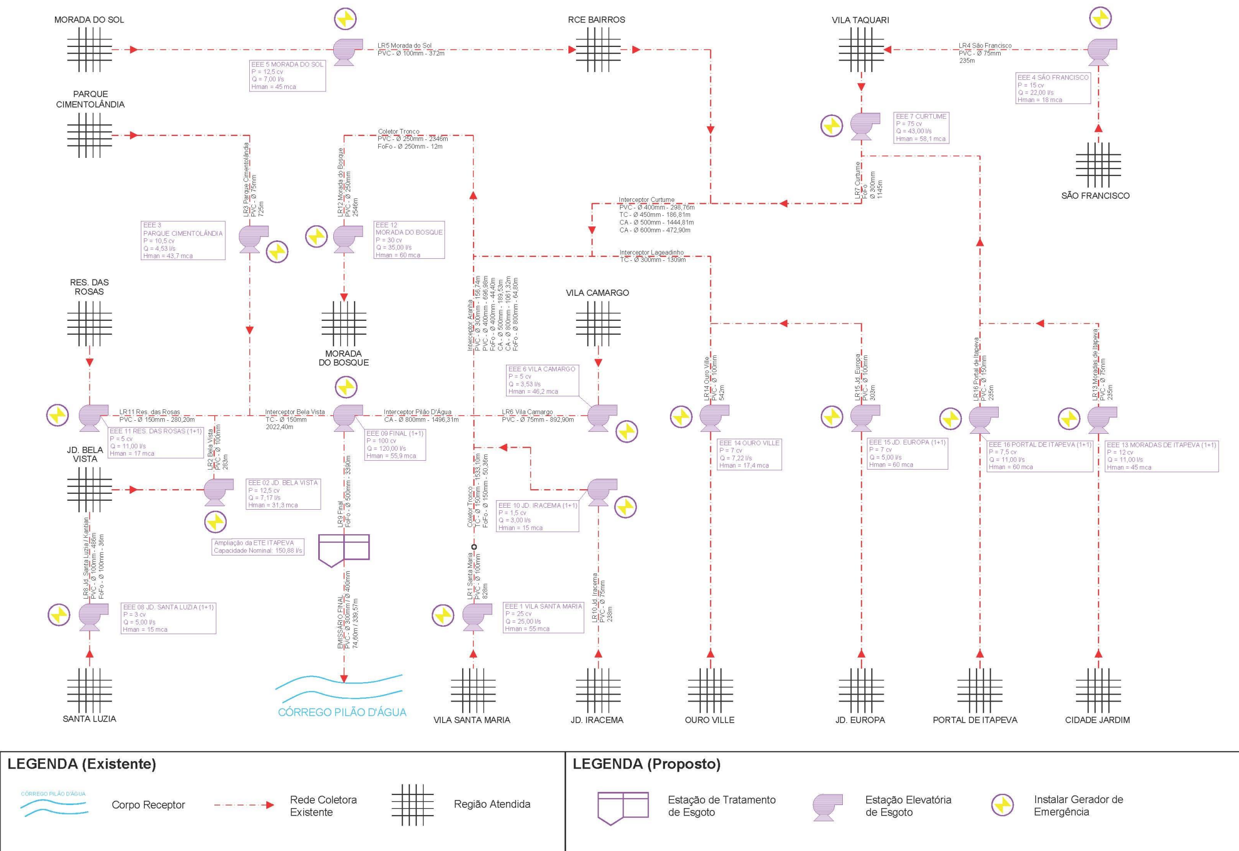
Figura 10.5 – Croqui do Sistema de Esgotamento Sanitário Proposto para Sede Urbana
