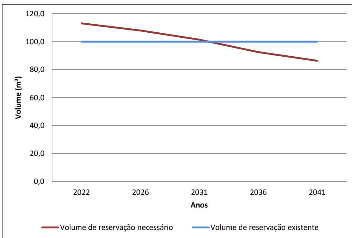
Gráfico 8.7 - Volume de Reservação Necessário (m³) x Volume de Reservação Atual (m³)
