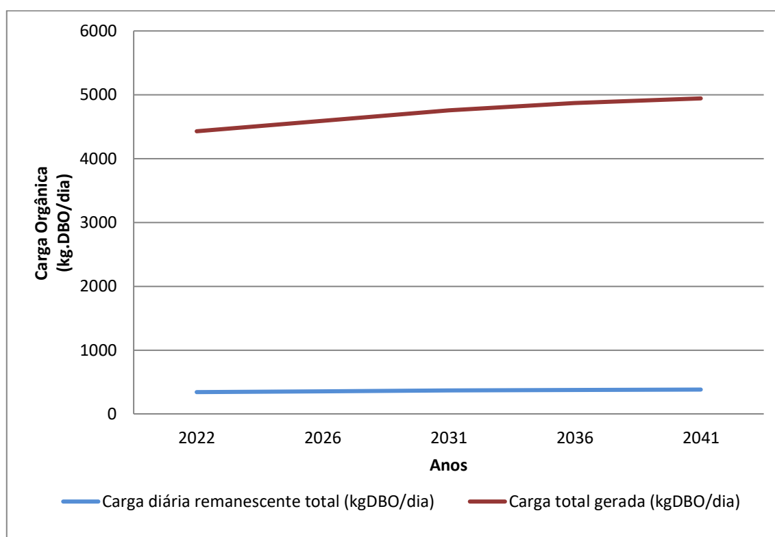
Gráfico 8.9 - Evolução de Cargas Orgânicas (Kg DBO/Dia)
