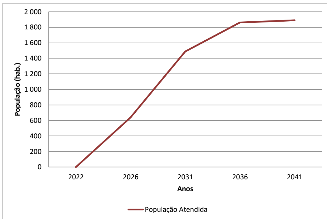
Gráfico 7.10- População Atendida (hab.) x Anos de Planejamento – Distrito de Alto da Brancal
