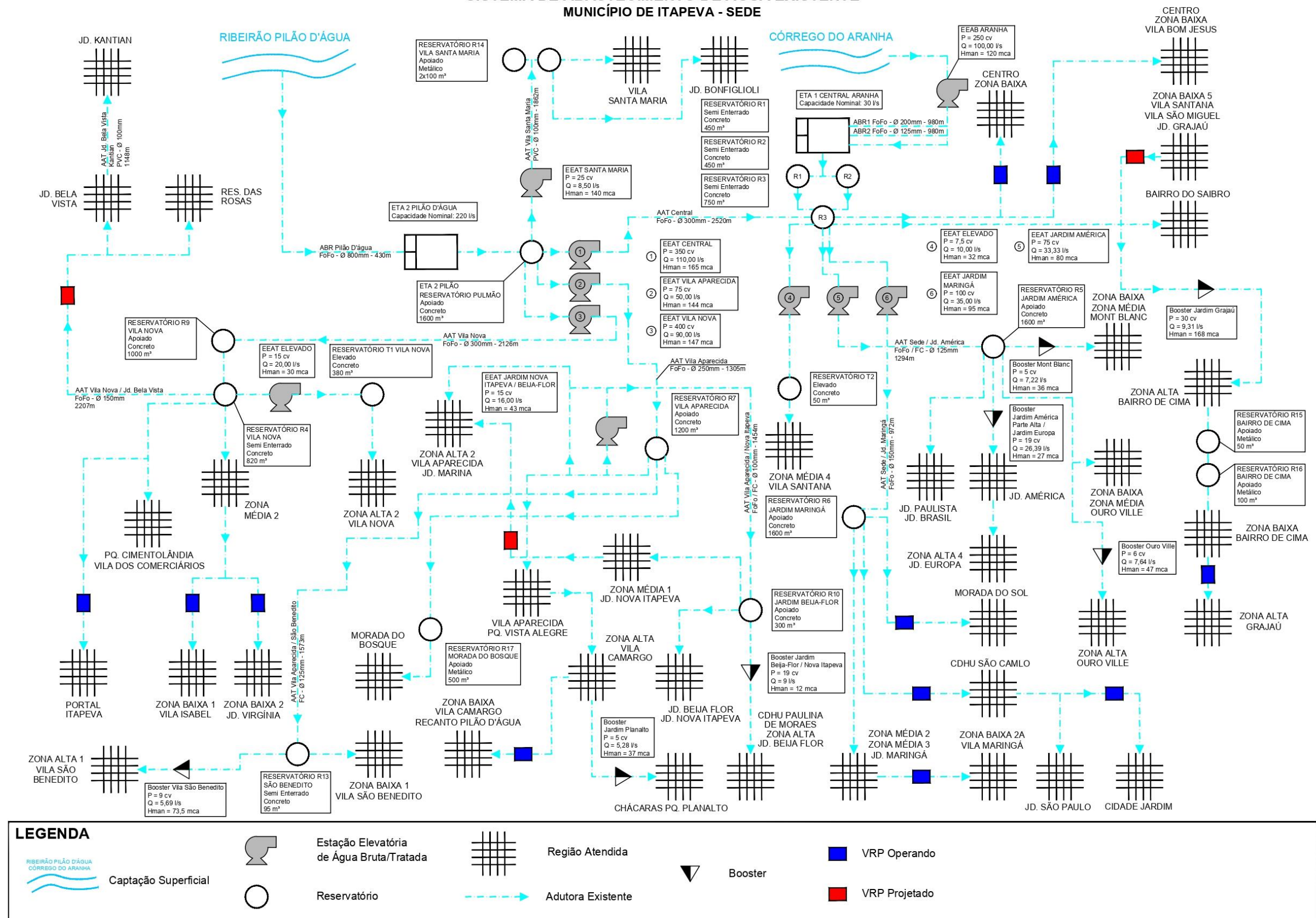
Figura 4.1 – Croqui do Sistema de Abastecimento de Água Existente – Sede Urbana.
