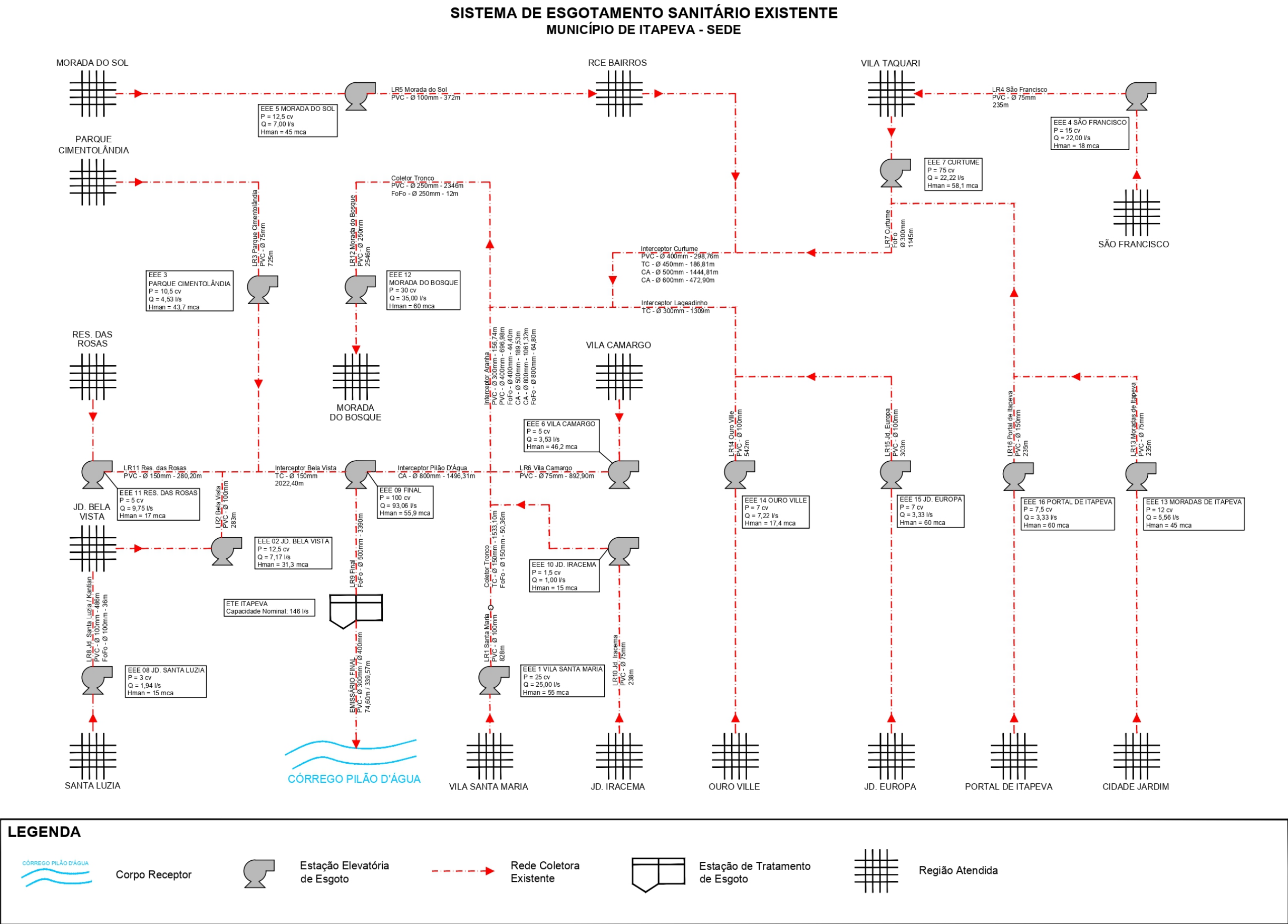
Figura 4.7– Croqui do Sistema de Esgotamento Sanitário Existente – Sede Urbana Fonte: SABESP, 2020.
