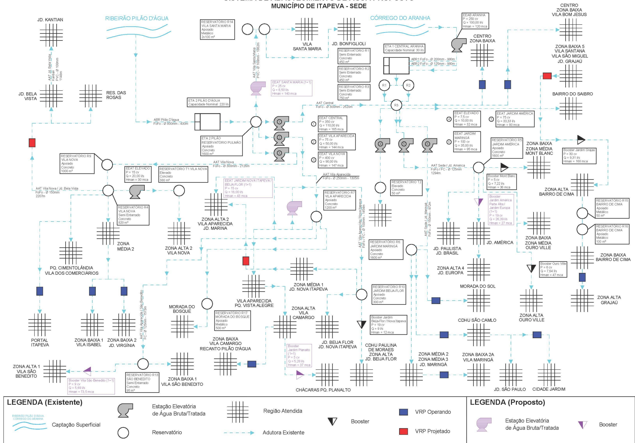
Figura 10.1 – Croqui do Sistema de Abastecimento de Água Proposto para a Sede Urbana
