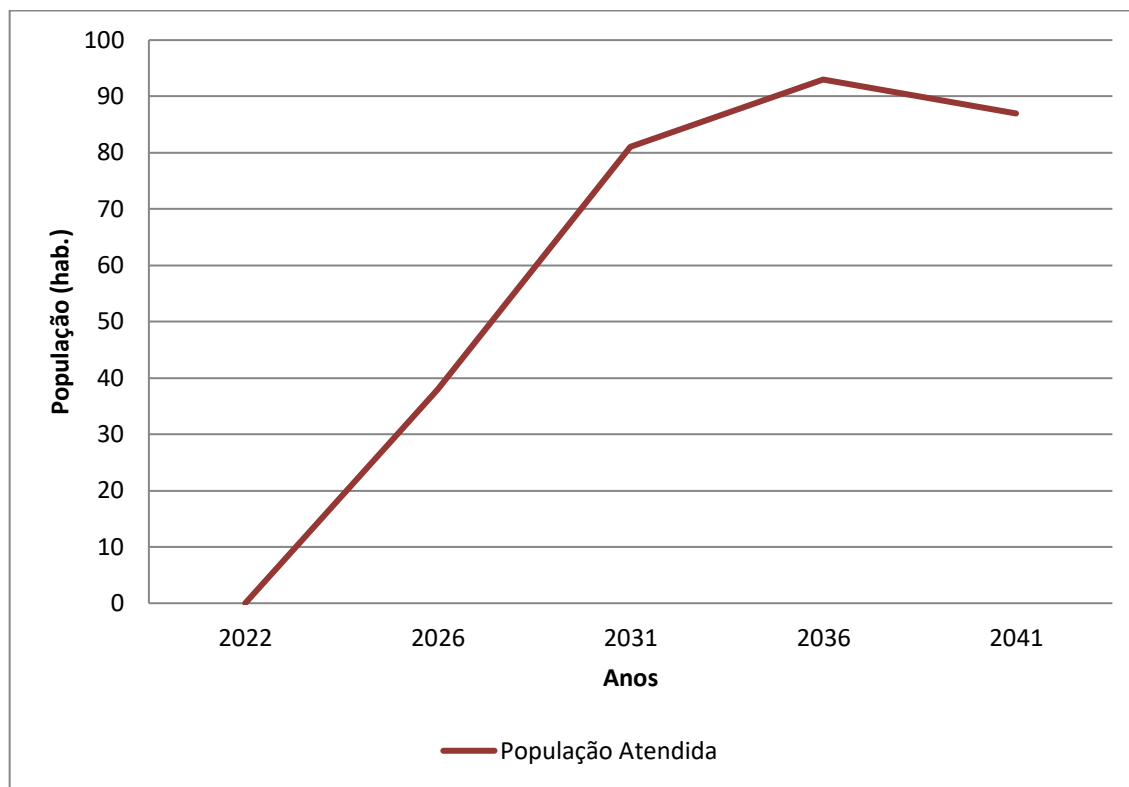
Gráfico 7.10 - População Atendida (hab.) x Anos de Planejamento – Bairro São Sebastião
