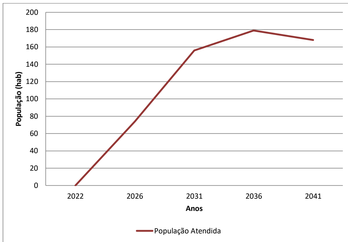
Gráfico 7.12 - População Atendida (hab.) x Anos de Planejamento – Bairro Cruzeiroinho
