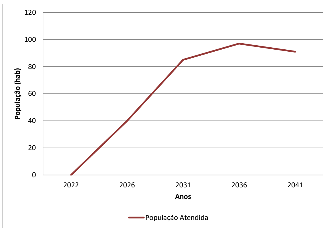
Gráfico 7.13 - População Atendida (hab.) x Anos de Planejamento – Bairro da Onça
