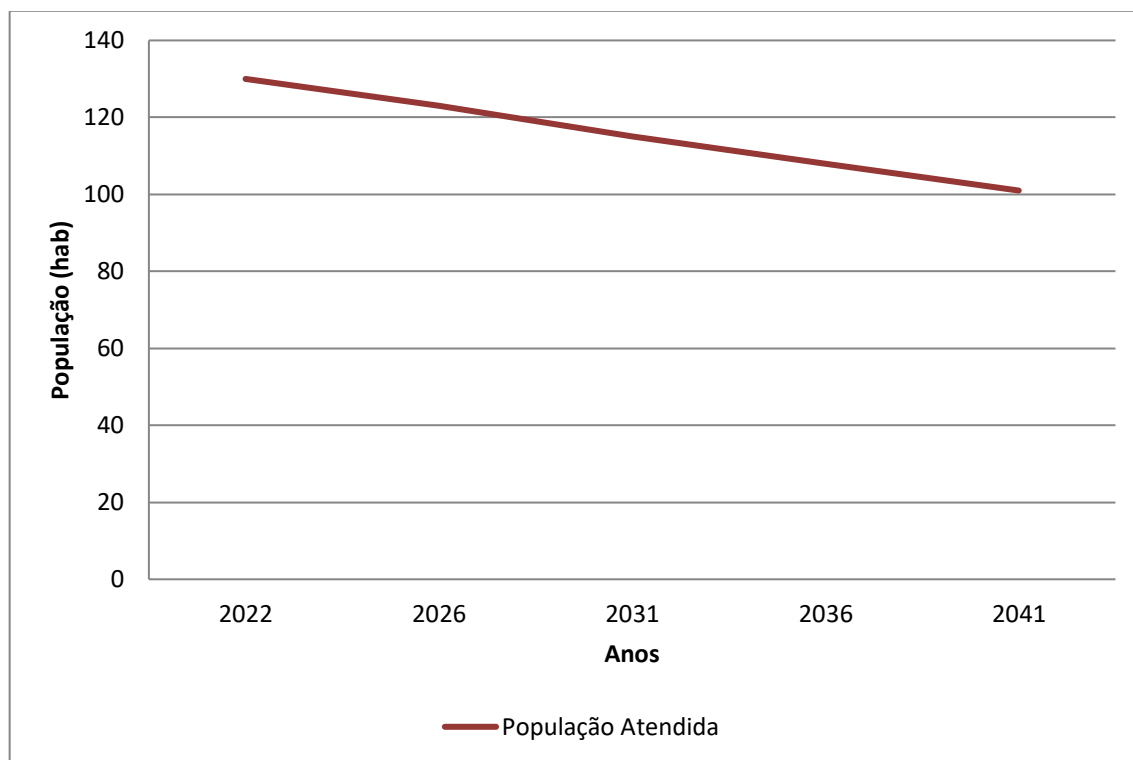
Gráfico 7.7 – População Atendida (hab.) x Anos de Planejamento – Bairro da Onça
