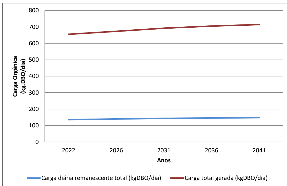
Gráfico 8.10 - Evolução de Cargas Orgânicas (Kg DBO/Dia)
