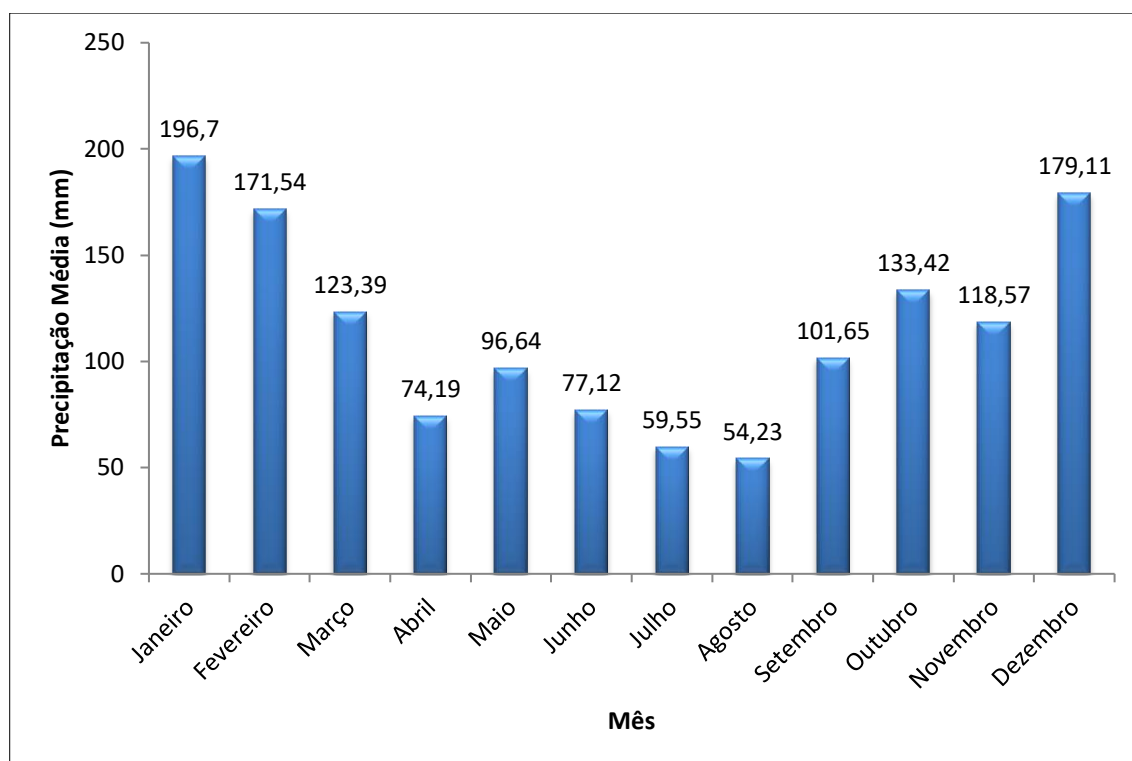
Gráfico 3.1 – Precipitação Média Mensal no Período de 1959 a 2006, Estação E6-008
