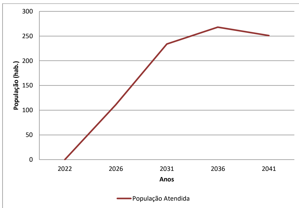
Gráfico 7.11 - População Atendida (hab.) x Anos de Planejamento – Bairro Ribeirão Branco
