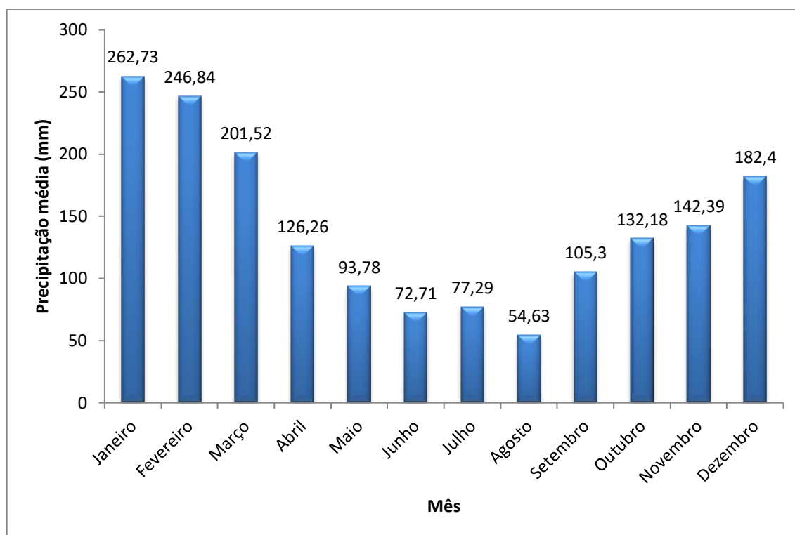
Gráfico 3.1 – Precipitação Média Mensal no Período de 1959 a 2021, Estação F4-006
