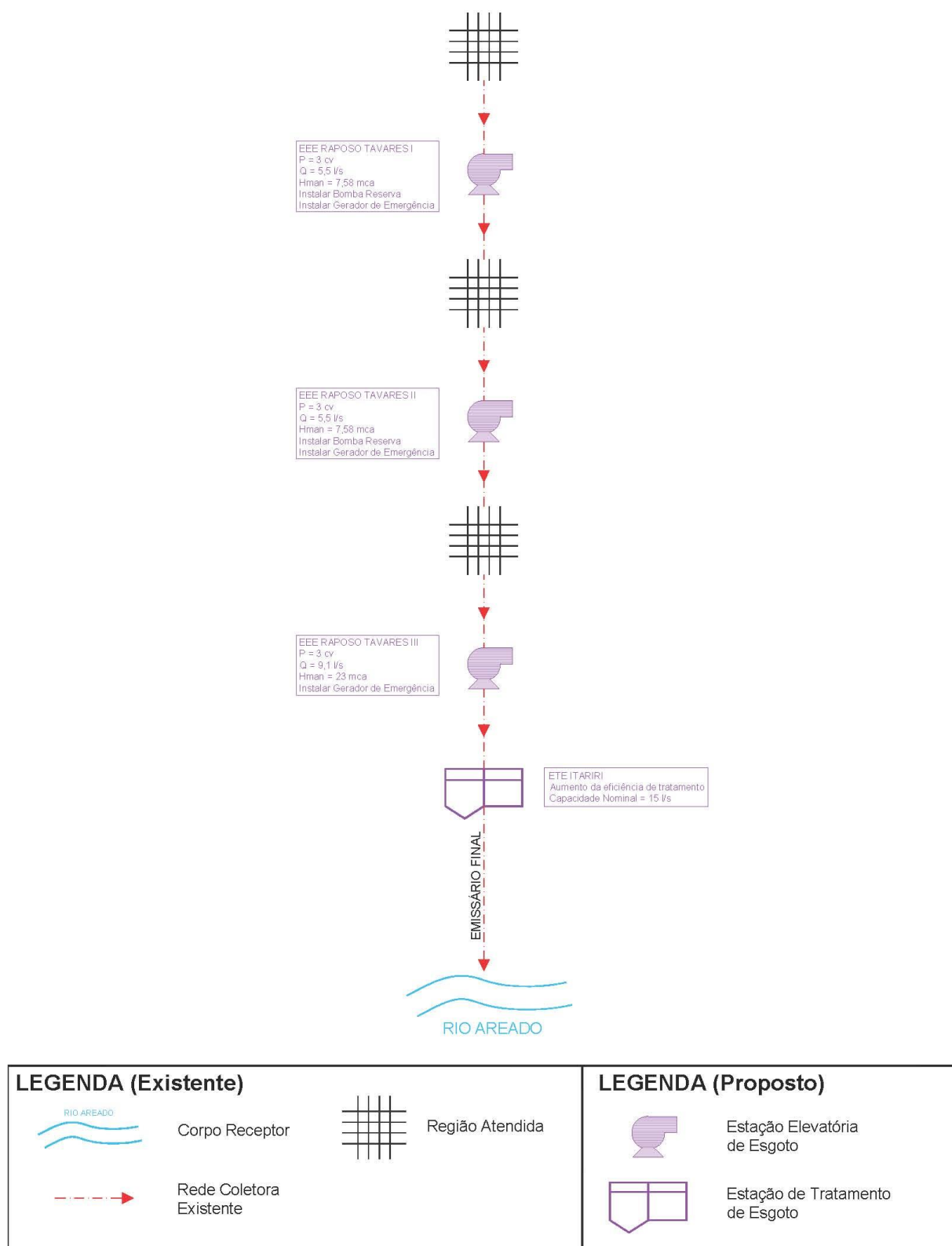
Figura 10.7 – Croqui do Sistema de Esgotamento Sanitário Proposto para o Substema do Bairro Raposo Tavares
