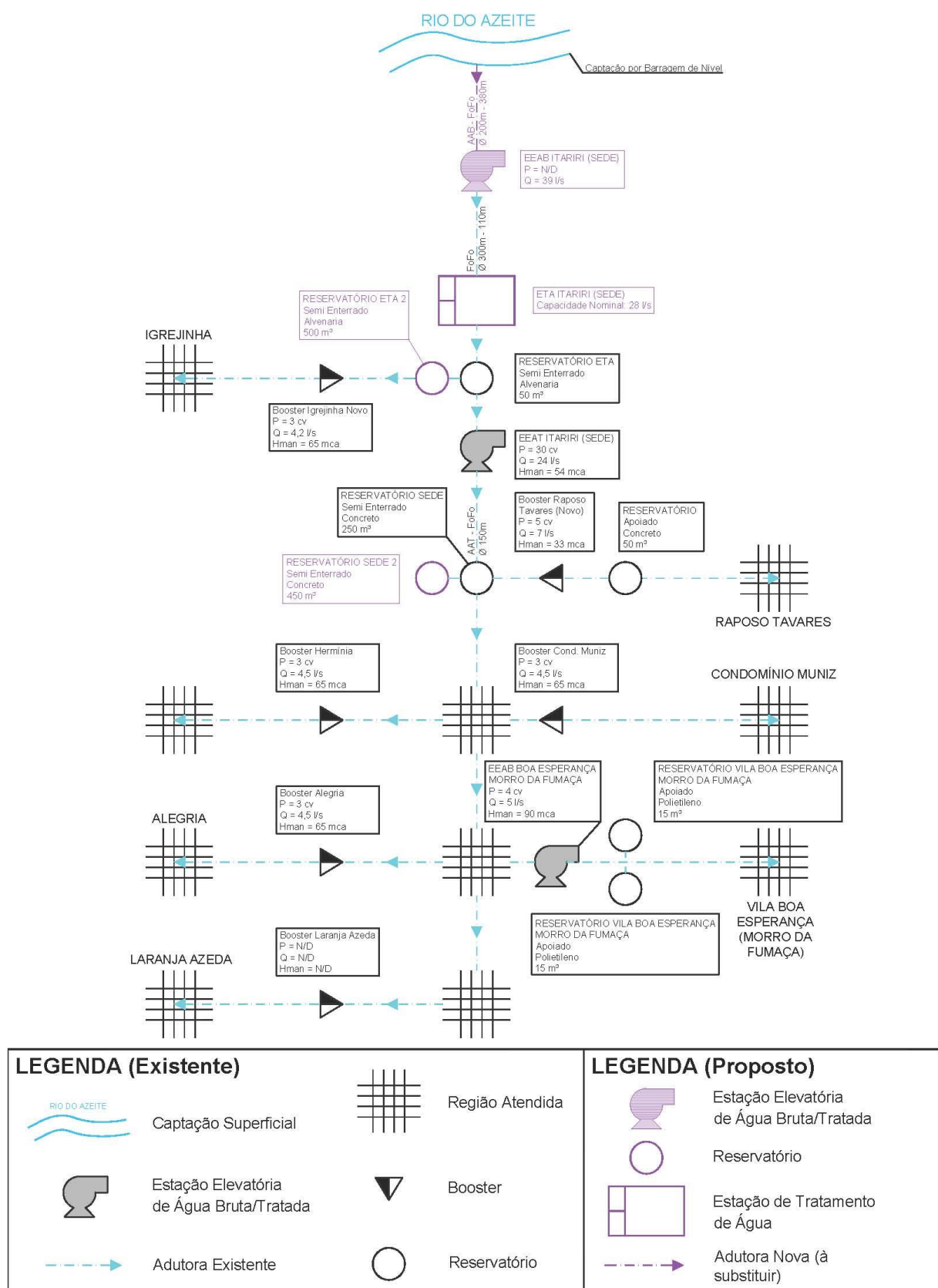
Figura 10.1 – Croqui do Sistema de Abastecimento de Água Proposto para o Sistema Sede Urbana + Bairro Raposo Tavares
