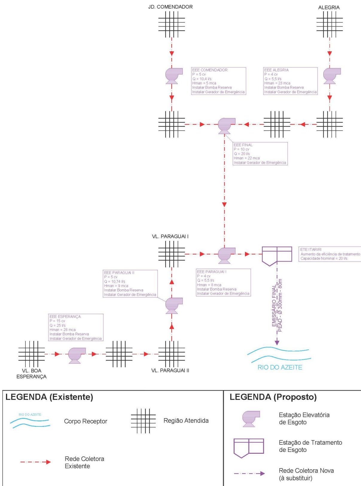
Figura 10.4 – Croqui do Sistema de Esgotamento Sanitário Proposto para o Sistema Sede Urbana
