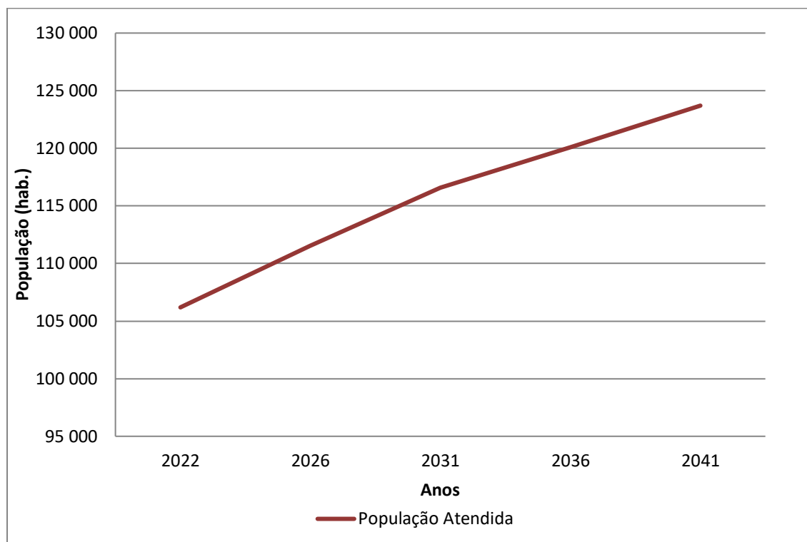
Gráfico 7.2 – População Atendida (hab.) x Anos de Planejamento – Sede Urbana + Bairro Residencial Villagio Paradiso
