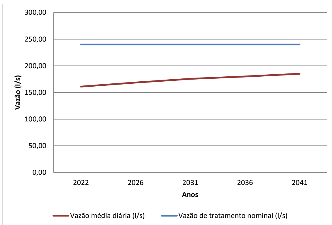
Gráfico 8.5 – Contribuição Média Diária (l/s) x Capacidade nominal da ETE (l/s)
