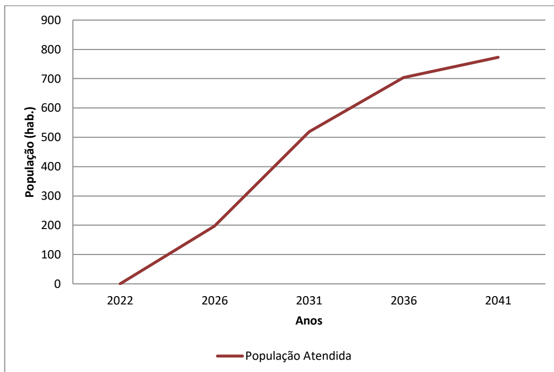
Gráfico 7.7 - População Atendida (hab.) x Anos de Planejamento – Bairro San Martin
