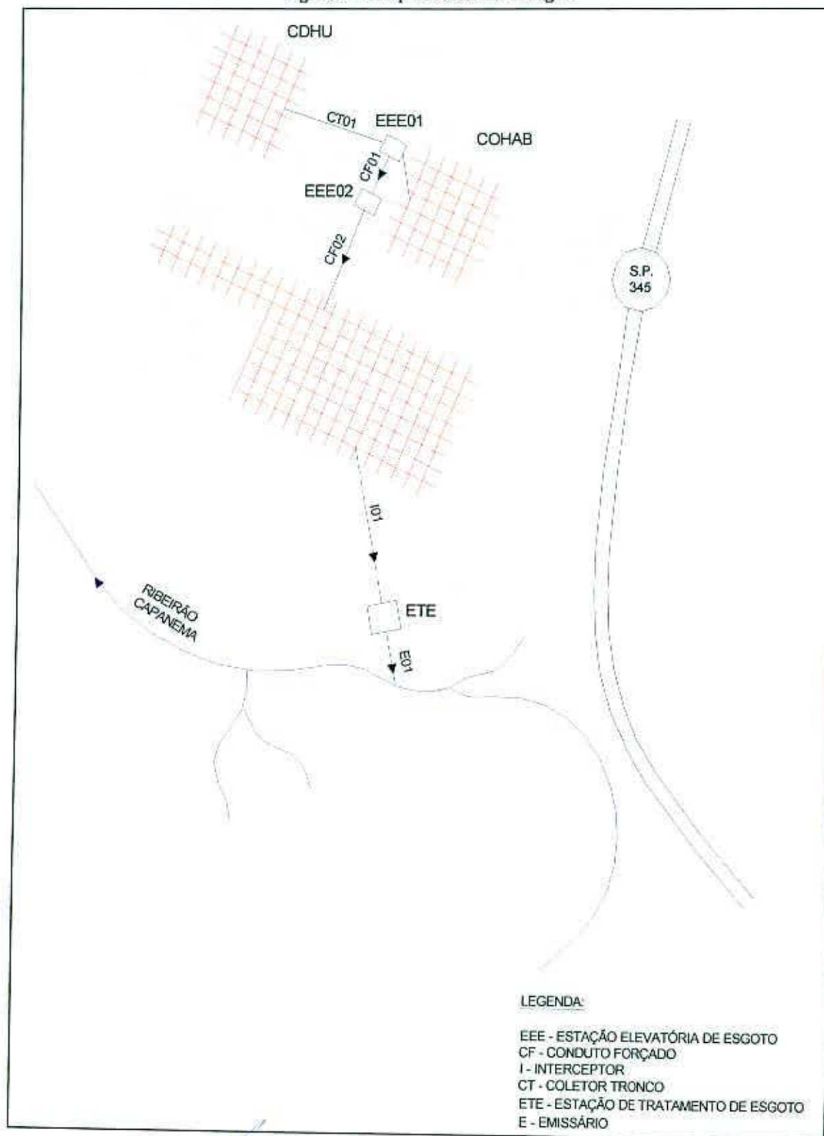
Figura 5 - Croqui do sistema de esgoto
