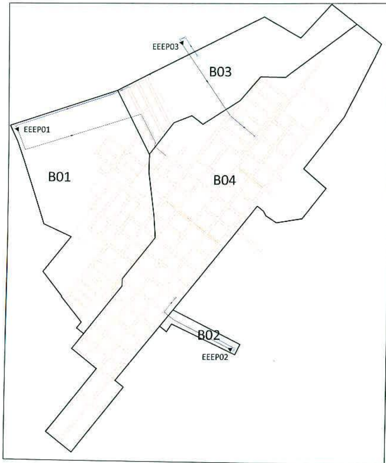
Figura 15 - Melhor alternativa para o sistema de afastamento de esgoto de fim de plano
