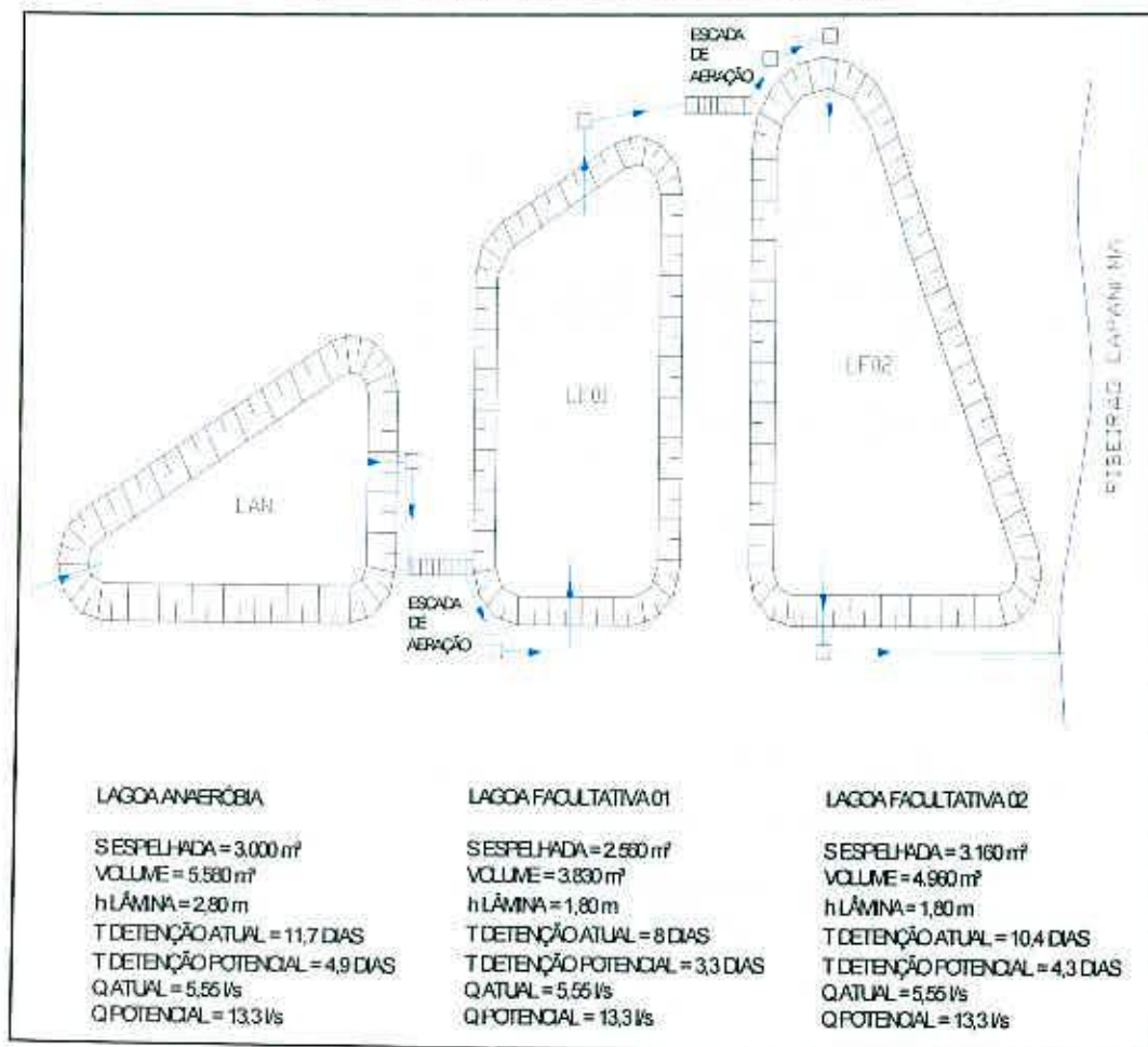
Figura 6 - Sistema de tratamento de esgoto - ETE
