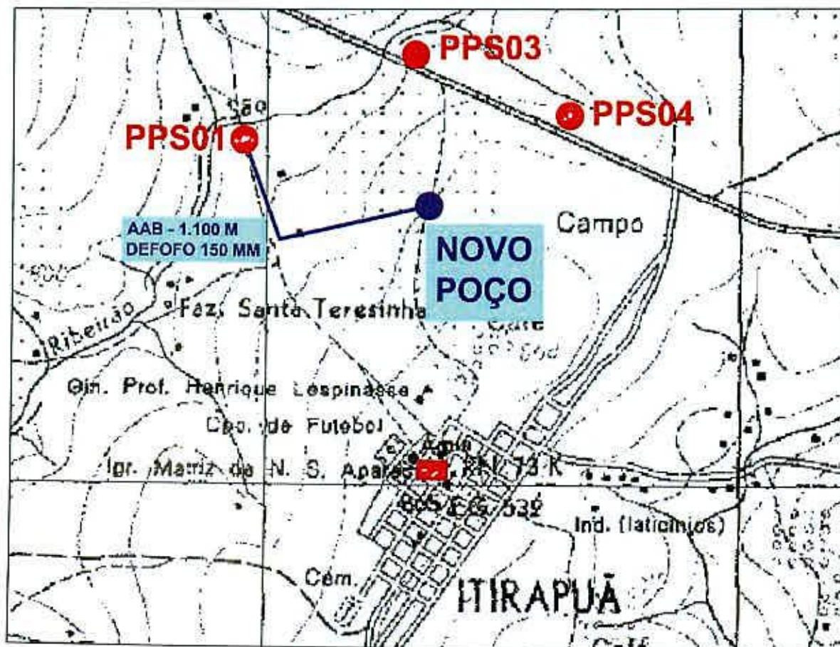
Figura 11 - AAB do novo poço
