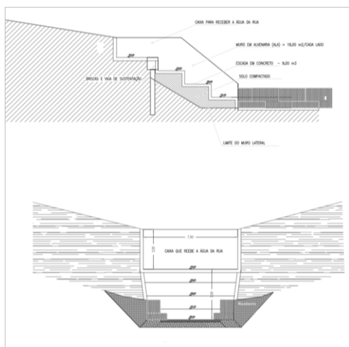
Foto 3.54 – Cortes do projeto do Canal – Rua 26 de Dezembro
