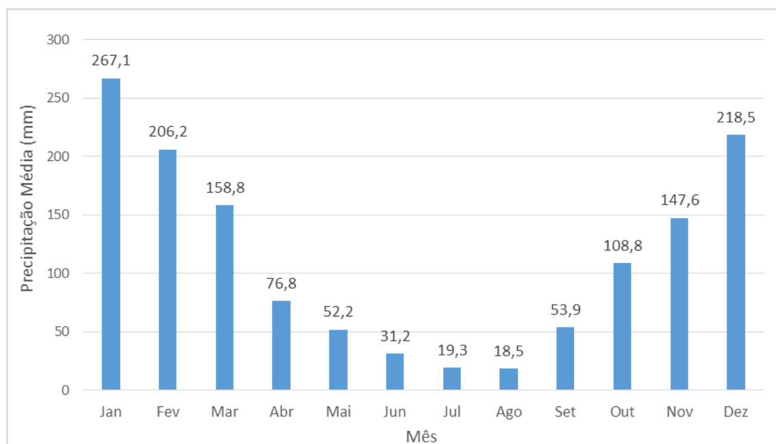
Gráfico 2.1 - Precipitação Média Mensal no Período de 1937 a 2016, Estação B6-002
