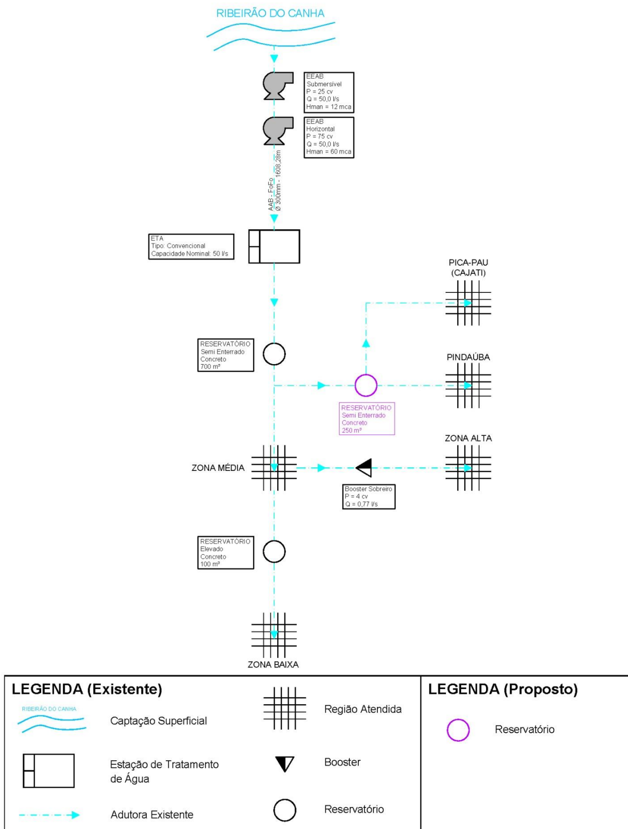
Figura 10.1 – Croqui do Sistema de Abastecimento de Água Proposto para o Sistema Sede Urbana + Bairro Pindaúba
