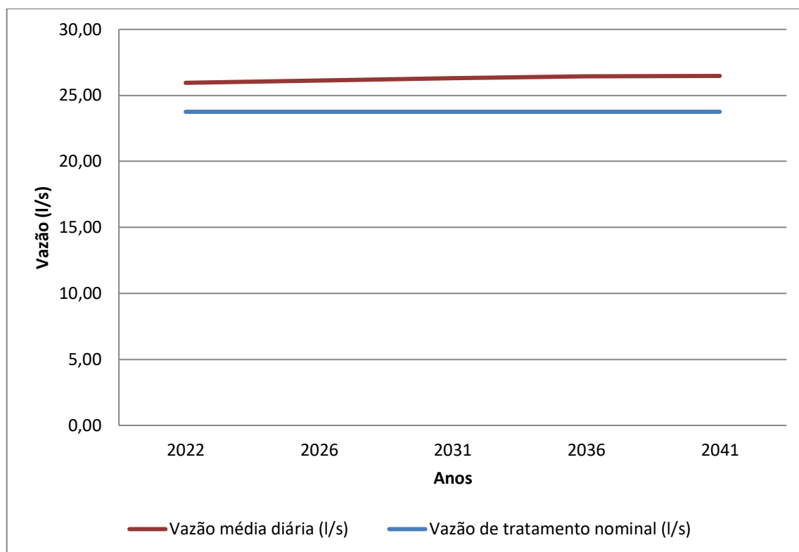
Gráfico 8.3 – Vazão Média Diária (l/s) x Capacidade nominal da ETE (l/s)
