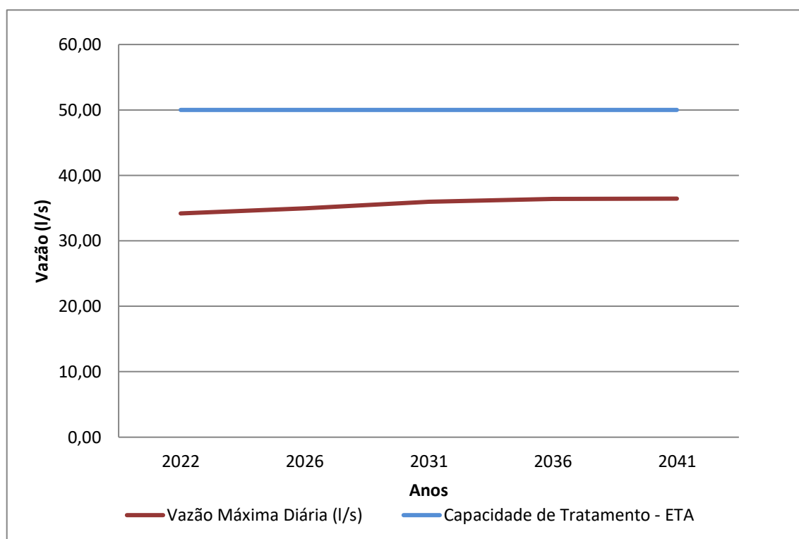
Gráfico 8.1 – Vazão Máxima Diária (l/s) X Capacidade de Tratamento ETA (l/s)
