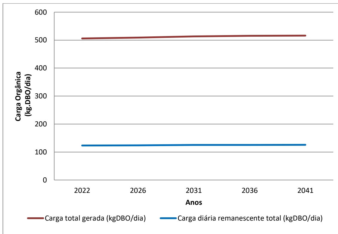
Gráfico 8.4 - Evolução de Cargas Orgânicas (Kg DBO/Dia)
