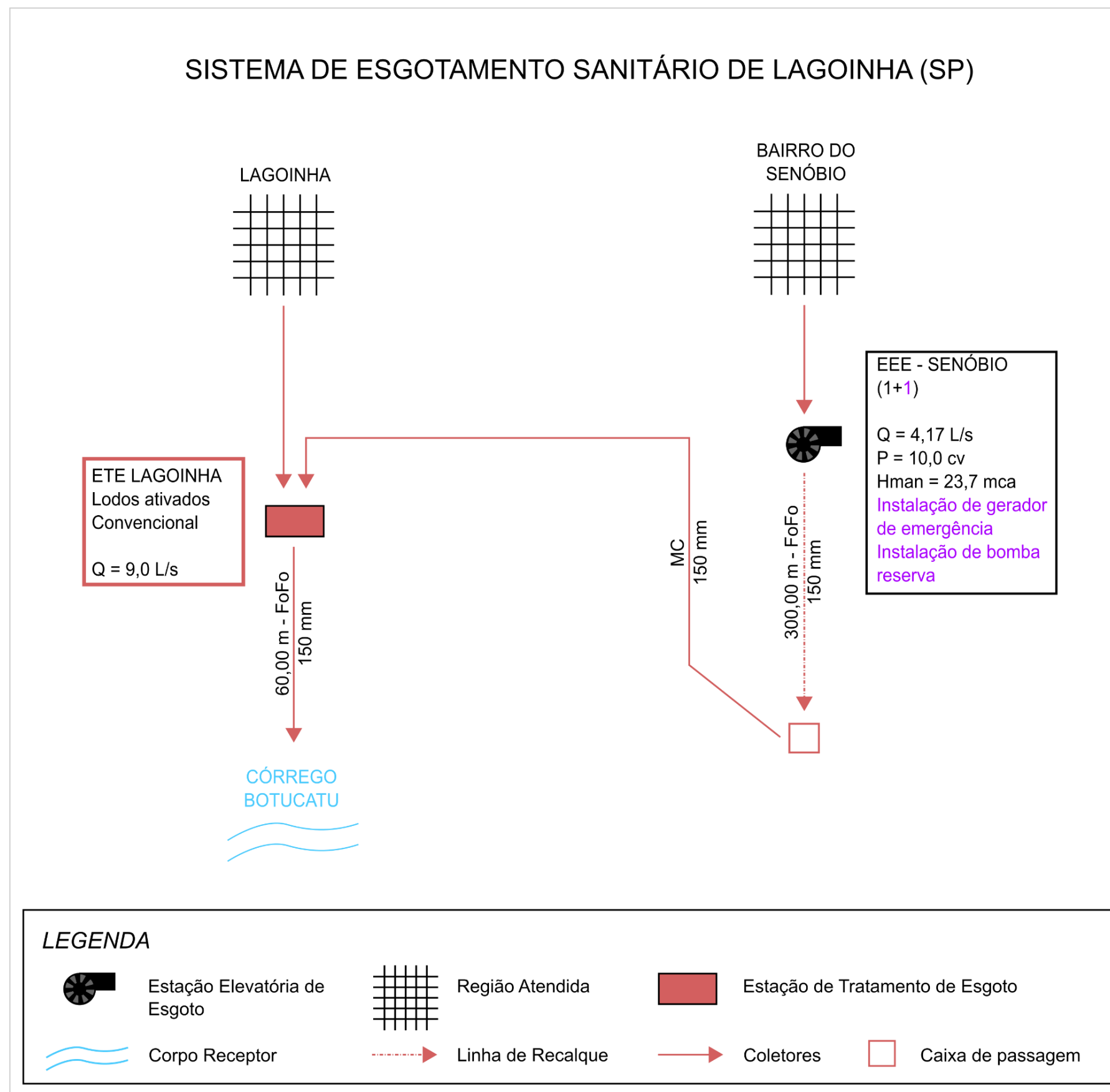
Figura 10.1 – Croqui com as intervenções propostas para o sistema de esgotamento sanitário Sede
