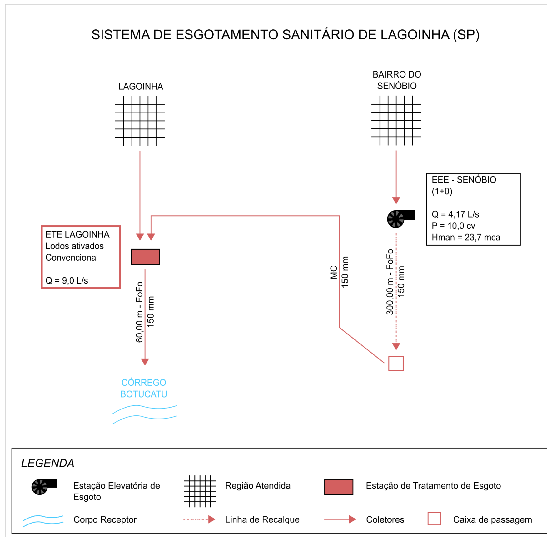
Figura 4.2 – Croqui do Sistema de Esgotamento Sanitário da Sede de Lagoinha.
