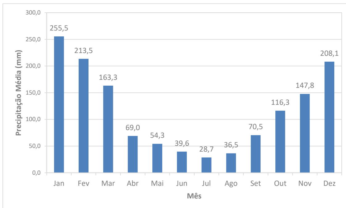
Figura 3.2 - Precipitação Média Mensal no Período de 1959 a 2006, Estação E2-007
