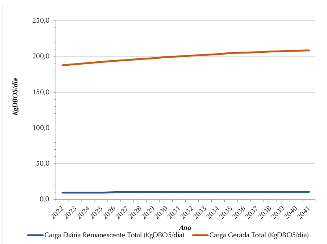
Figura 8.4 - Evolução de Cargas Orgânicas (Kg \text{DBO}_{5,20} /Dia)
