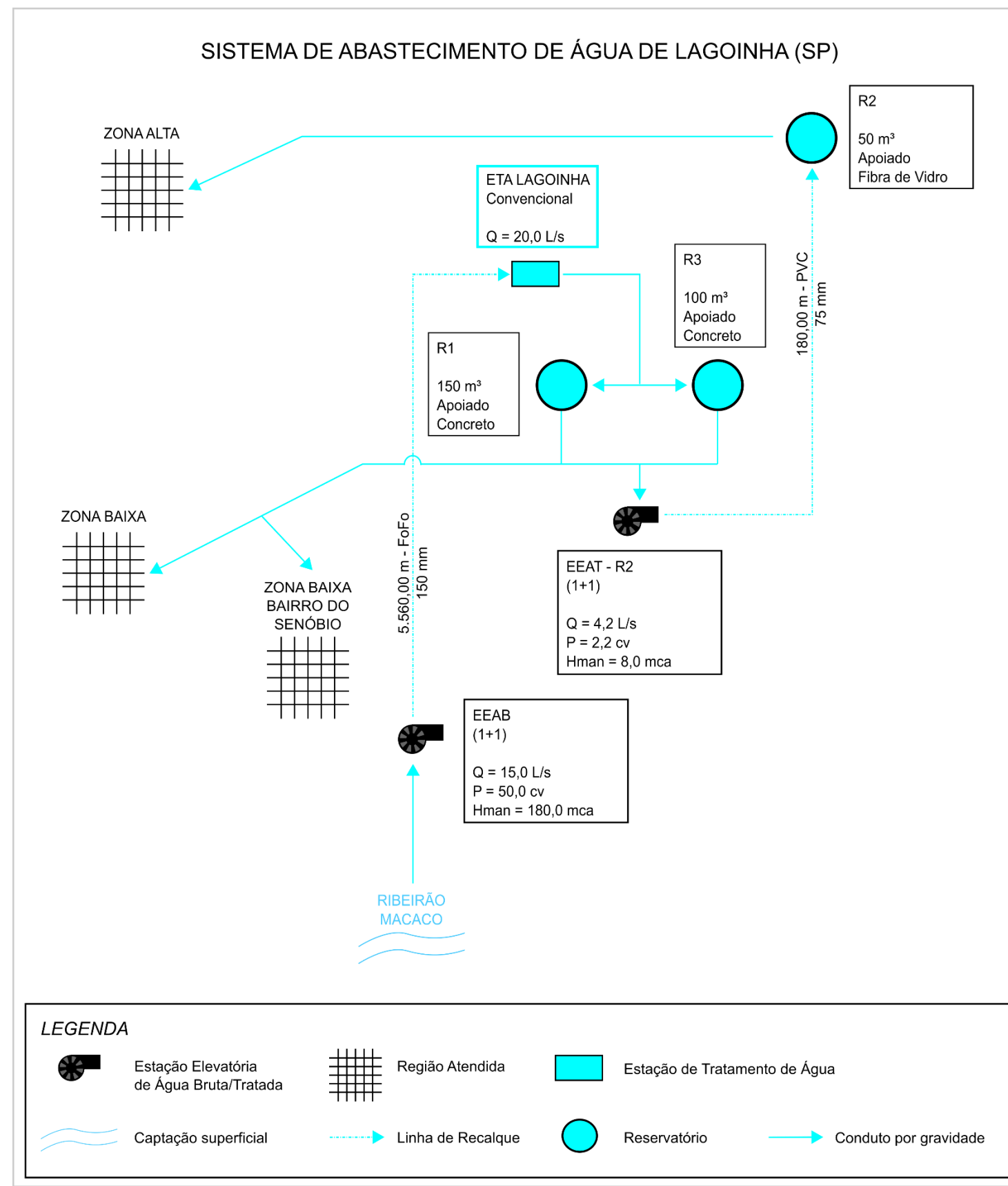
Figura 4.1 – Croqui do Sistema de Abastecimento de Água de Lagoinha. Fonte: SABESP, 2020.
