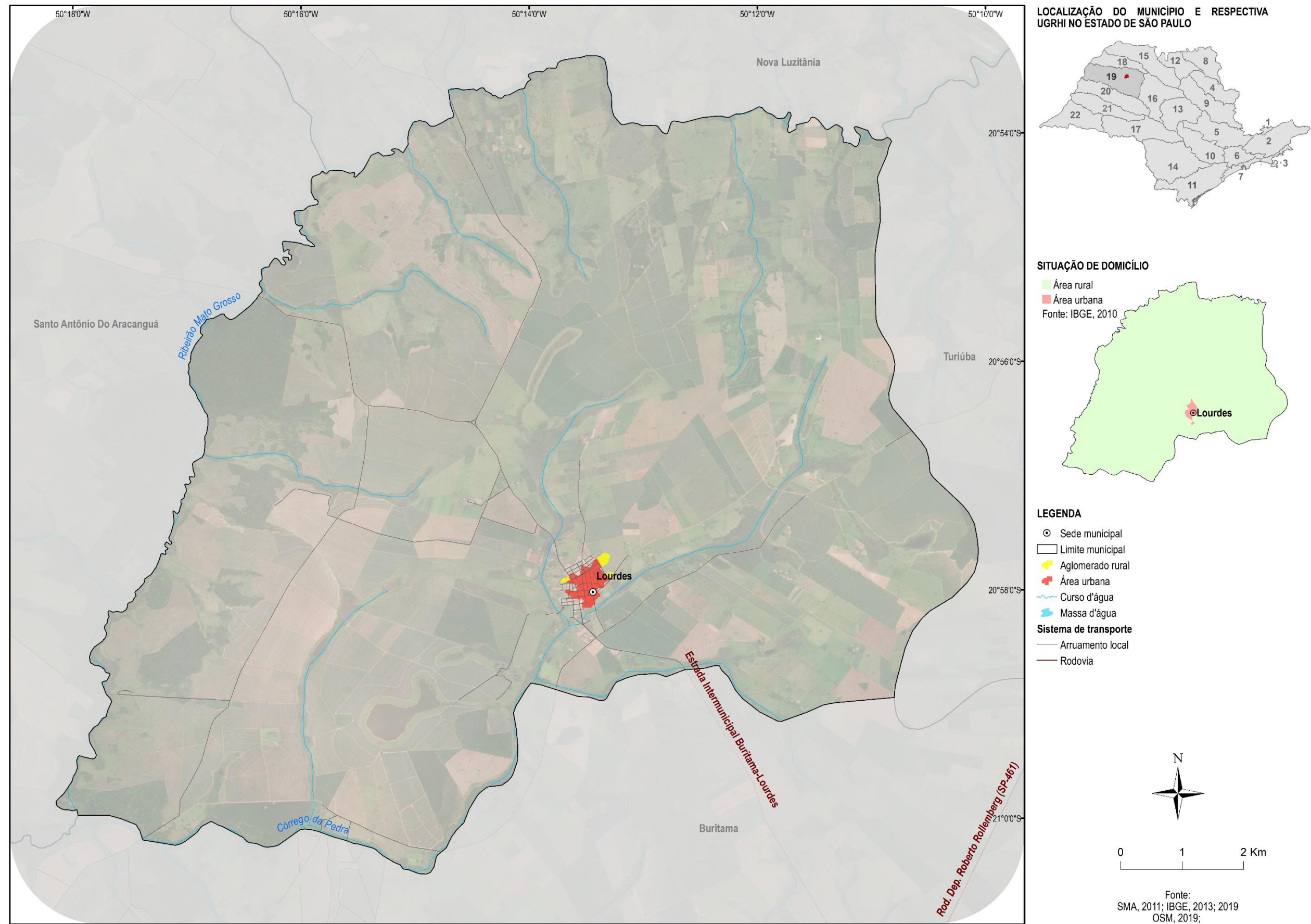
Figura 3.1 – Localização e Acessos do Município de Lourdes
