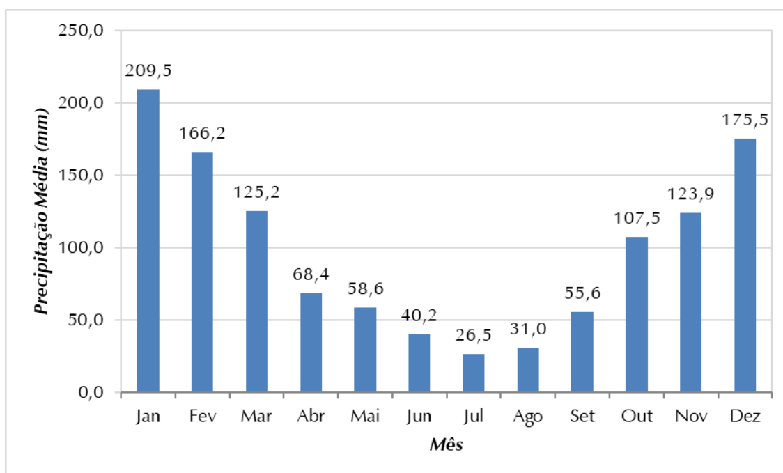
Figura 3.2 - Precipitação Média Mensal no Período de 1946 a 2021, Estação C7-064
