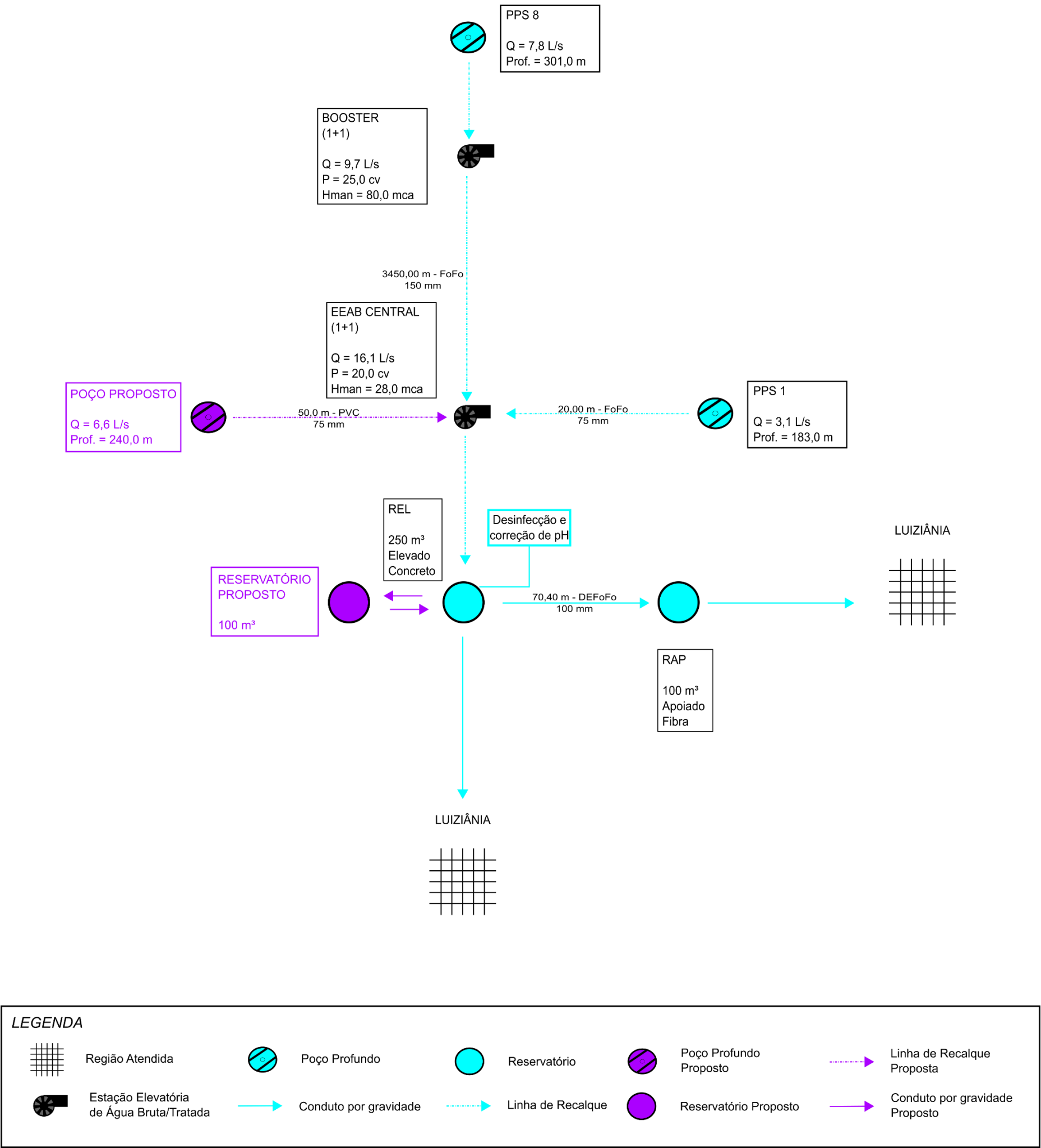
Figura 10.1 – Croqui das intervenções propostas no sistema de abastecimento de água Sede
