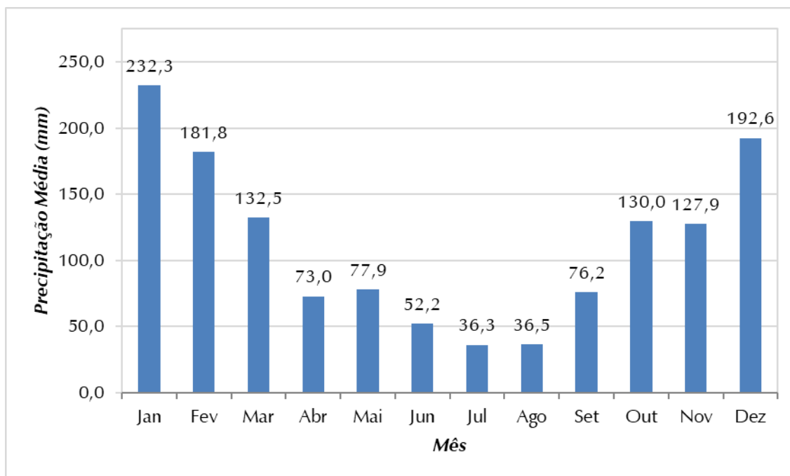
Figura 3.2 - Precipitação Média Mensal no Período de 1961 a 2021, Estação D7-007
