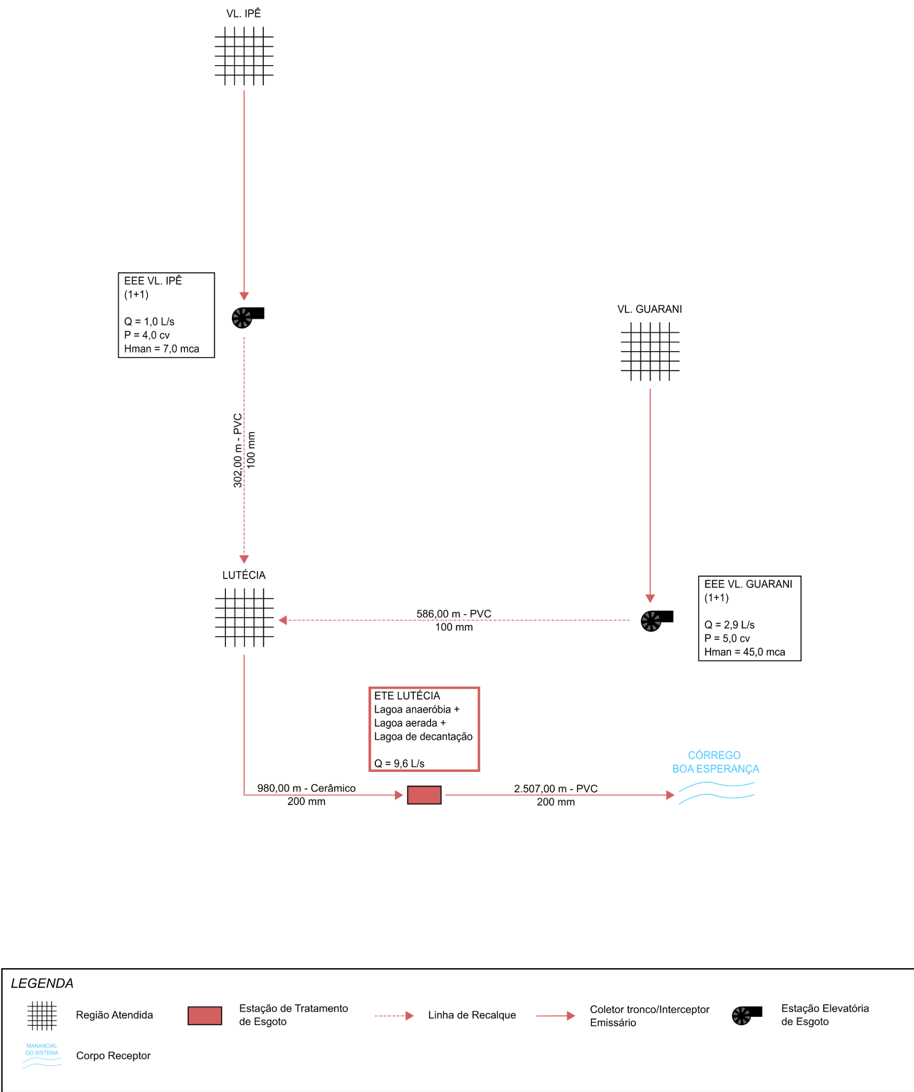
Figura 4.2 – Croqui do Sistema de Esgotamento Sanitário da Sede de Lutécia
