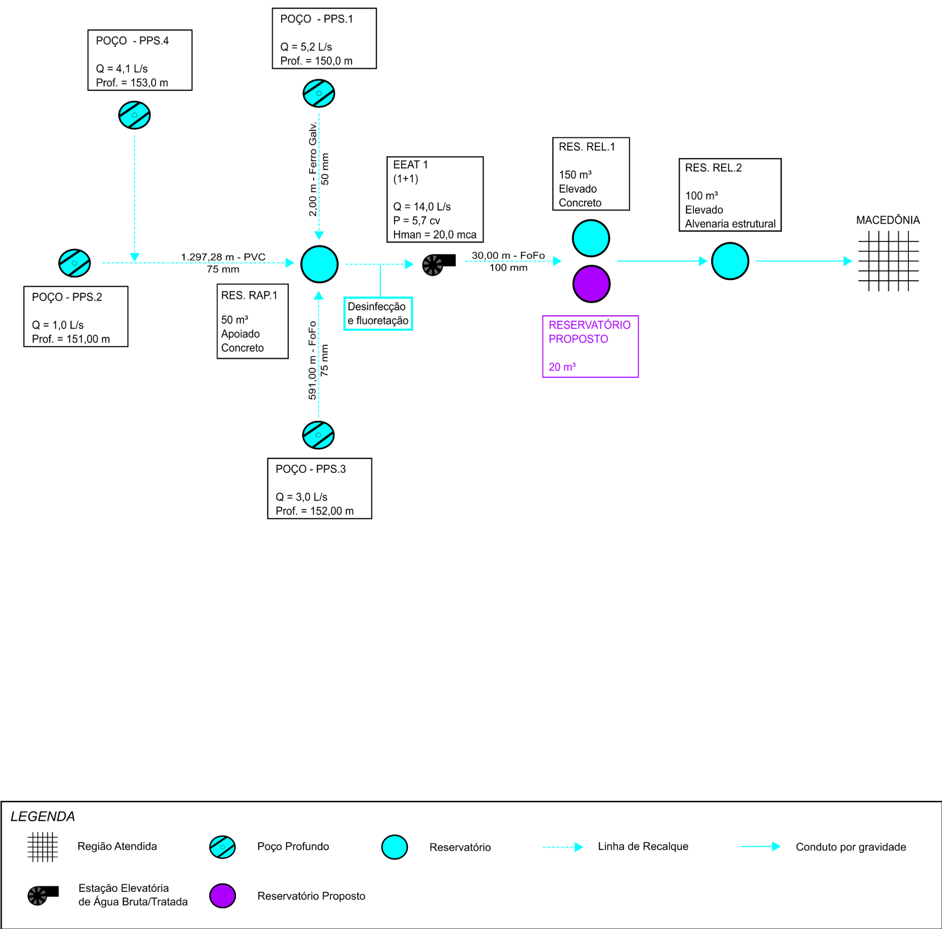
Figura 10.1 – Croqui das intervenções propostas para o sistema de abastecimento de água Sede
